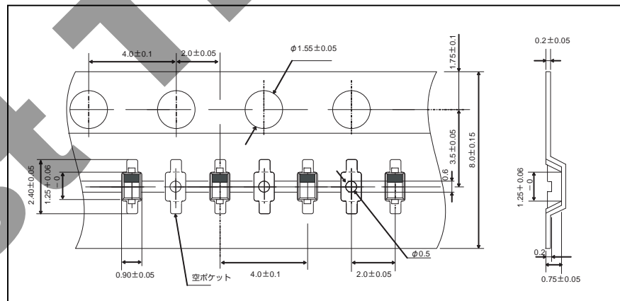
●テーピング仕様 (Unit : mm)
