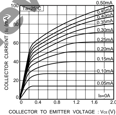
Fig.11 エミッタ接地出力静特性 (I)
