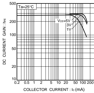
Fig.13 直流電流増幅率 - コレクタ電流特性 (I)
