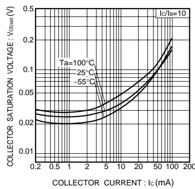
Fig.16 コレクタ・エミッタ間飽和電圧 - コレクタ電流特性 (I)
