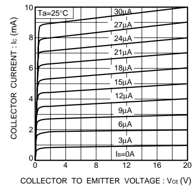
Fig.12 エミッタ接地出力静特性 (II)
