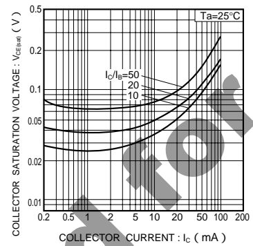
Fig.15 コレクタ・エミッタ間飽和電圧 - コレクタ電流特性
