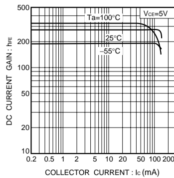
Fig.14 直流電流増幅率 - コレクタ電流特性 (II)
