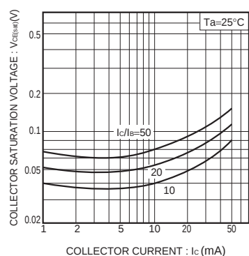
Fig.4 コレクタ・エミッタ飽和電圧 -コレクタ電流特性 (I)
