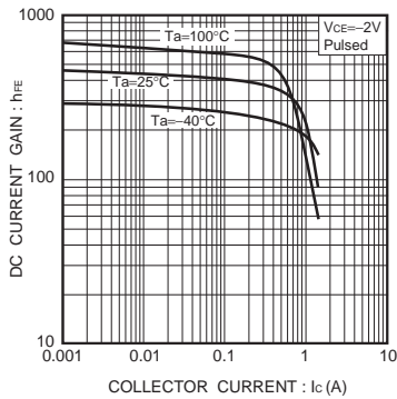
Fig.1 直流電流増幅率 - コレクタ電流特性
