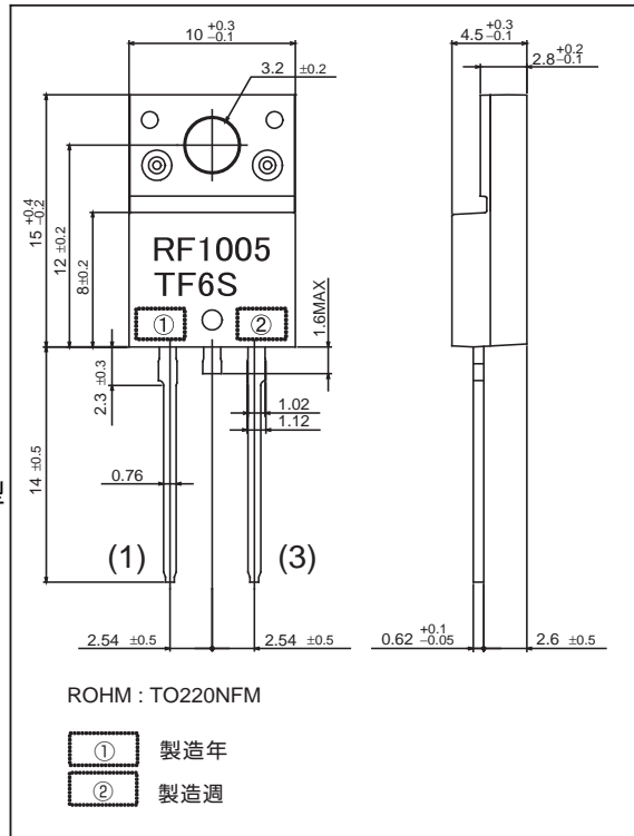
●外形寸法図 (Unit : mm)
