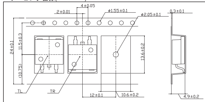
●テーピング仕様(Unit : mm)
