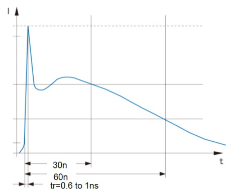
IEC61000-4-2 波形
