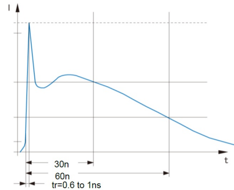
IEC61000-4-2 波形
