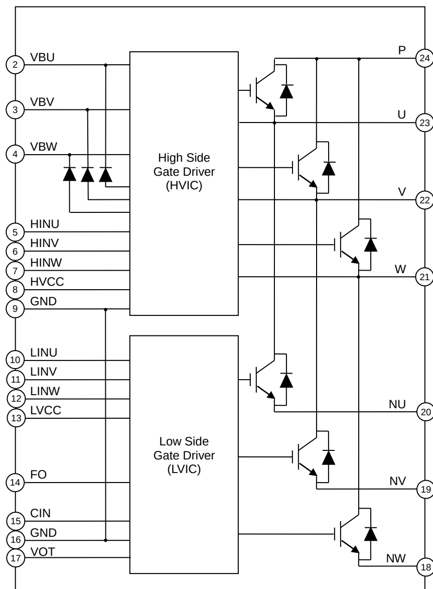
Figure 3. ブロック図
