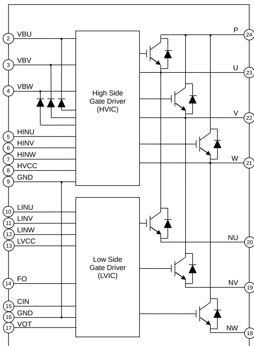
Figure 3. ブロック図
