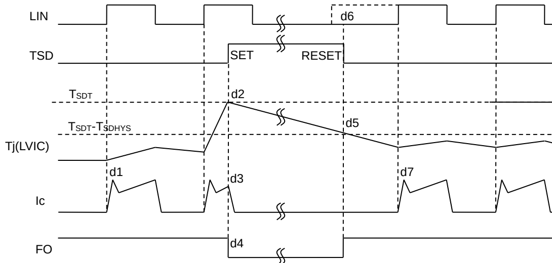
Figure 14. TSD タイミングチャート
