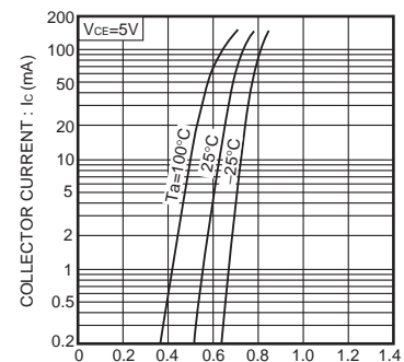
Fig.3 エミッタ接地伝達静特性
