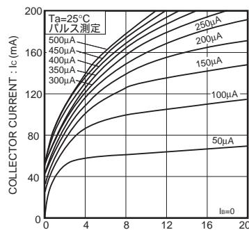
Fig.2 エミッタ接地出力静特性 (II)
