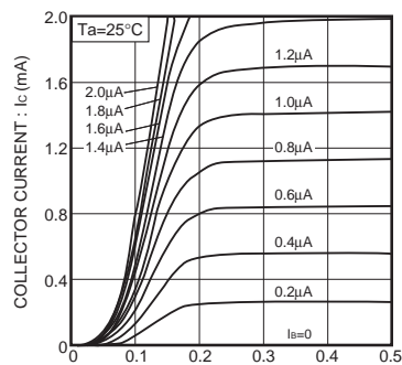
Fig.1 エミッタ接地出力静特性 (I)
