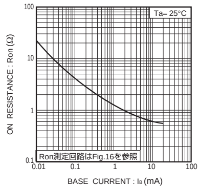
Fig.14 出力オン抵抗 —ベース電流特性 (II)
