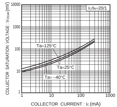
Fig.6 コレクタ・エミッタ間飽和電圧 -コレクタ電流特性 (II)
