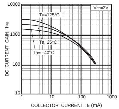
Fig.3 直流電流増幅率 -コレクタ電流特性 (I)
