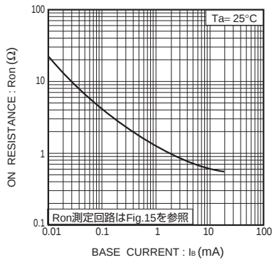
Fig.13 出力オン抵抗 —ベース電流特性 (I)
