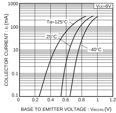
Fig.2 エミッタ接地伝達静特性 (II)
