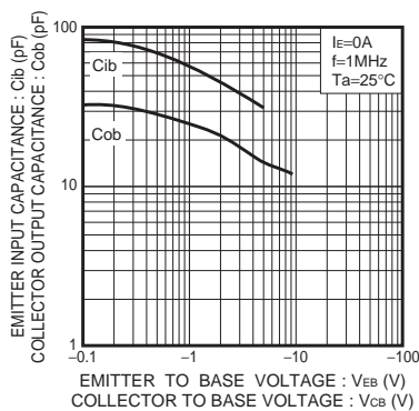
Fig.7 コレクタ出力容量 - コレクタ・ベ - ス間電圧特性 エミッタ入力容量 - エミッタ・ベ - ス間電圧特性
