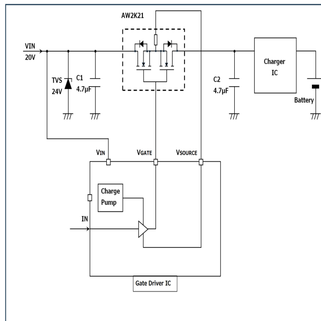
図. 1 USB PD 回路
