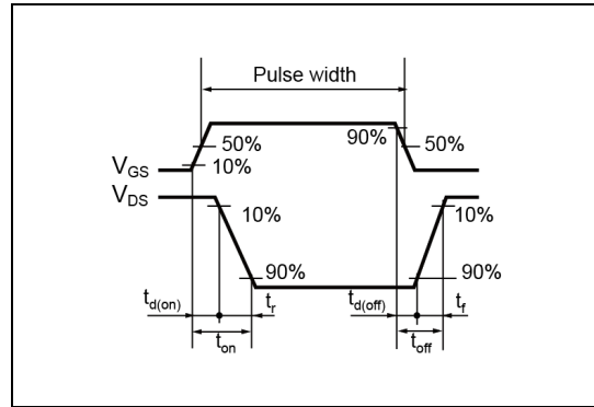
図 1-2 スイッチング波形
