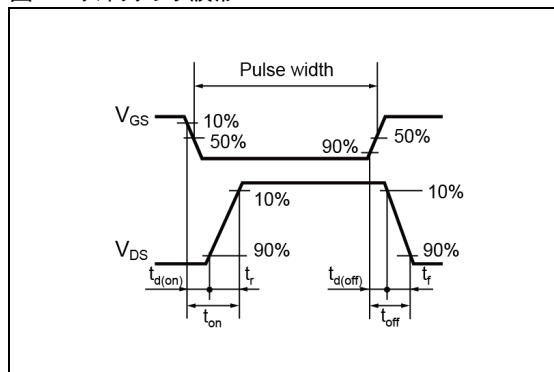
図 2-2 スイッチング波形
