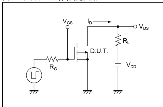
図 2-1 スイッチング時間測定回路
