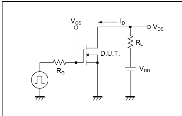
図 1-1 スイッチング時間測定回路
