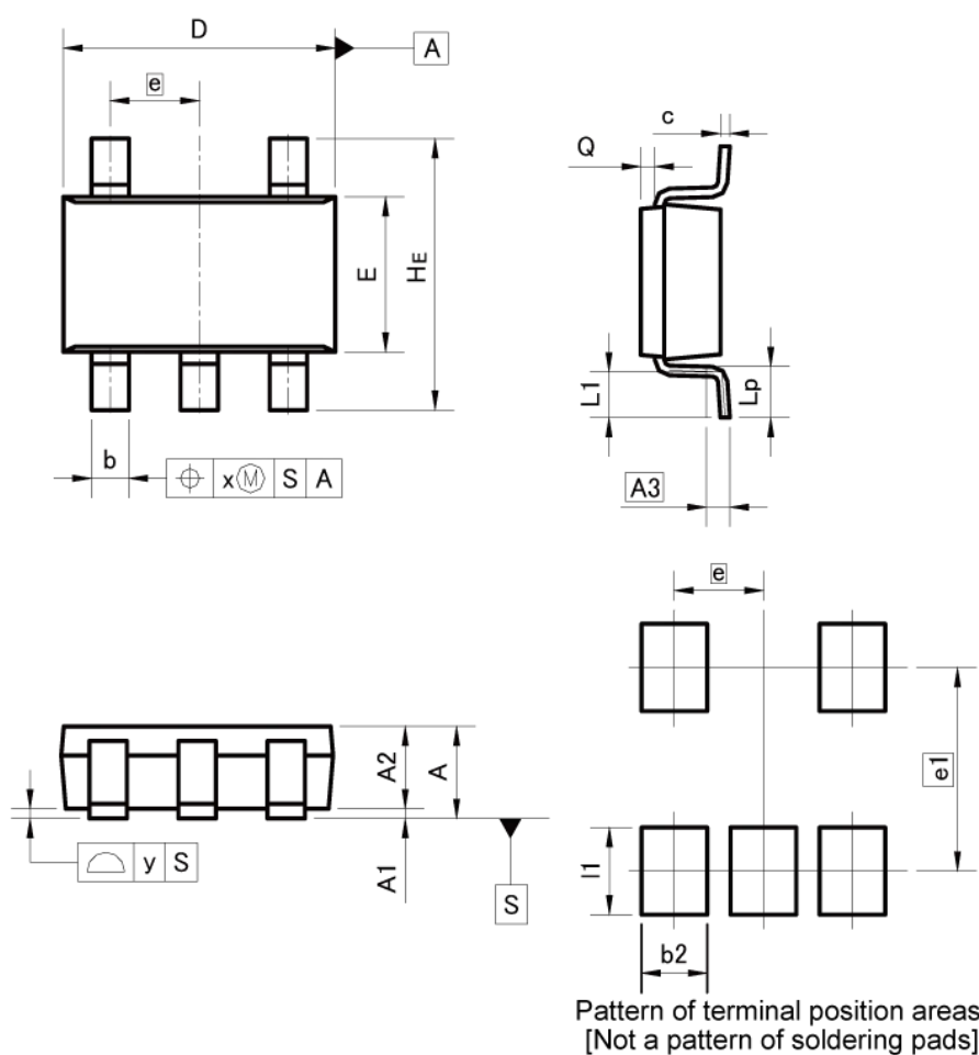
TSM5 < SOT-25T >
