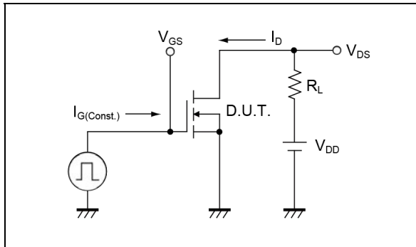
図 3-1 アバランシェ測定回路
