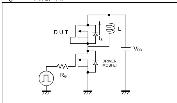
Fig.4-1 trr測定回路
