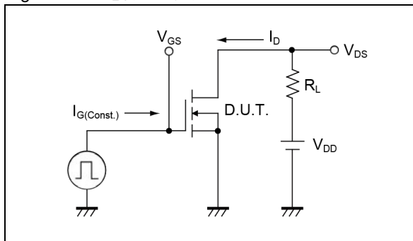
Fig.3-1 アバランシェ測定回路
