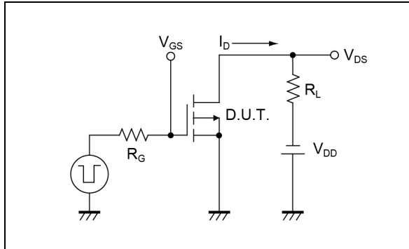
図 1-1 スイッチング時間測定回路
