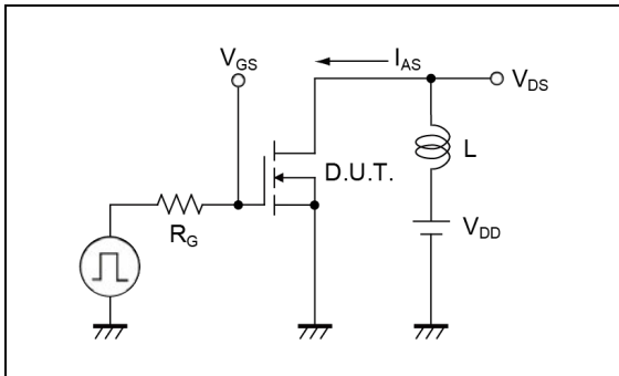
図 3-1 アバランシェ測定回路
