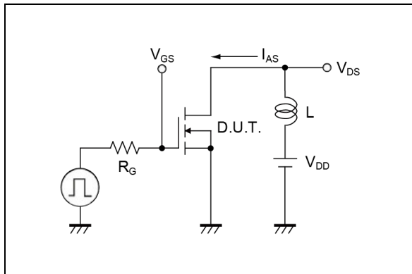
図 3-1 アバランシェ測定回路
