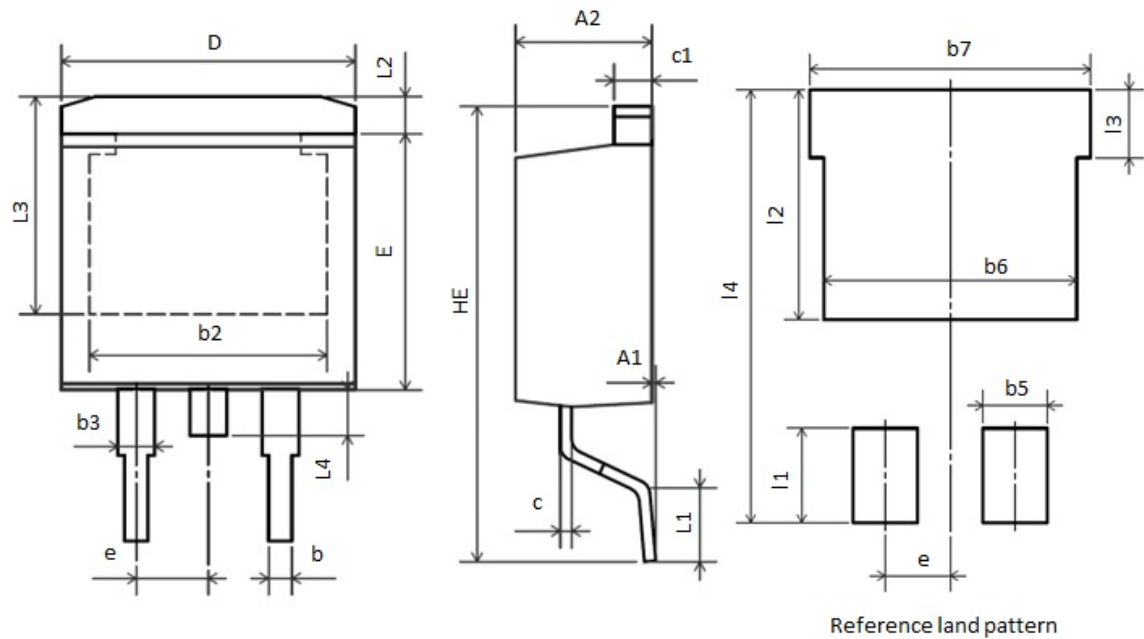
TO-263AB (TO-263AB-3L SHYAD)
