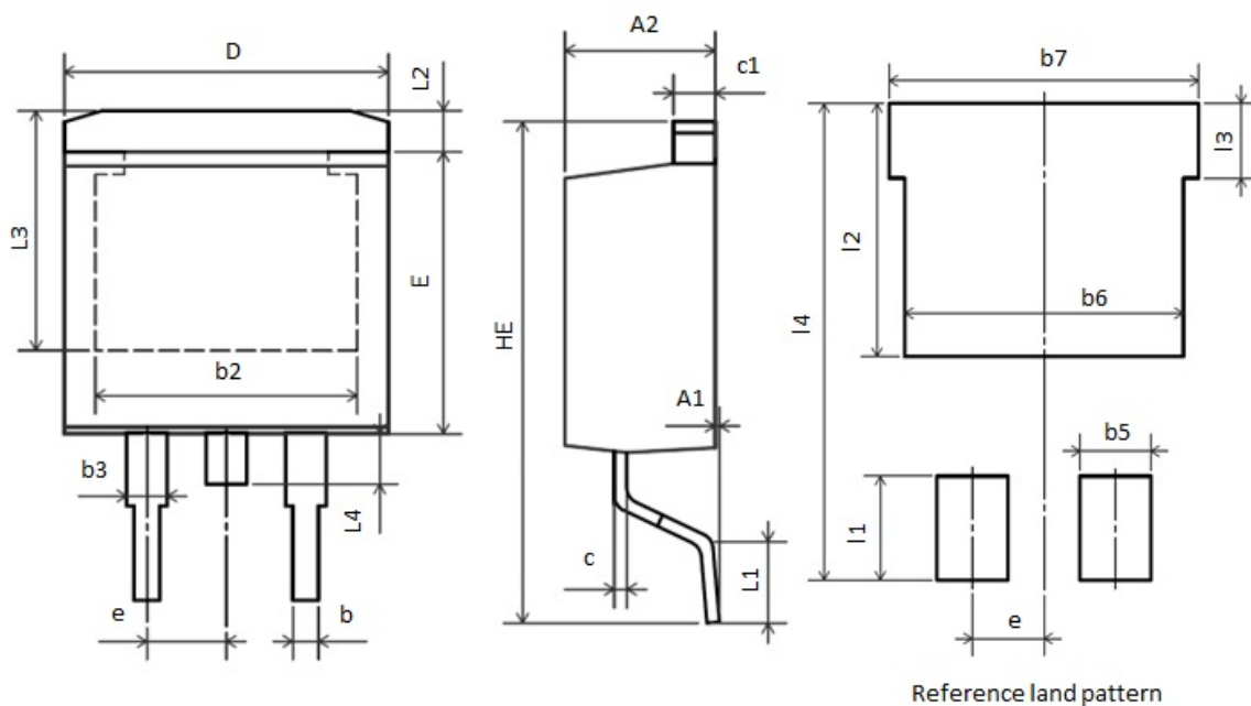
TO-263AB (TO-263AB-3LSHYAD)
