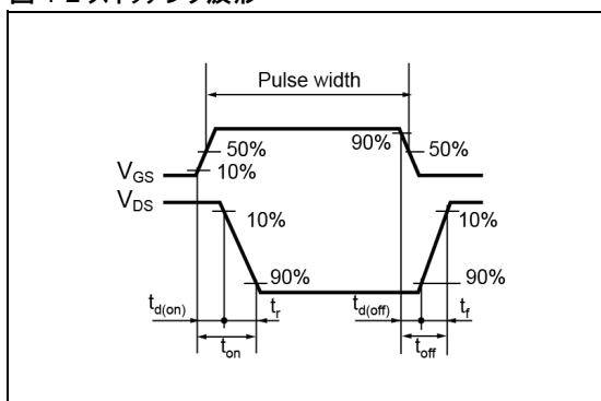
図 1-2 スイッチング波形
