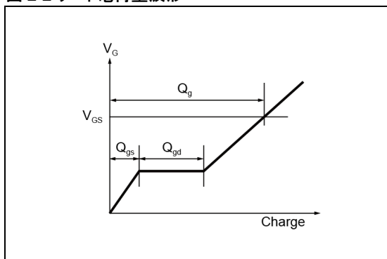
図 2-2 ゲート電荷量波形
