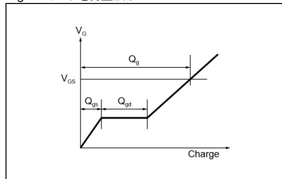
Fig.2-2 ゲート電荷量波形
