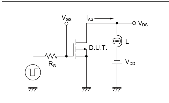
図 3-1 L 負荷測定回路
