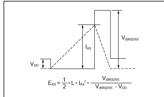
Fig.3-2 アバランシE波形
