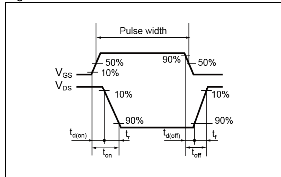
Fig.1-2 スイッチング波形
