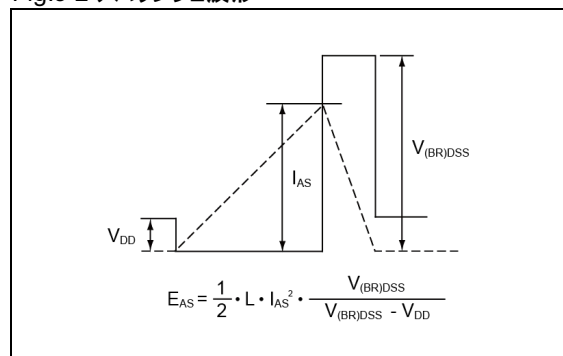
Fig.3-2 アバランシェ波形
