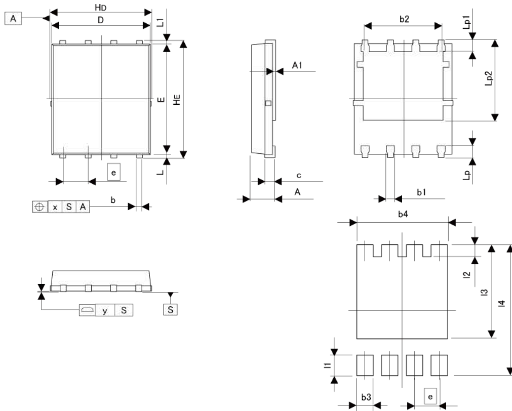
HSOP8 ( 5 x 6 )
