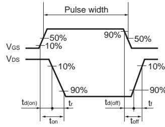
図1-2 スイッチング波形
