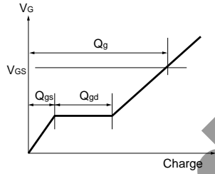
図1-4 ゲート電荷量波形
