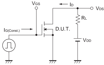
図1-3 ゲート電荷量測定回路
