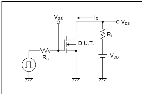
図 1-1 スイッチング時間測定回路
