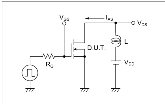
図 3-1 アバランシェ測定回路
