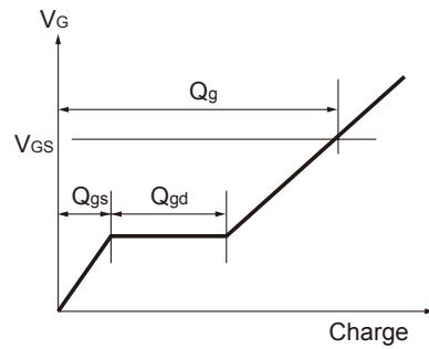
Fig.13 ゲート電荷量波形
