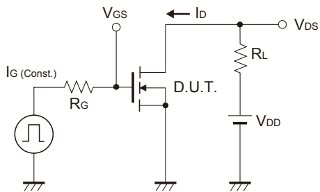
Fig.12 ゲート電荷量測定回路
