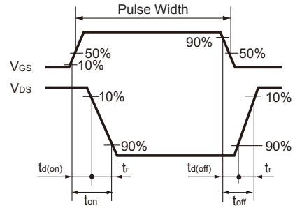
Fig.11 スイッチング波形
