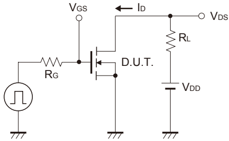
Fig.10 スイッチング時間測定回路
