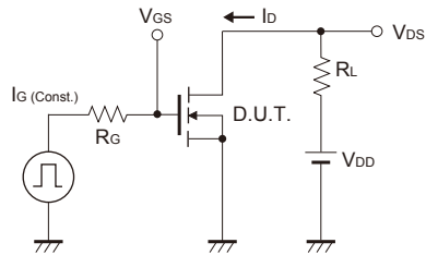
Fig.13 ゲート電荷量測定回路
