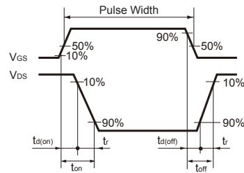
Fig.12 スイッチング波形
