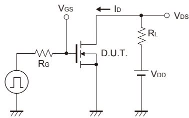
Fig.11 スイッチング時間測定回路
