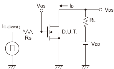
Fig.13 ゲート電荷量測定回路
