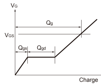
Fig.14 ゲート電荷量波形
