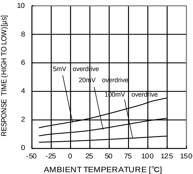
Figure 24. H→L 応答時間－温度特性 (VCC=5V,VRL=5V,RL=5.1kΩ)
