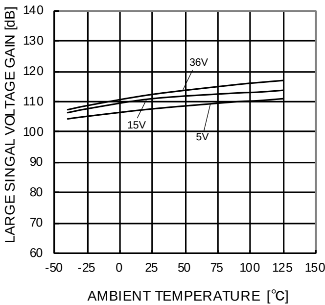
Figure 16. 大振幅電圧利得－温度特性
