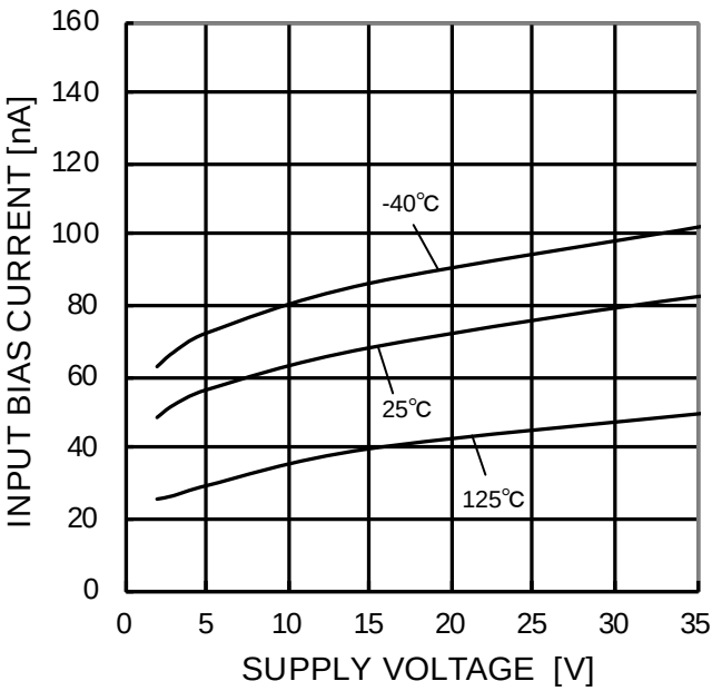
Figure 34. 入力バイアス電流－電源電圧特性
