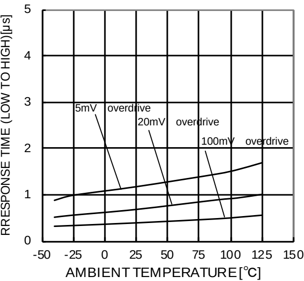
Figure 45. L→H 応答時間－温度特性 (VCC=5V,VRL=5V,RL=5.1kΩ)
