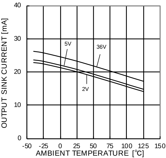
Figure 31. 出力シンク電流－温度特性 ( \text{OUT}=1.5\text{V} )
