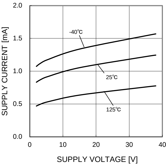
Figure 26. 回路電流－電源電圧特性
