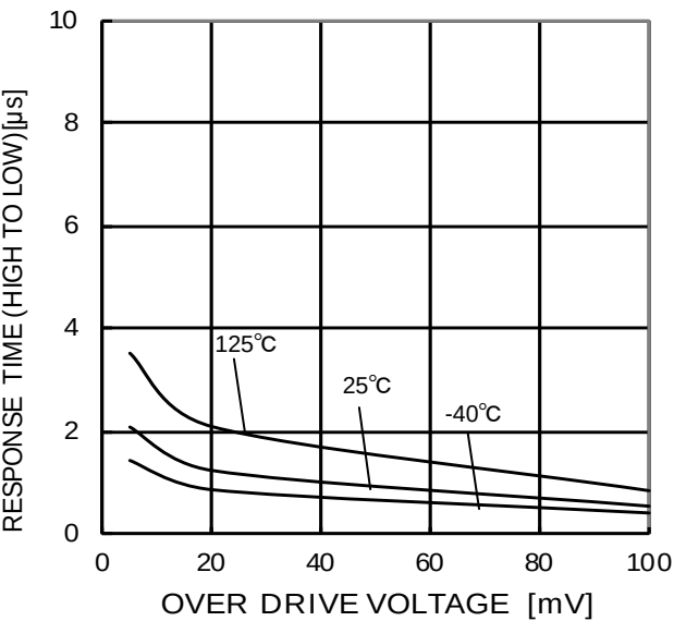
Figure 46. H→L 応答時間－オーバードライブ電圧特性 (VCC=5V,VRL=5V,RL=5.1kΩ)
