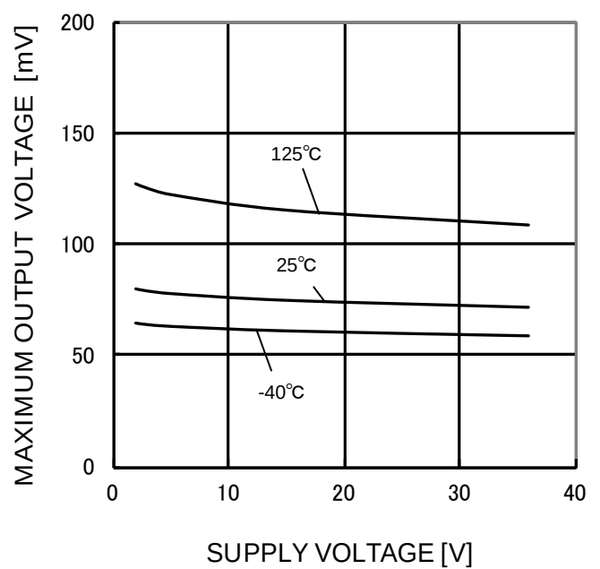
Figure 5. 出力飽和電圧－電源電圧特性 (Isink=4mA)
