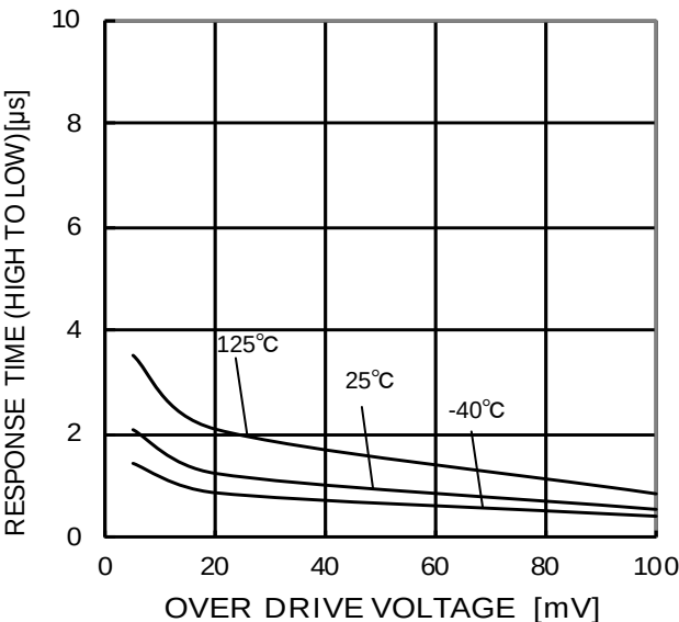
Figure 23. H→L 応答時間－オーバードライブ電圧特性 (VCC=5V,VRL=5V,RL=5.1kΩ)
