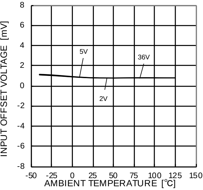
Figure 10. 入力オフセット電圧－温度特性
