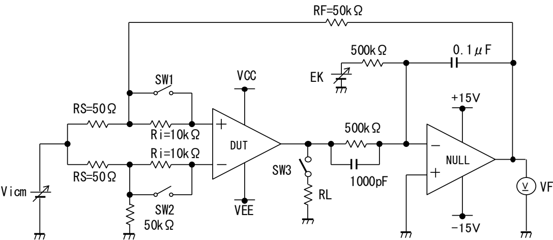
Figure 50. 測定回路 1 (1 チャンネルのみ)
