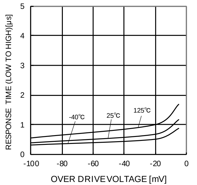
Figure 44. L→H 応答時間－オーバードライブ電圧特性 (VCC=5V,VRL=5V,RL=5.1kΩ)
