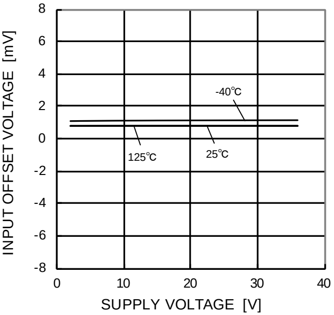
Figure 9. 入力オフセット電圧－電源電圧特性
