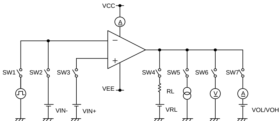
Figure 51. 測定回路 2 (片チャンネルのみ)
