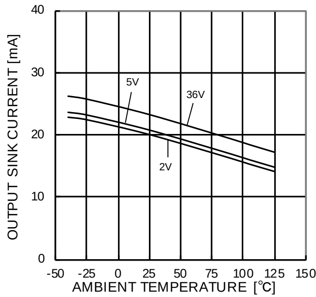
Figure 8. 出力シンク電流－温度特性 ( \text{OUT}=1.5\text{V} )
