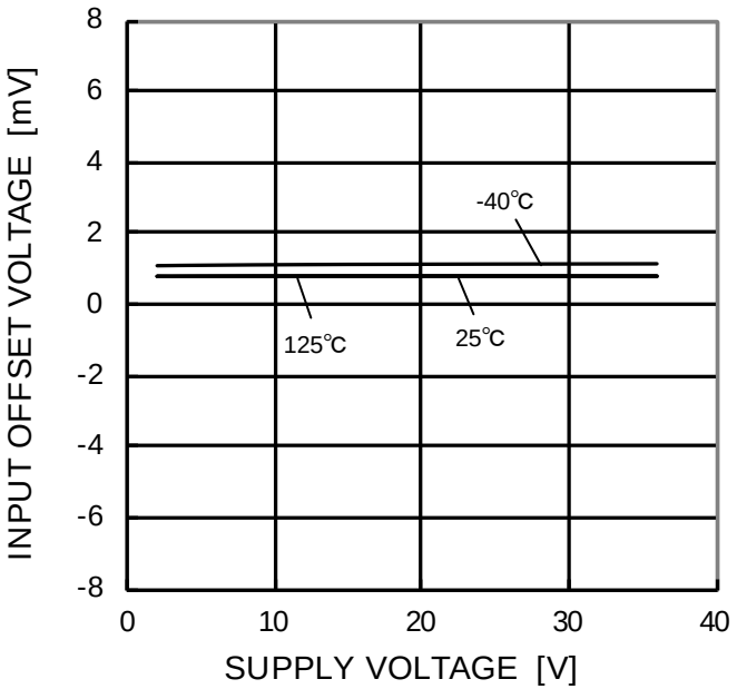
Figure 32. 入力オフセット電圧－電源電圧特性
