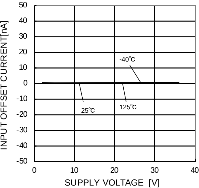
Figure 36. 入力オフセット電流－電源電圧特性
