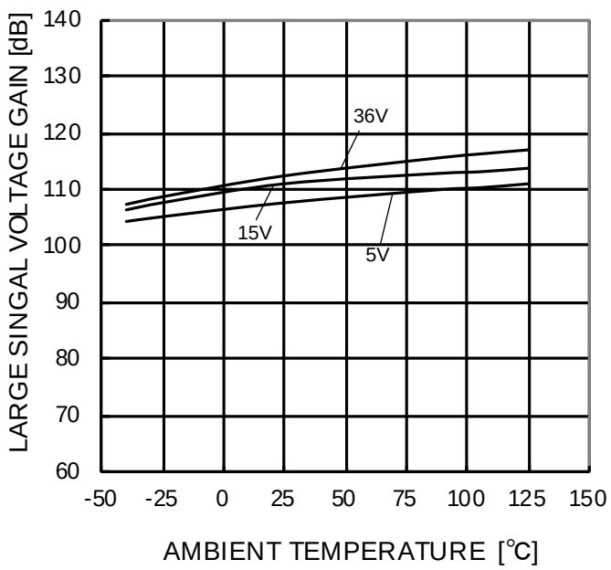
Figure 39. 大振幅電圧利得－温度特性
