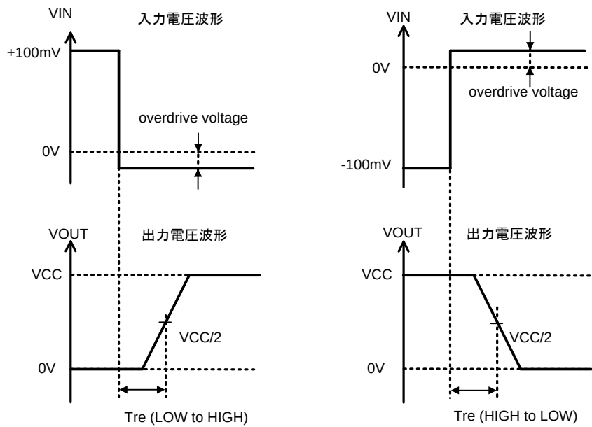
Figure 52. 応答時間測定時 入出力波形
