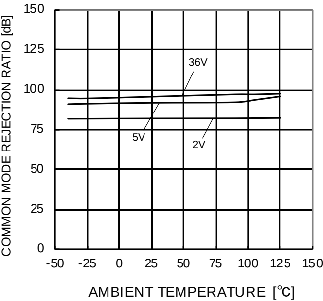
Figure 18. 同相信号除去比－温度特性
