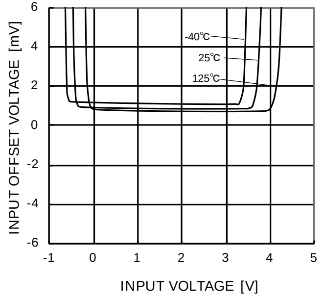
Figure 19. 入力オフセット電圧－同相入力電圧範囲 (VCC=5V)
