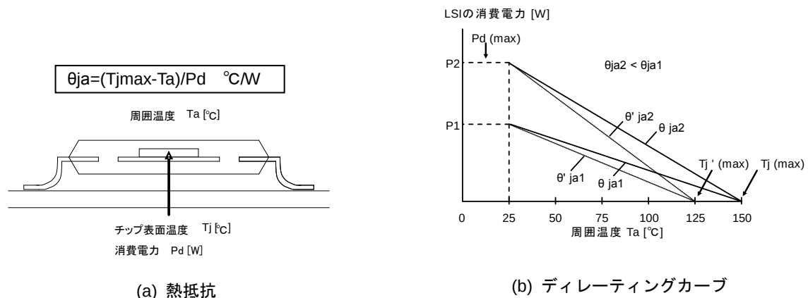
Figure 48. 熱抵抗とディレーティングカーブ
