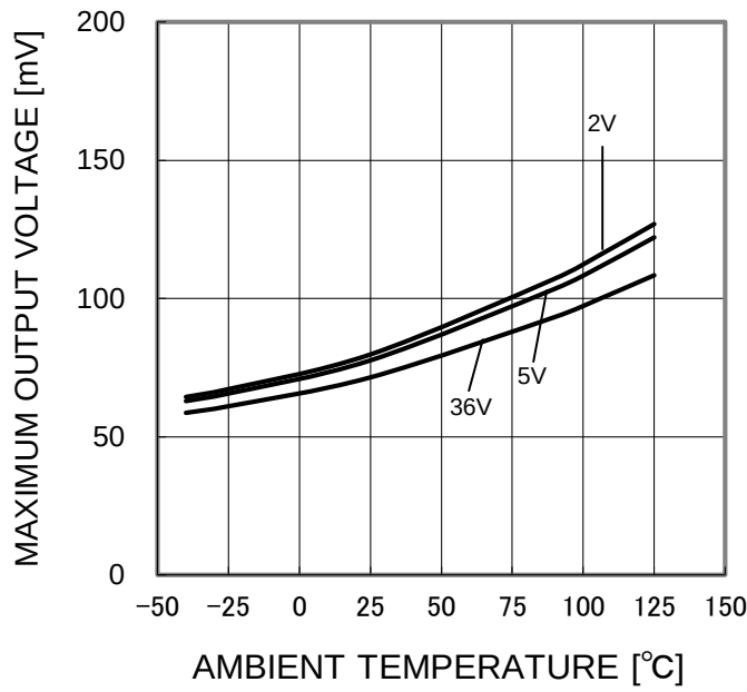
Figure 6. 出力飽和電圧－温度特性 ( I_{\text{sink}}=4\text{mA} )
