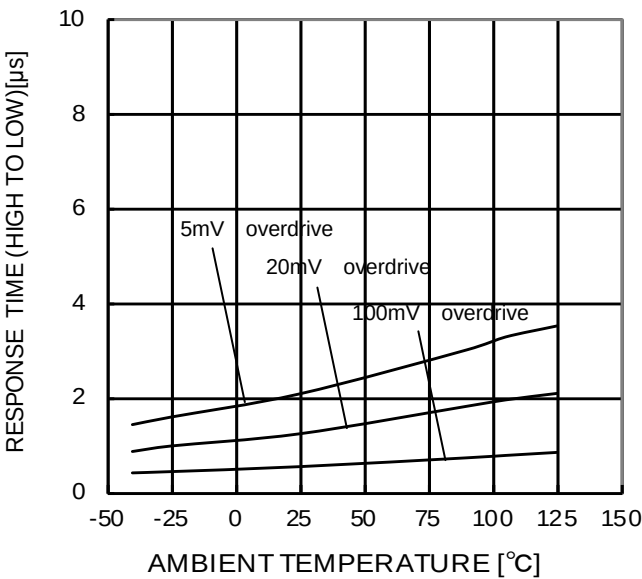
Figure 47. H→L 応答時間－温度特性 (VCC=5V,VRL=5V,RL=5.1kΩ)
