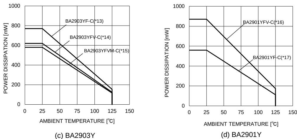
Figure 48. 熱抵抗とディレーティングカーブ
