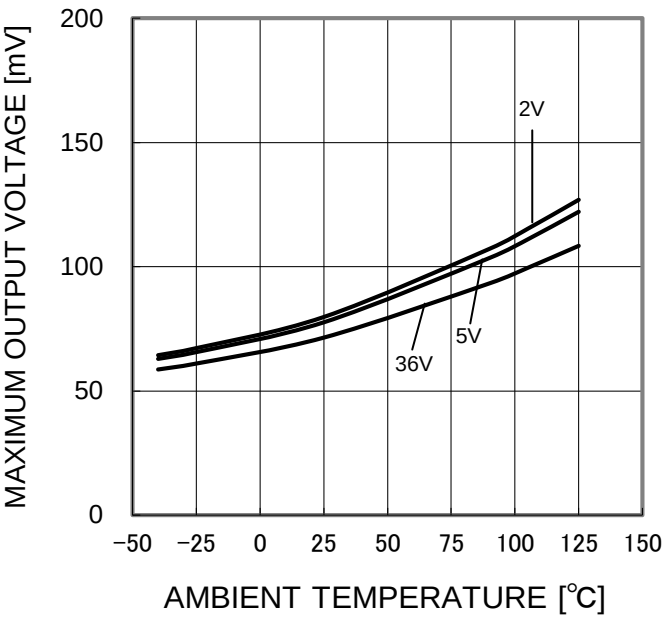
Figure 29. 出力飽和電圧－温度特性 ( I_{\text{sink}}=4\text{mA} )
