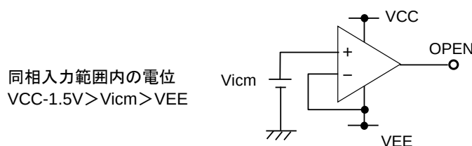
Figure 53. 未使用回路の処理例
