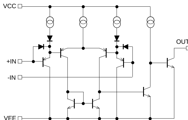
Figure 1. 内部等価回路図 (1 チャンネルのみ)
