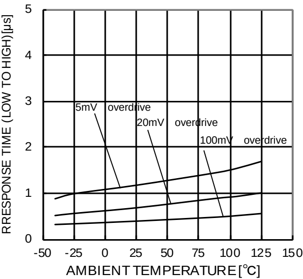
Figure 22. L→H 応答時間－温度特性 (VCC=5V,VRL=5V,RL=5.1kΩ)
