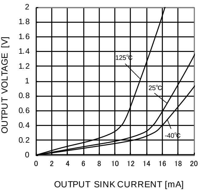
Figure 7. Low レベル出力電圧－出力シンク電流特性 ( V_{\text{CC}}=5\text{V} )
