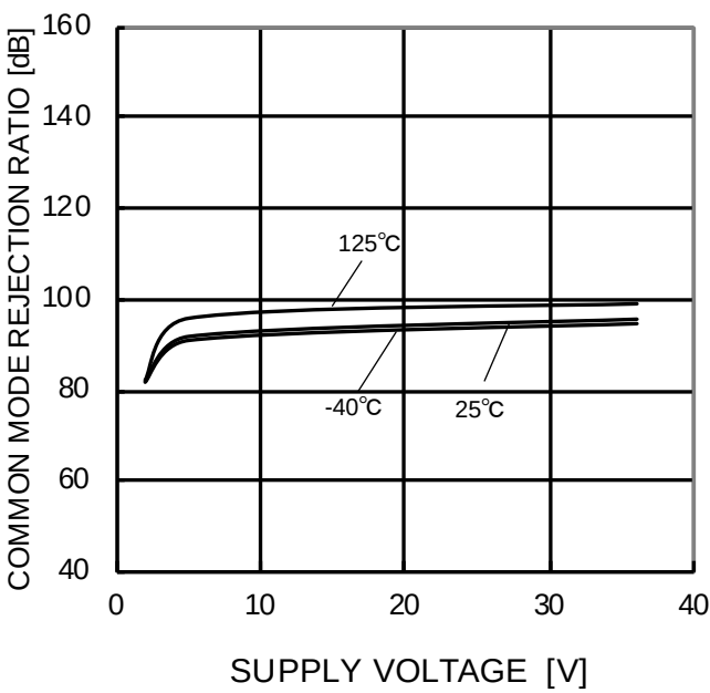
Figure 17. 同相信号除去比－電源電圧特性
