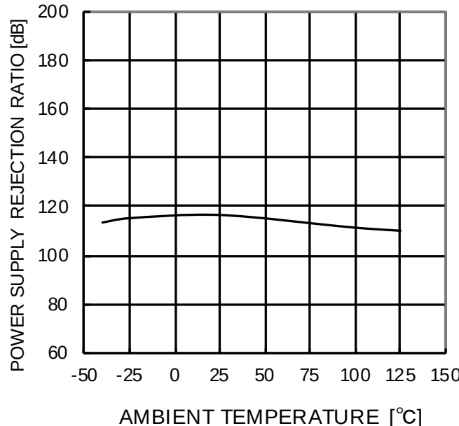
Figure 43. 電源電圧除去比－温度特性
