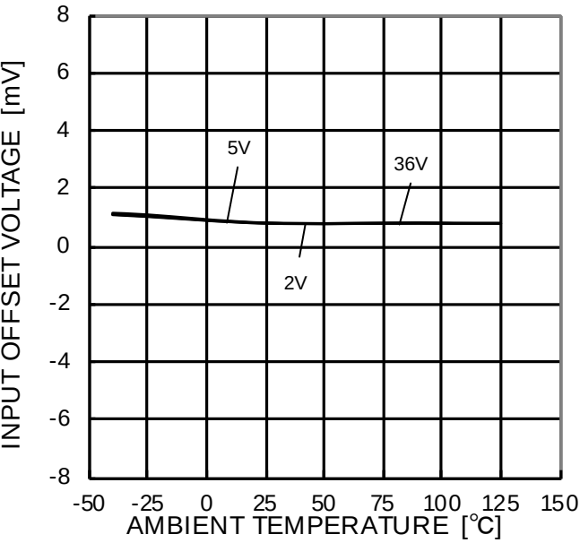
Figure 33. 入力オフセット電圧－温度特性
