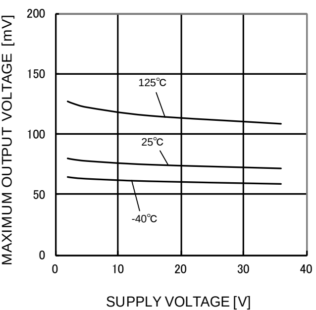
Figure 28. 出力飽和電圧－電源電圧特性 (Isink=4mA)
