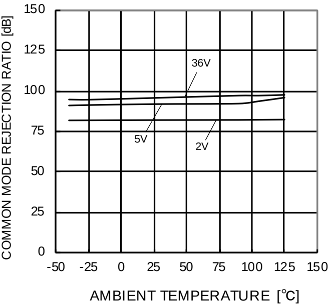
Figure 41. 同相信号除去比－温度特性
