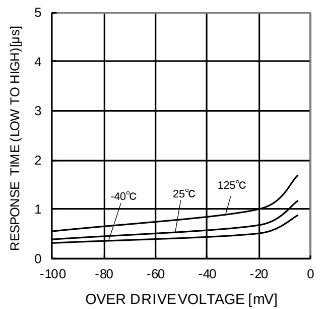
Figure 21. L→H 応答時間－オーバードライブ電圧特性 (VCC=5V,VRL=5V,RL=5.1kΩ)
