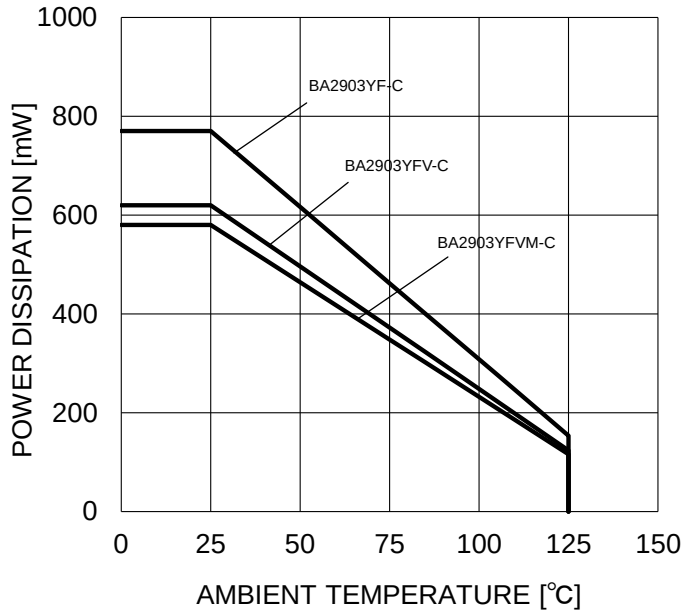
Figure 2. ディレーティングカーブ
