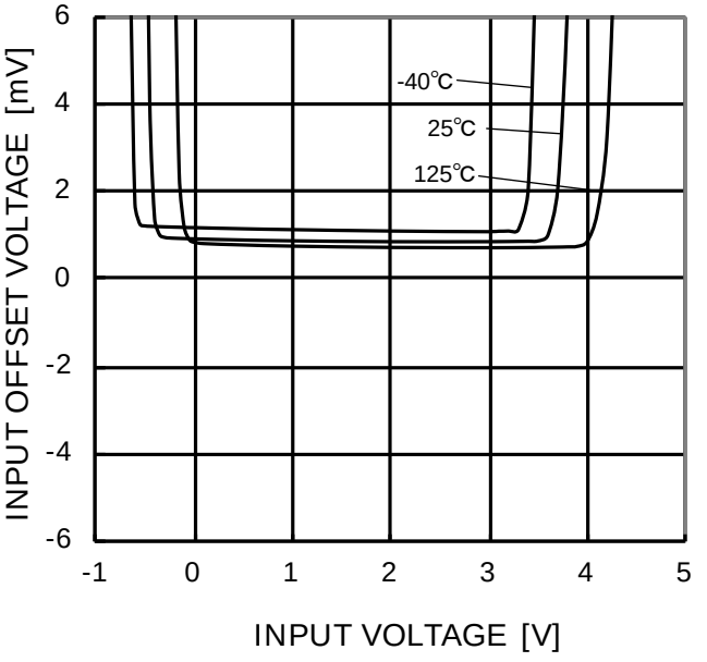
Figure 42. 入力オフセット電圧－同相入力電圧範囲 (VCC=5V)
