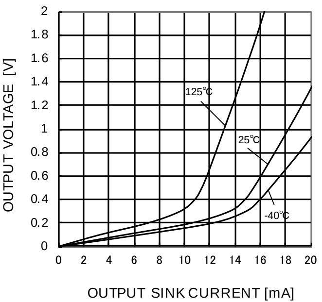
Figure 30. Low レベル出力電圧－出力シンク電流特性 ( V_{\text{CC}}=5\text{V} )
