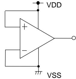
Figure 27.未使用回路処理例
