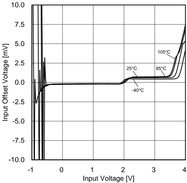
Figure 15. 入力オフセット電圧－入力電圧 ( V_{DD}=3V )
