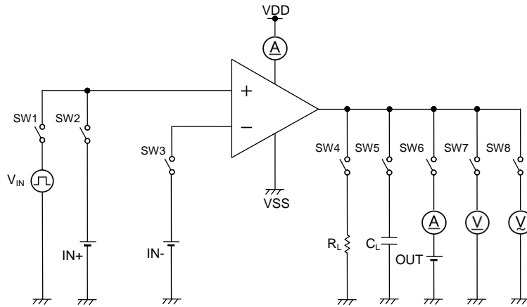
Figure 24. 測定回路 2
