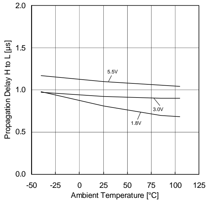
Figure 22. 立ち下がり伝播遅延-温度特性 ( C_L=15\text{pF} , I_N=1.5\text{V} 100mV Overdrive)
