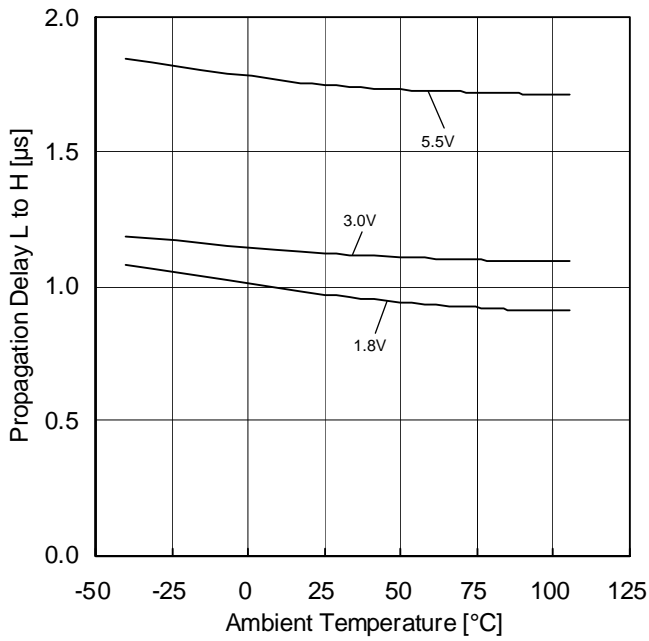
Figure 21. 立ち上がり伝搬遅延時間-温度特性 ( C_L=15\text{pF} , I_N=1.5\text{V} 100mV Overdrive)
