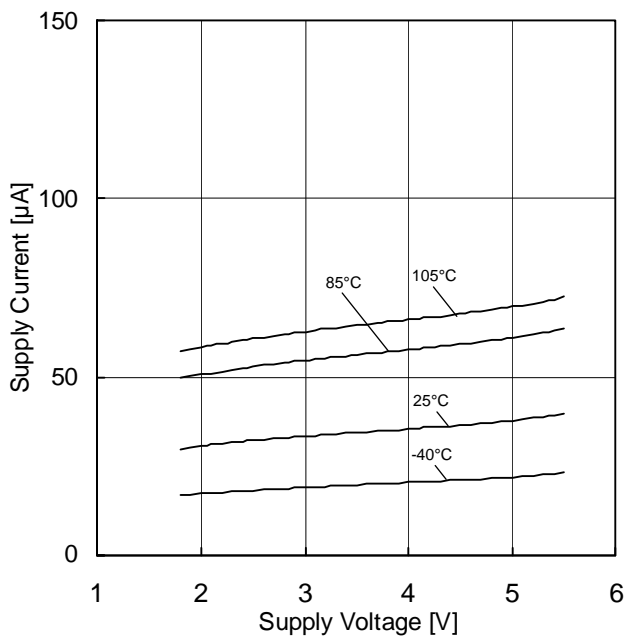
Figure 25. 回路電流 - 電源電圧特性
