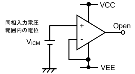
Figure 24. 未使用回路の処理例
