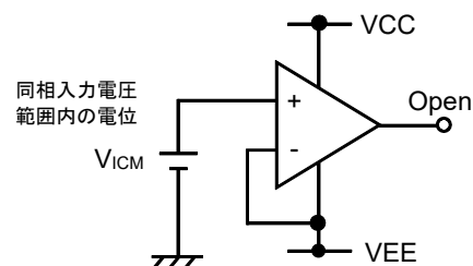
Figure 20. 未使用回路の処理例
