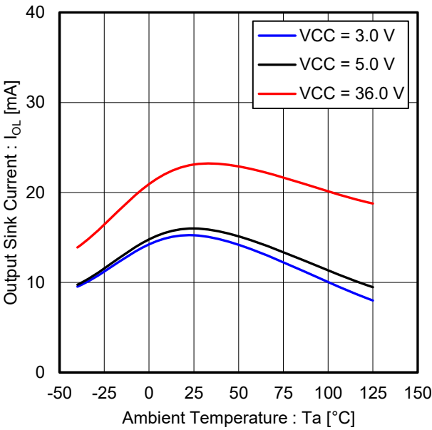
Figure 6. 出力シンク電流 vs 温度 ( V_{OUT} = 1.5\text{ V} )
