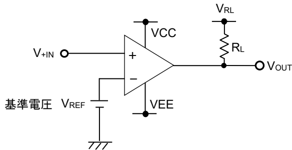
Figure 21. -IN を基準とした場合の回路例
