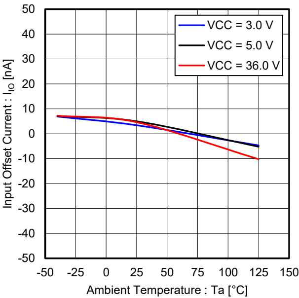
Figure 12. 入力オフセット電流 vs 温度
