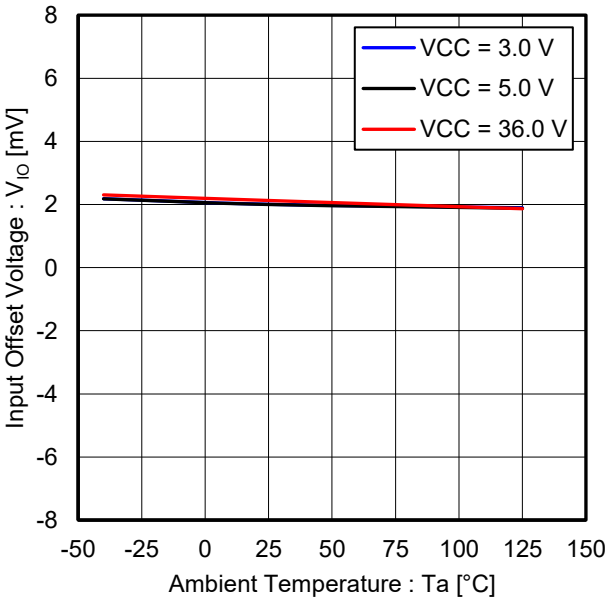
Figure 8. 入力オフセット電圧 vs 温度
