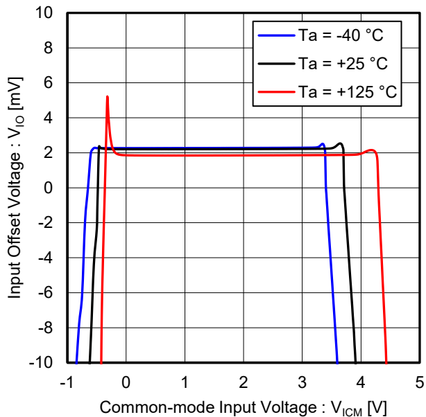
Figure 15. 入力オフセット電圧 vs 同相入力電圧 ( V_{CC} = 5\text{ V} )
