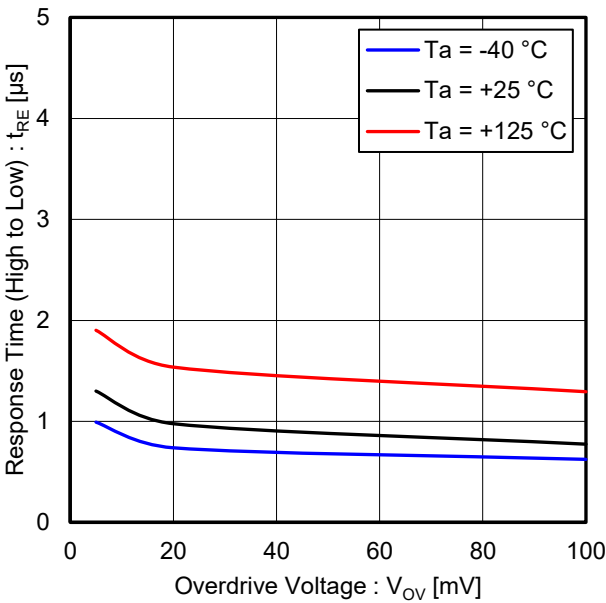
Figure 18. 応答時間 (High to Low) vs オーバードライブ電圧 ( V_{CC} = 5\text{ V} , V_{RL} = 5\text{ V} , R_L = 5.1\text{ k}\Omega )
