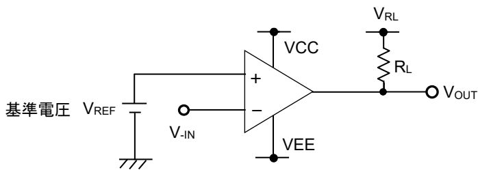
Figure 22. +IN を基準とした場合の回路例
