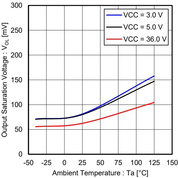
Figure 4. 出力飽和電圧 vs 温度 ( I_{OL} = 4\text{ mA} )
