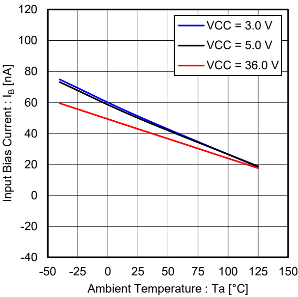
Figure 10. 入力バイアス電流 vs 温度
