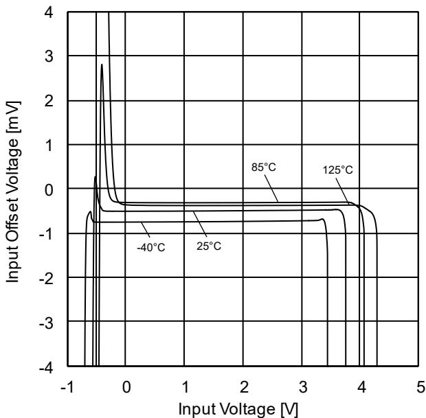
Figure 15. 入力オフセット電圧-入力電圧特性 (同相入力電圧範囲) (V CC =5V)
