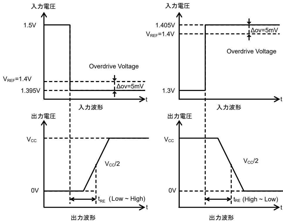
Figure 41. 応答時間測定時 入出力波形
