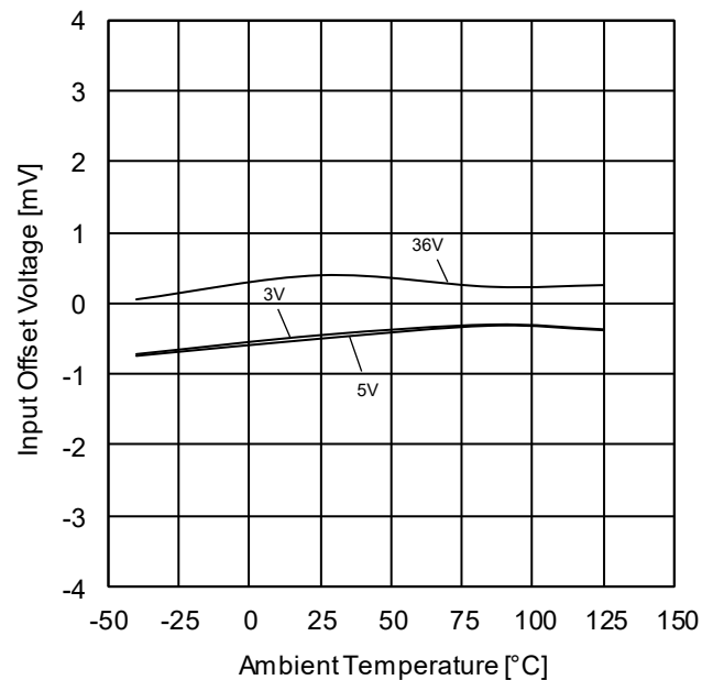
Figure 27. 入力オフセット電圧—温度特性
