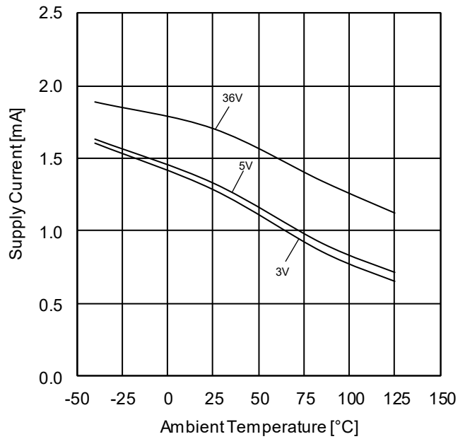
Figure 21. 回路電流-温度特性
