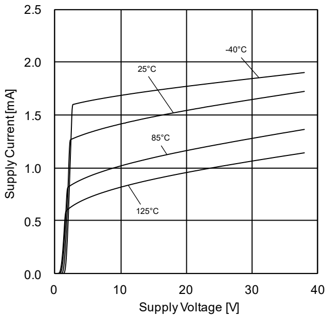
Figure 20. 回路電流-電源電圧特性
