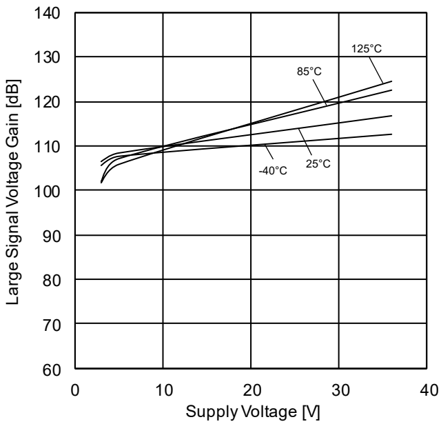
Figure 32. 大振幅電圧利得－電源電圧特性 ( R_L=15k\Omega )
