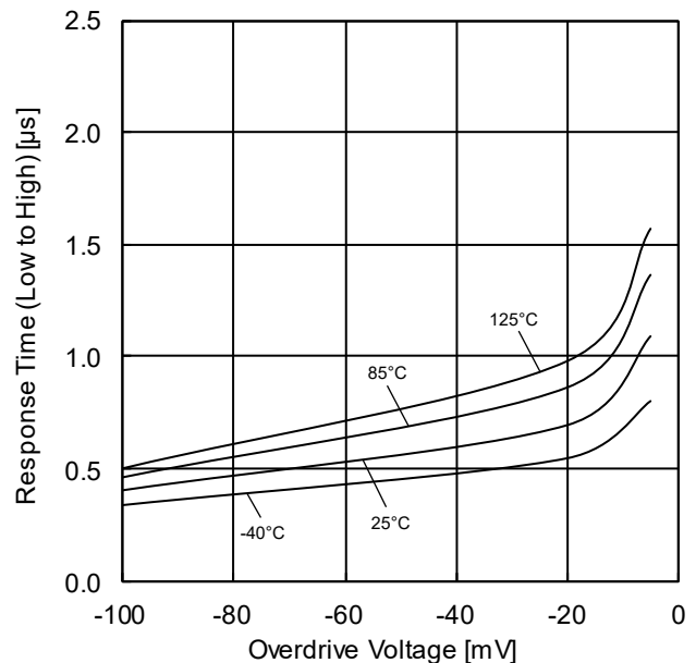
Figure 16. L-H 応答時間-オーバードライブ電圧特性 (V CC =5V, V RL =5V, R L =5.1kΩ)
