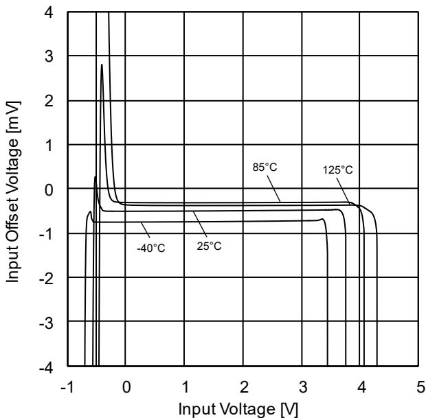
Figure 34. 入力オフセット電圧－入力電圧特性 (同相入力電圧範囲) ( V_{CC}=5V )
