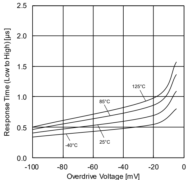
Figure 35. L-H 応答時間－オーバードライブ電圧特性 ( V_{CC}=5V, V_{RL}=5V, R_L=5.1k\Omega )
