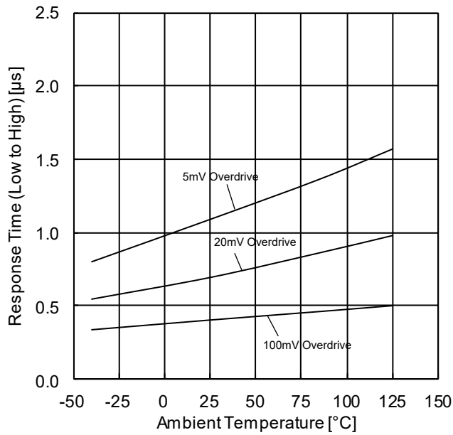
Figure 36. L-H 応答時間-温度特性 ( V_{CC}=5V, V_{RL}=5V, R_L=5.1k\Omega )
