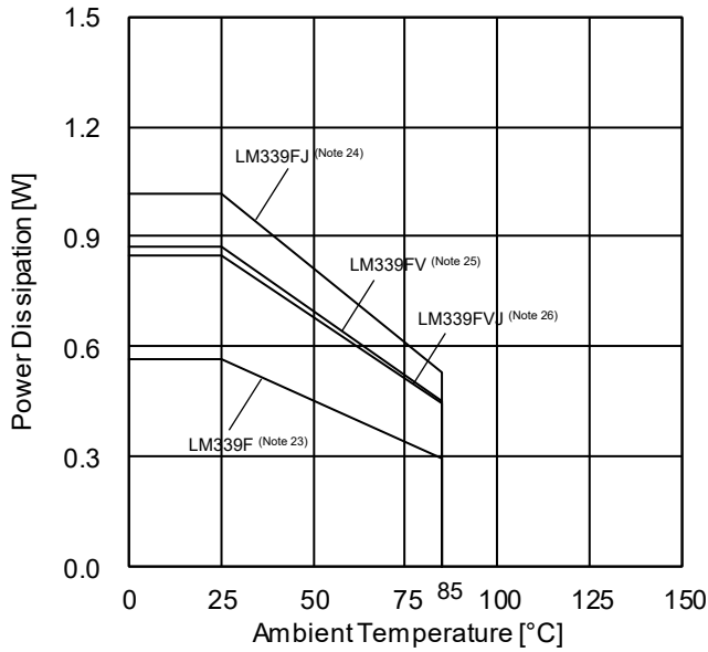
(e) LM339xxx
