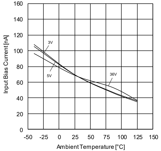
Figure 29. 入力バイアス電流－温度特性
