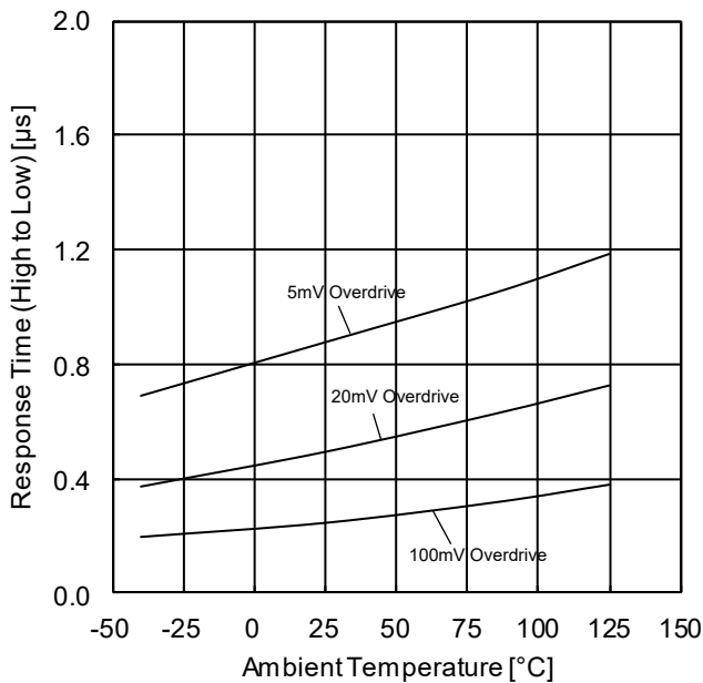
Figure 38. H-L 応答時間-温度特性 ( V_{CC}=5V, V_{RL}=5V, R_L=5.1k\Omega )
