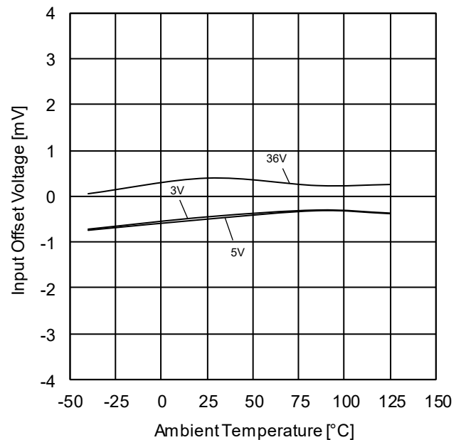
Figure 8. 入力オフセット電圧—温度特性
