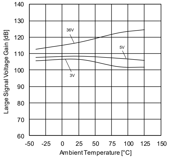
Figure 33. 大振幅電圧利得－温度特性 ( R_L=15k\Omega )
