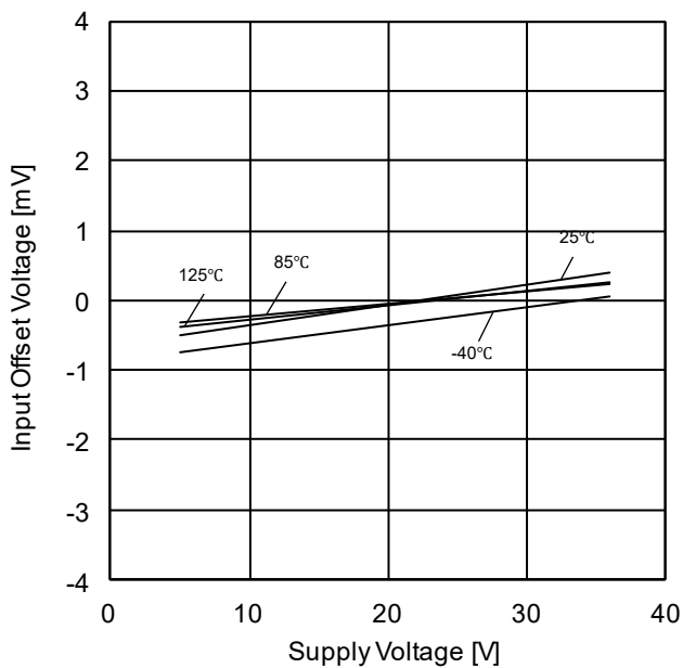
Figure 7. 入力オフセット電圧-電源電圧特性
