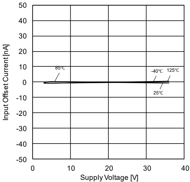
Figure 30. 入力オフセット電流－電源電圧特性
