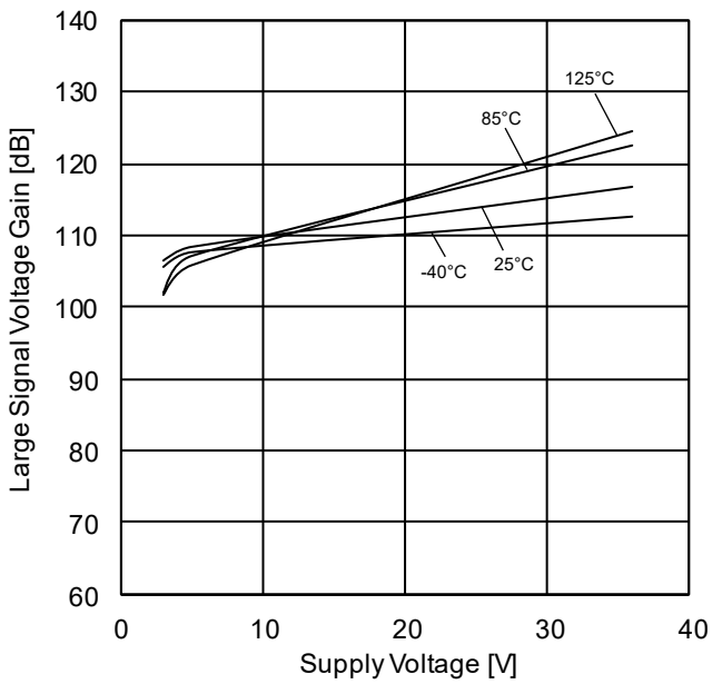
Figure 13. 大振幅電圧利得-電源電圧特性 (R L =15kΩ)
