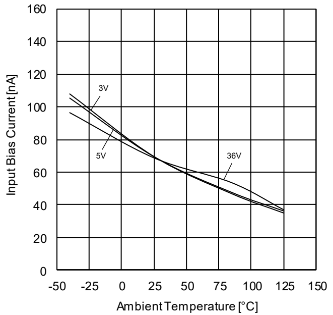
Figure 10. 入力バイアス電流—温度特性
