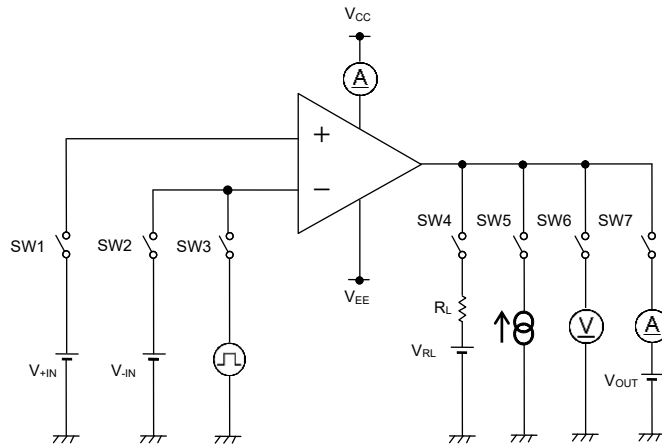
Figure 40. 測定回路 2 (1 チャンネルのみ)
