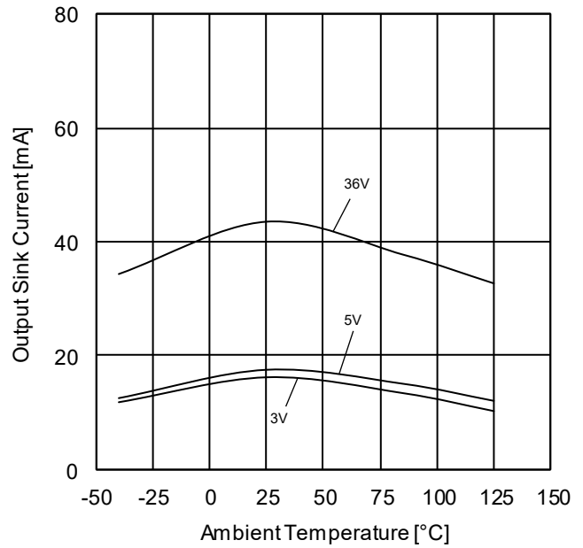
Figure 6. 出力シンク電流-温度特性 ( V_{OUT}=V_{CC} )
