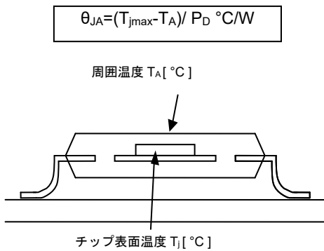
(a) 熱抵抗
