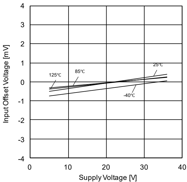
Figure 26. 入力オフセット電圧-電源電圧特性
