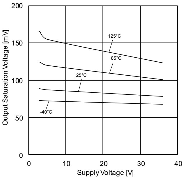
Figure 3. 出力飽和電圧-電源電圧特性 ( I_{SINK}=4mA )
