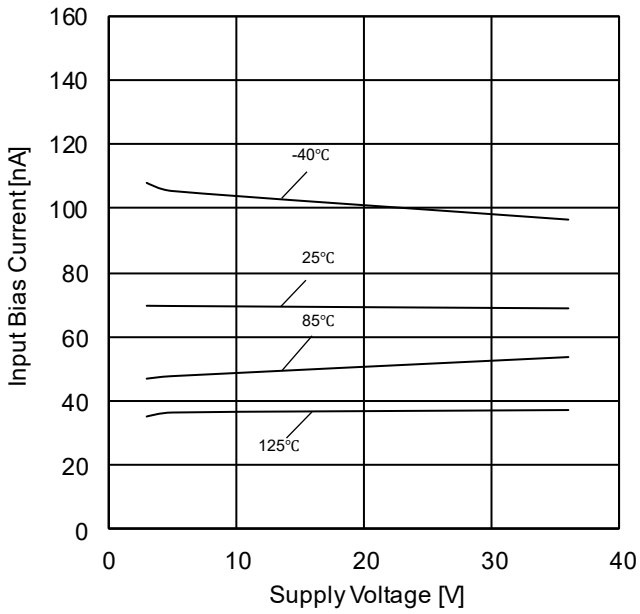
Figure 28. 入力バイアス電流－電源電圧特性
