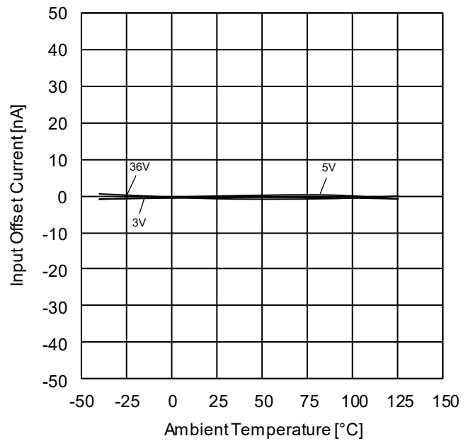
Figure 31. 入力オフセット電流－温度特性
