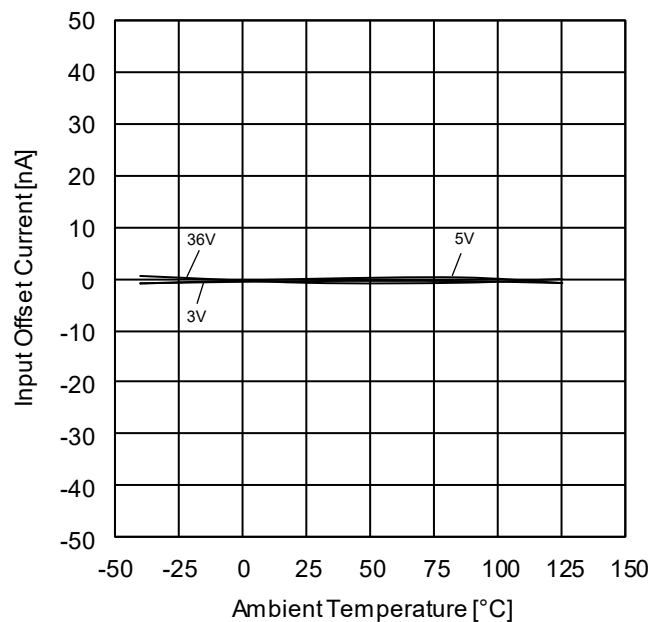
Figure 12. 入力オフセット電流—温度特性
