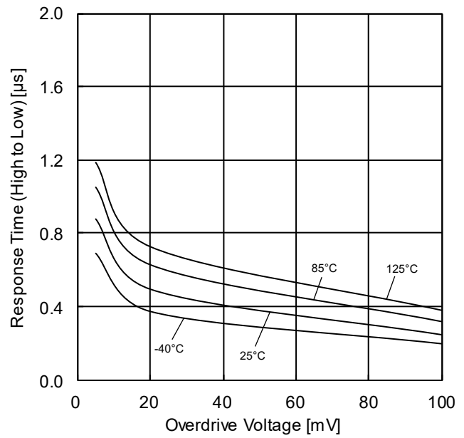
Figure 37. H-L 応答時間-オーバードライブ電圧特性 ( V_{CC}=5V, V_{RL}=5V, R_L=5.1k\Omega )
