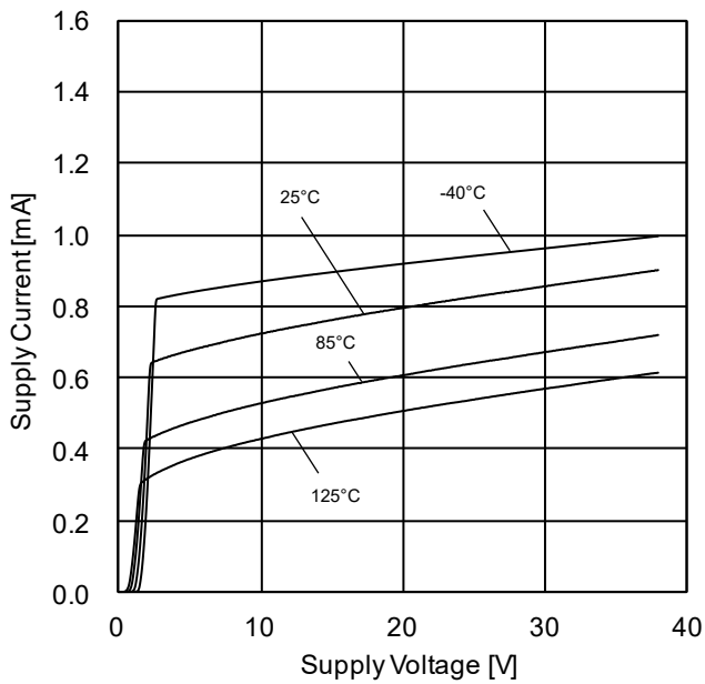
Figure 1. 回路電流－電源電圧特性
