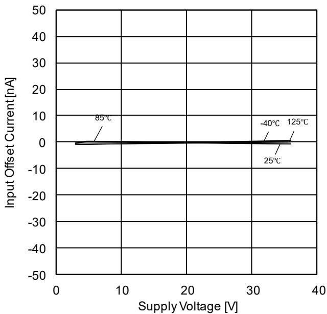
Figure 11. 入力オフセット電流—電源電圧特性
