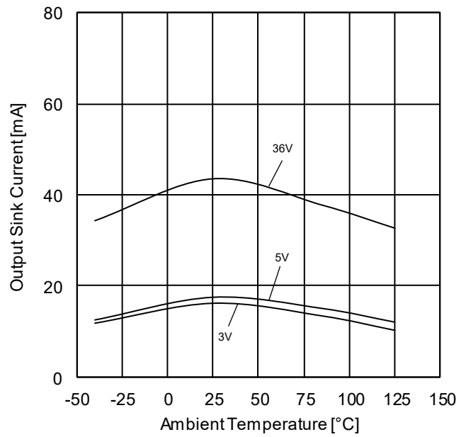
Figure 25. 出力シンク電流-温度特性 ( V_{OUT}=V_{CC} )
