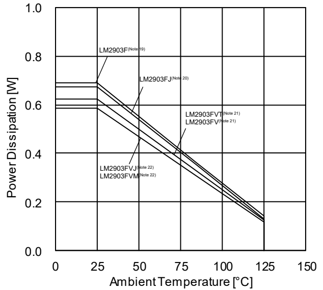
(d) LM2903xxx
