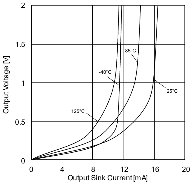
Figure 24. 出力電圧-出力シンク電流特性 ( V_{CC}=5V )
