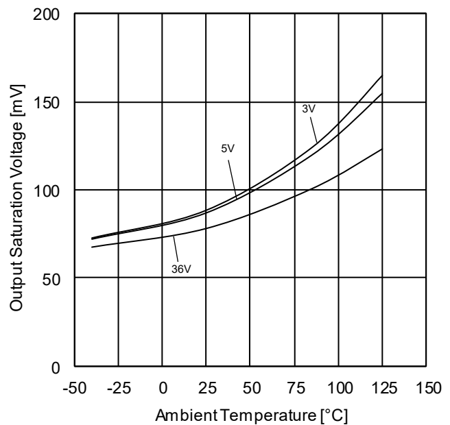
Figure 4. 出力飽和電圧-温度特性 ( I_{SINK}=4mA )
