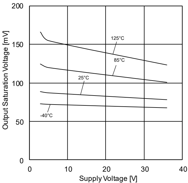
Figure 22. 出力飽和電圧-電源電圧特性 ( I_{SINK}=4mA )
