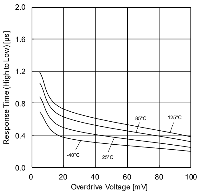
Figure 18. H-L 応答時間-オーバードライブ電圧特性 ( V_{CC}=5V , V_{RL}=5V , R_L=5.1k\Omega )
