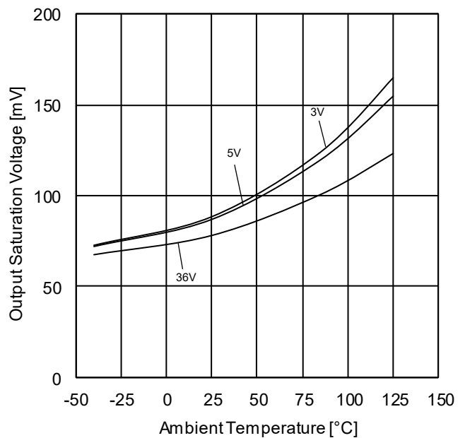
Figure 23. 出力飽和電圧-温度特性 ( I_{SINK}=4mA )
