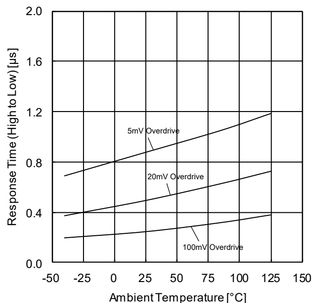
Figure 19. H-L 応答時間-温度特性 ( V_{CC}=5V , V_{RL}=5V , R_L=5.1k\Omega )
