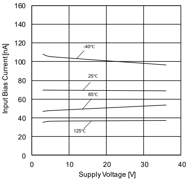
Figure 9. 入力バイアス電流—電源電圧特性
