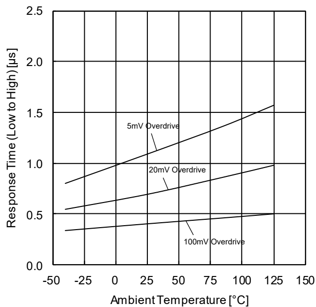
Figure 17. L-H 応答時間-温度特性 ( V_{CC}=5V , V_{RL}=5V , R_L=5.1k\Omega )
