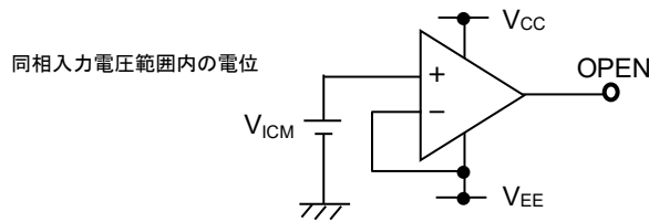
Figure 42. 未使用回路処理例
