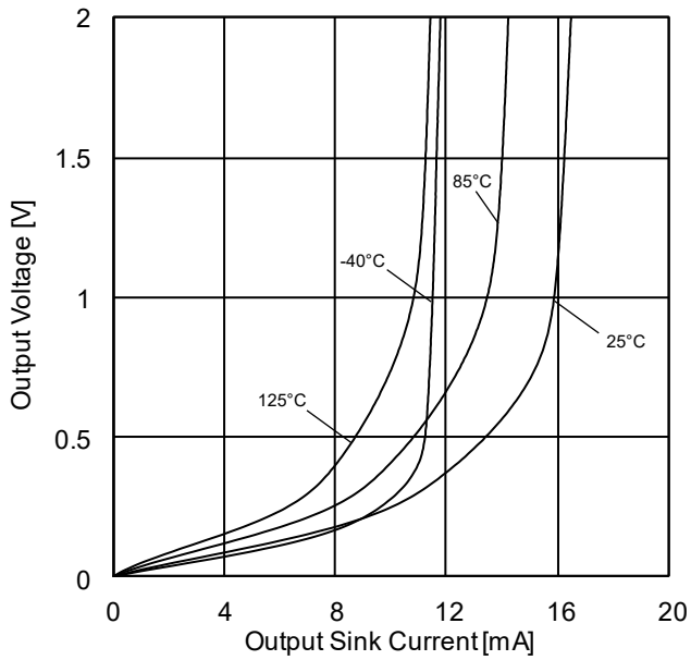
Figure 5. 出力電圧-出力シンク電流特性 ( V_{CC}=5V )
