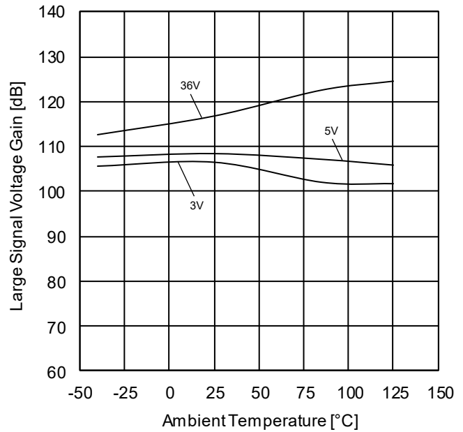
Figure 14. 大振幅電圧利得-温度特性 (R L =15kΩ)
