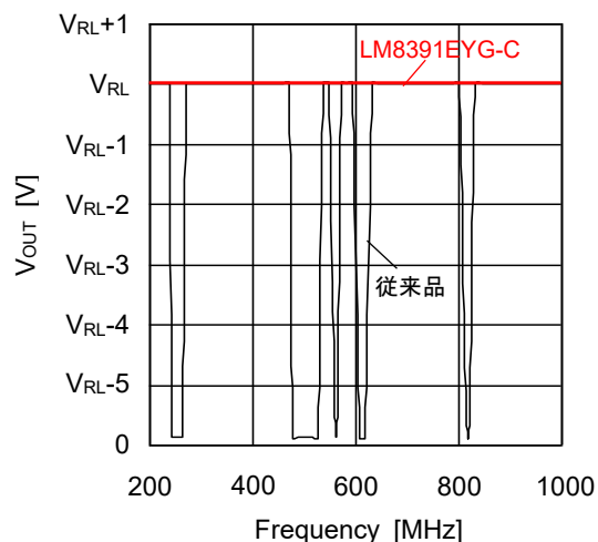
Figure 20. EMI 特性データ(H 出力時)
