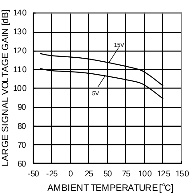
Figure 70. 大振幅電圧利得－温度特性 (RL=2kΩ)
