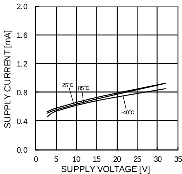
Figure 27. 回路電流－電源電圧特性
