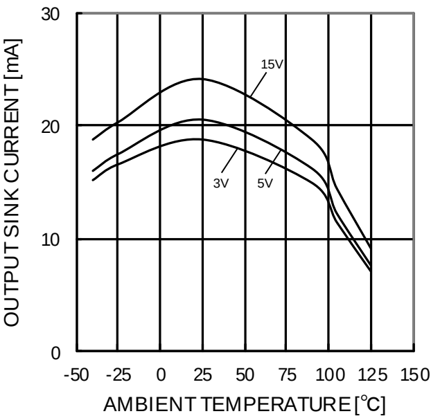
Figure 58. 出力シンク電流－温度特性 (OUT=VCC)
