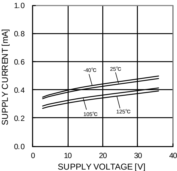
Figure 51. 回路電流－電源電圧特性
