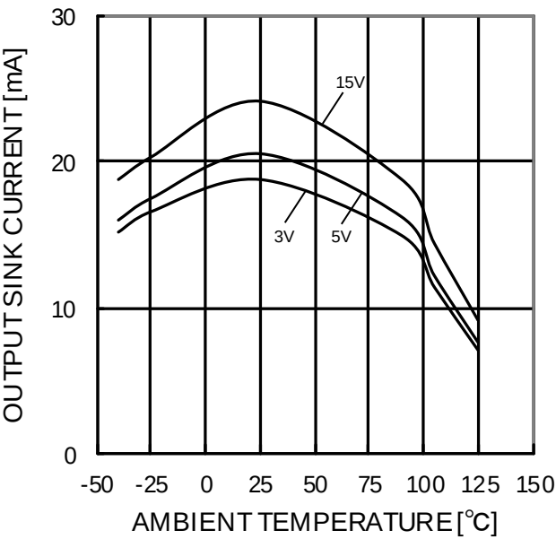
Figure 82. 出力シンク電流－温度特性 (OUT=VCC)
