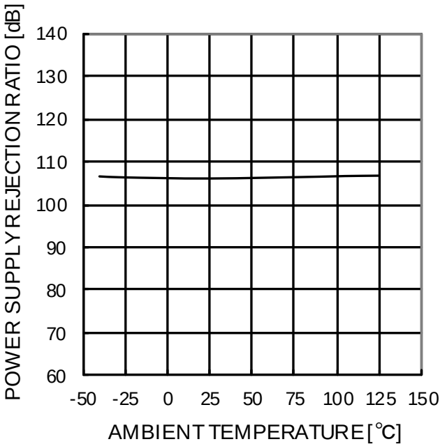
Figure 73. 電源電圧除去比－温度特性
