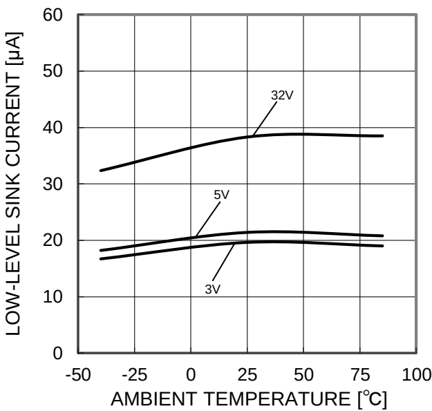
Figure 12. LOW レベルシンク電流－温度特性 (OUT=0.2V)
