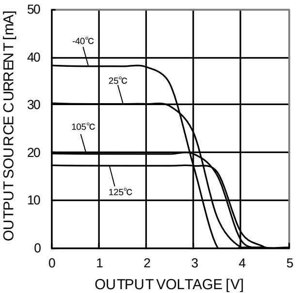
Figure 79. 出力ソース電流－出力電圧特性 (VCC=5V)
