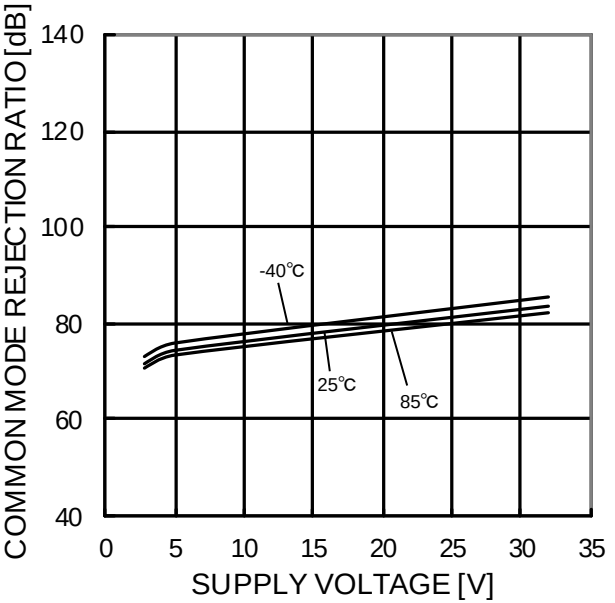
Figure 23. 同相信号除去比－電源電圧特性
