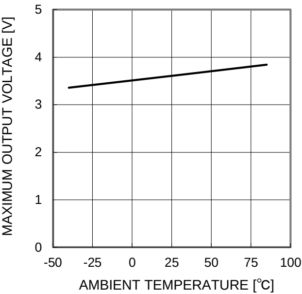
Figure 6. 最大出力電圧－温度特性 (VCC=5V,RL=2kΩ)
