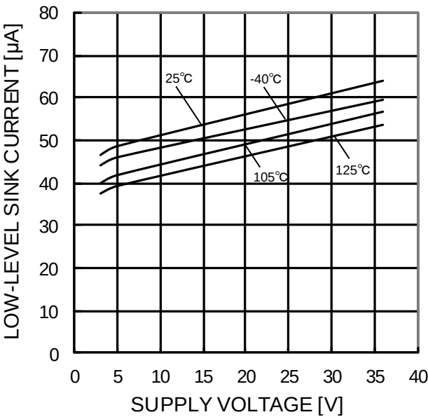
Figure 59. LOW レベルシンク電流－電源電圧特性 (OUT=0.2V)
