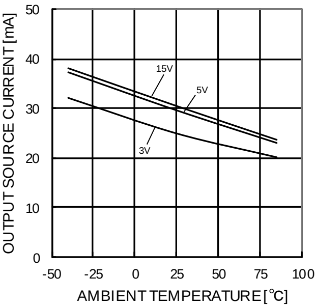
Figure 32. 出力ソース電流－温度特性 (OUT=0V)
