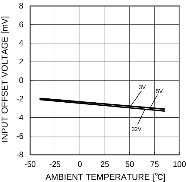
Figure 14. 入力オフセット電圧－温度特性 ( V_{ICM}=0V , OUT=1.4V )
