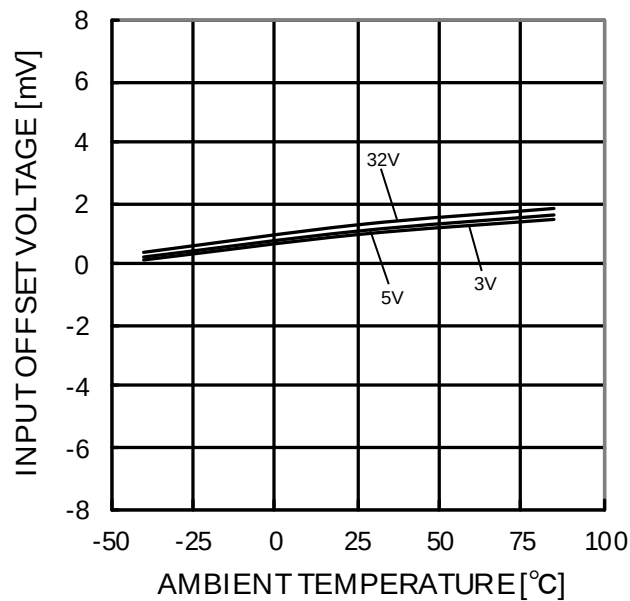
Figure 38. 入力オフセット電圧－温度特性 ( V_{ICM}=0V , OUT=1.4V )
