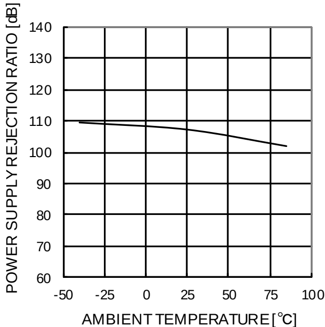
Figure 49. 電源電圧除去比－温度特性
