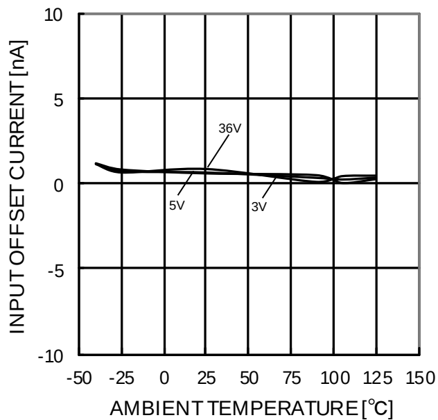
Figure 68. 入力オフセット電流—温度特性 ( V_{ICM}=0V , OUT=1.4V )
