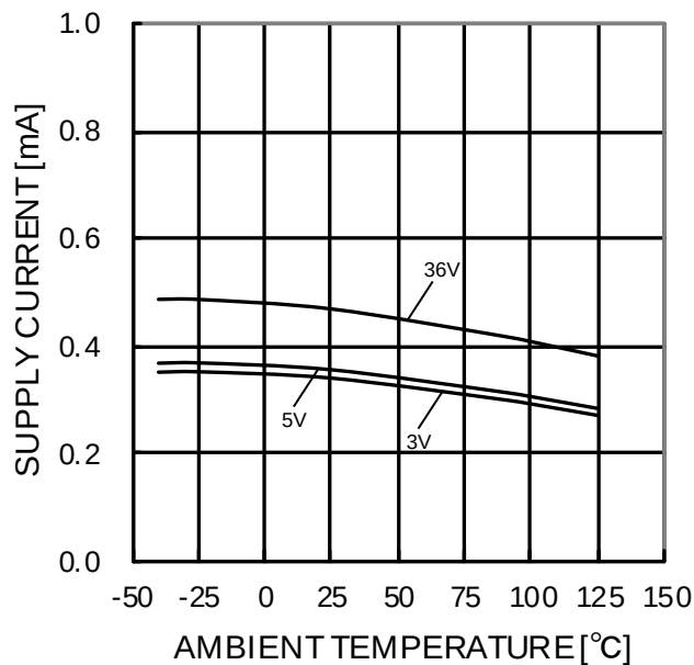
Figure 52. 回路電流－温度特性
