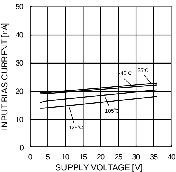
Figure 87. 入力バイアス電流－電源電圧特性 ( V_{ICM}=0V , OUT=1.4V )
