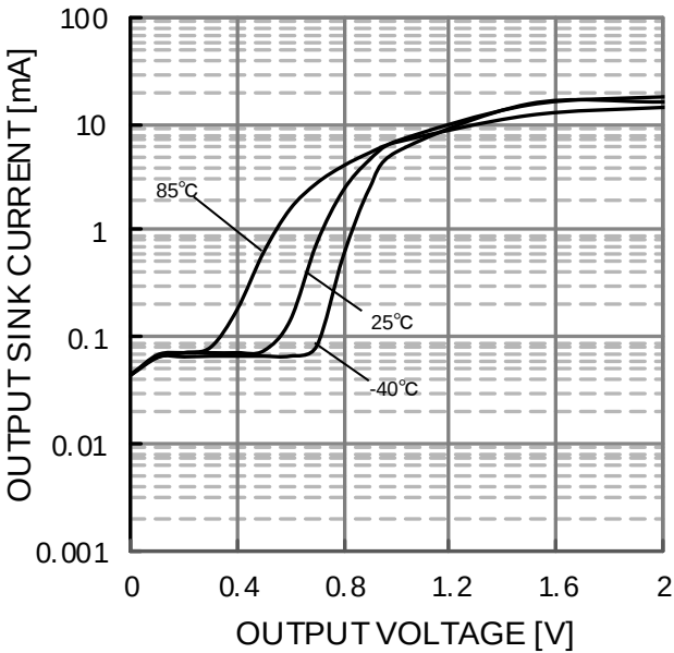
Figure 33. 出力シンク電流－出力電圧特性 (VCC=5V)
