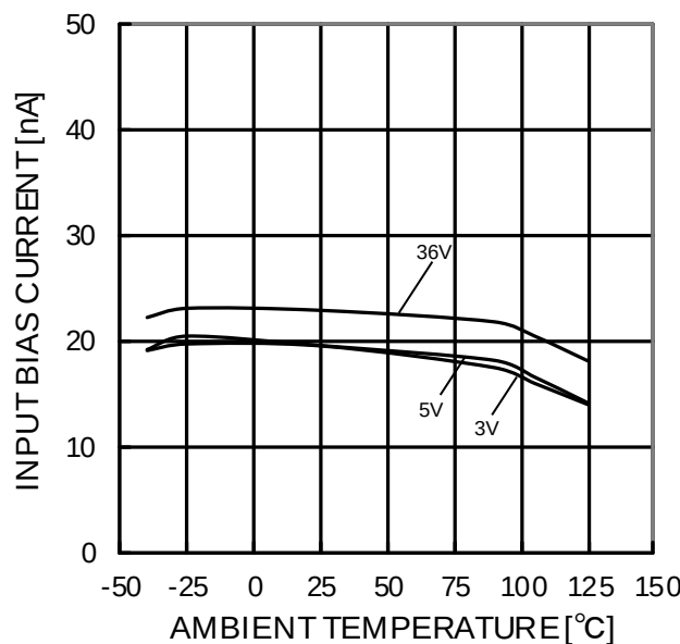
Figure 64. 入力バイアス電流－温度特性 ( V_{ICM}=0V , OUT=1.4V )
