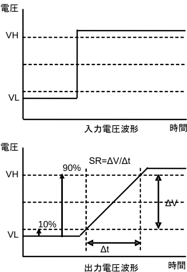
Figure 100. スルーレート測定時 入出力波形
