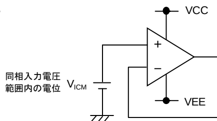
Figure 104. 未使用回路の処理例
