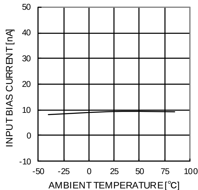
Figure 41. 入力バイアス電流－温度特性 ( V_{CC}=30V , V_{ICM}=28V , OUT=1.4V )
