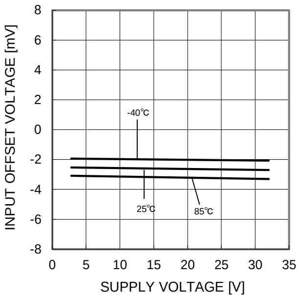
Figure 13. 入力オフセット電圧－電源電圧特性 (V ICM =0V, OUT=1.4V)
