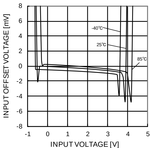
Figure 42. 入力オフセット電圧—同相入力電圧特性 (VCC=5V)
