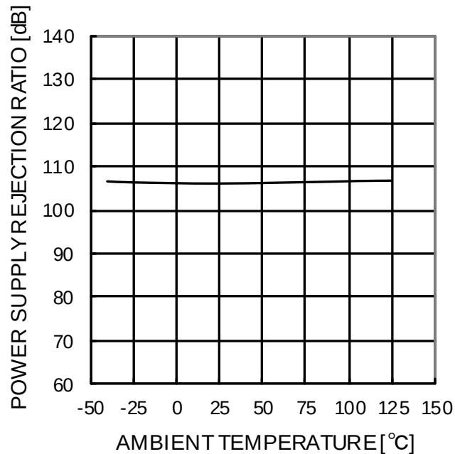
Figure 97. 電源電圧除去比－温度特性
