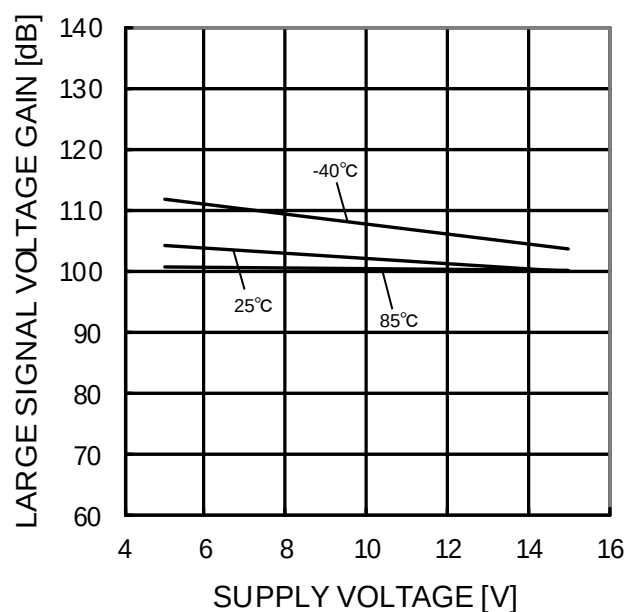
Figure 45. 大振幅電圧利得—電源電圧特性 (R L =2kΩ)
