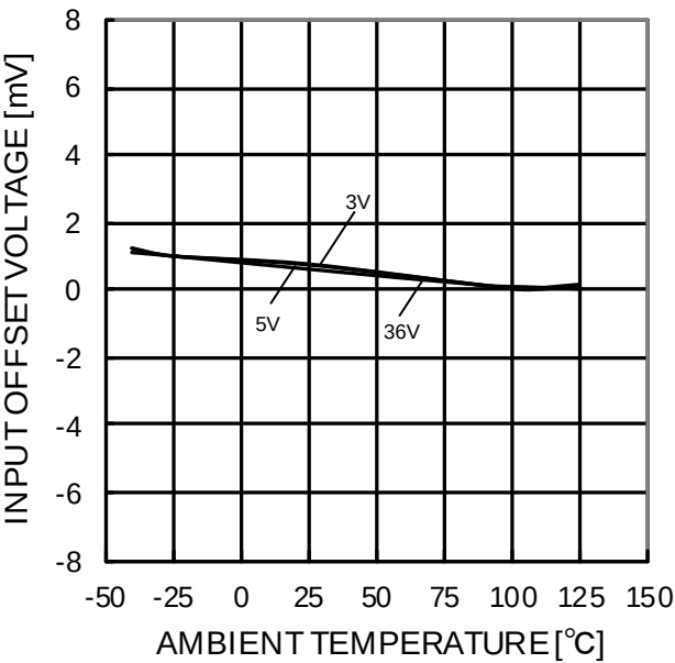
Figure 86. 入力オフセット電圧－温度特性 ( V_{ICM}=0V , OUT=1.4V )
