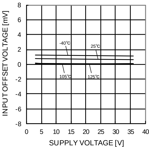
Figure 85. 入力オフセット電圧－電源電圧特性 (V ICM =0V, OUT=1.4V)
