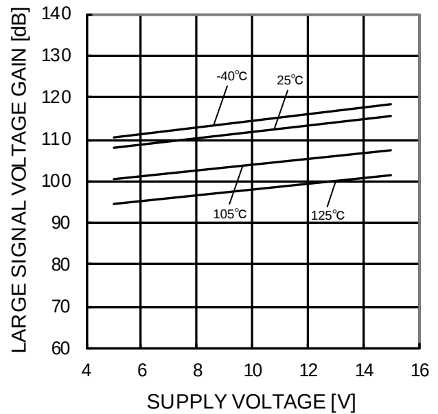
Figure 69. 大振幅電圧利得—電源電圧特性 ( R_L=2k\Omega )
