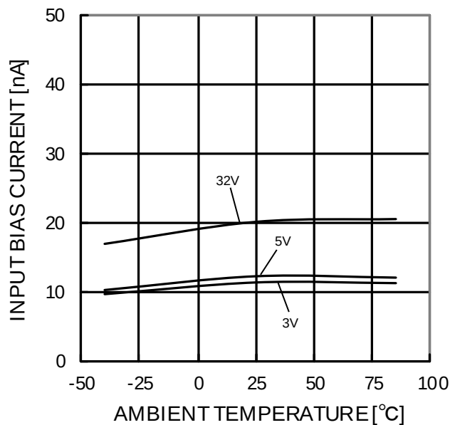
Figure 40. 入力バイアス電流－温度特性 ( V_{ICM}=0V , OUT=1.4V )
