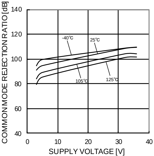
Figure 71. 同相信号除去比－電源電圧特性
