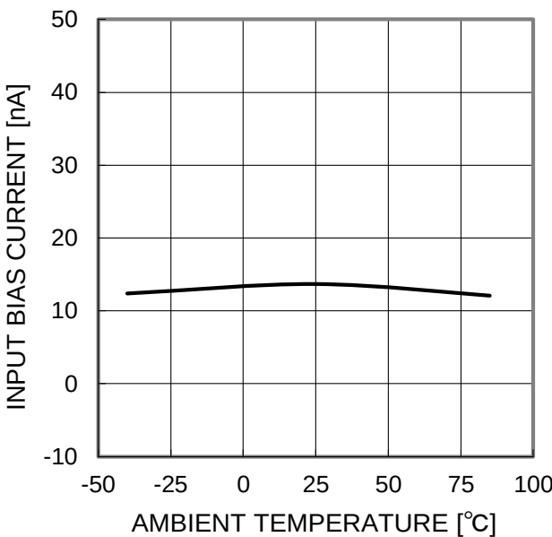
Figure 17. 入力バイアス電流－温度特性 ( V_{CC}=30V , V_{ICM}=28V , OUT=1.4V )
