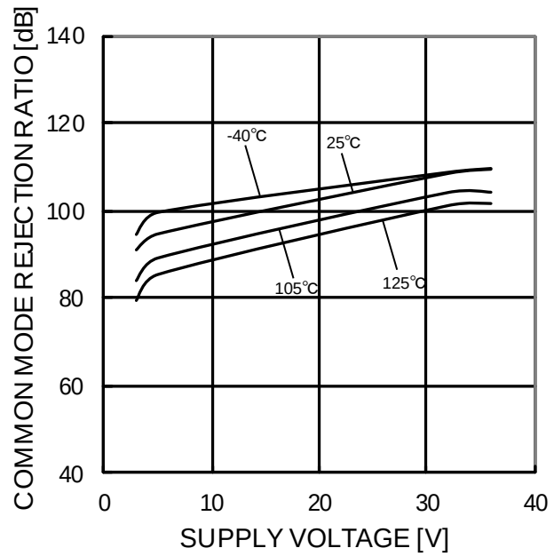
Figure 95. 同相信号除去比－電源電圧特性
