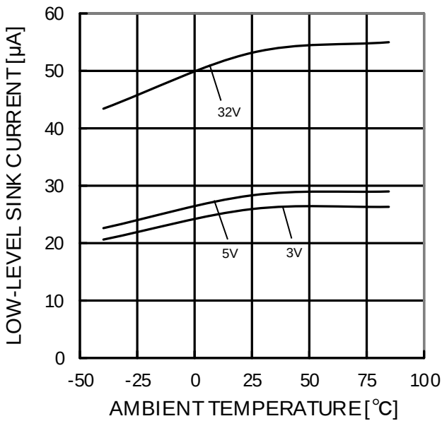
Figure 36. LOW レベルシンク電流－温度特性 (OUT=0.2V)
