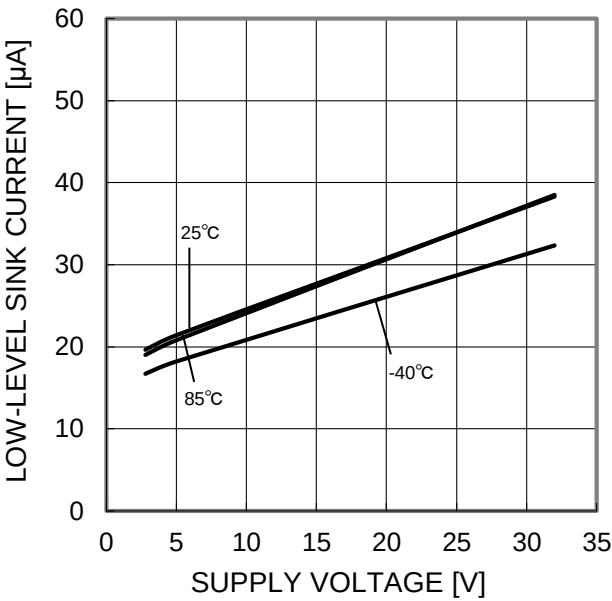
Figure 11. LOW レベルシンク電流－電源電圧特性 (OUT=0.2V)
