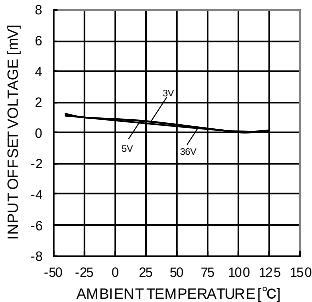
Figure 62. 入力オフセット電圧－温度特性
