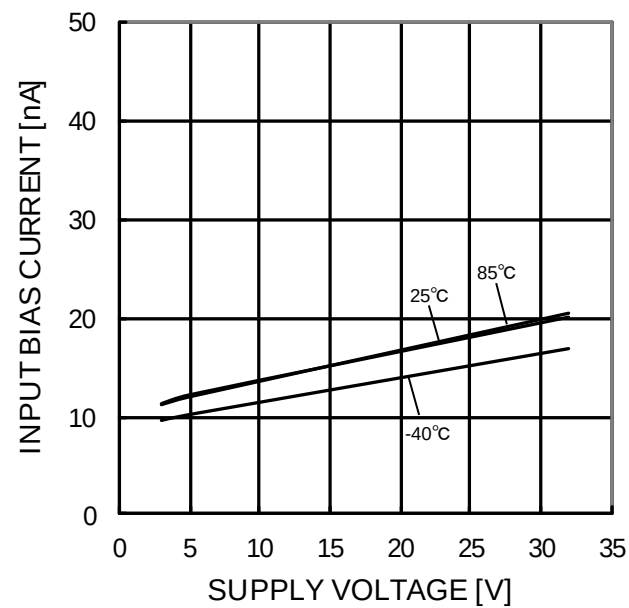
Figure 39. 入力バイアス電流－電源電圧特性 ( V_{ICM}=0V , OUT=1.4V )
