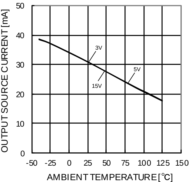
Figure 56. 出力ソース電流－温度特性 (OUT=0V)
