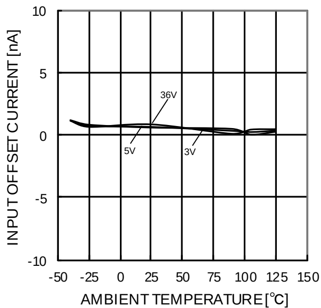
Figure 92. 入力オフセット電流－温度特性 (V ICM =0V, OUT=1.4V)
