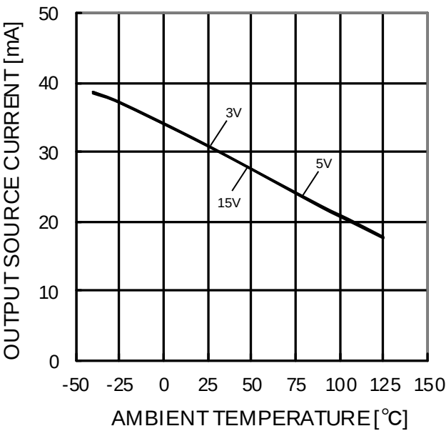
Figure 80. 出力ソース電流－温度特性 (OUT=0V)
