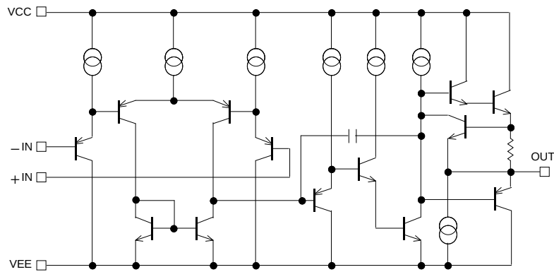
Figure 1. 内部等価回路図（1回路のみ）
