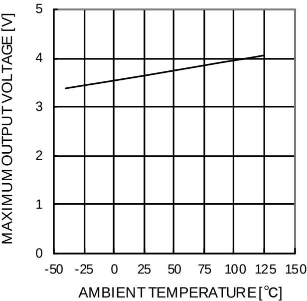
Figure 54. 最大出力電圧－温度特性 (VCC=5V, RL=2kΩ)
