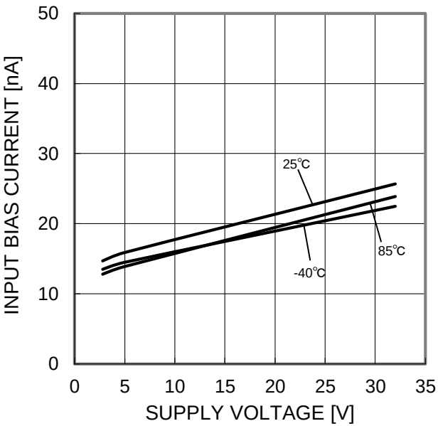
Figure 15. 入力バイアス電流－電源電圧特性 ( V_{ICM}=0V , OUT=1.4V )
