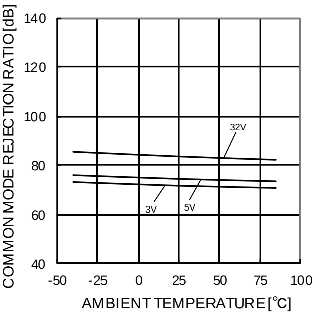
Figure 24. 同相信号除去比－温度特性
