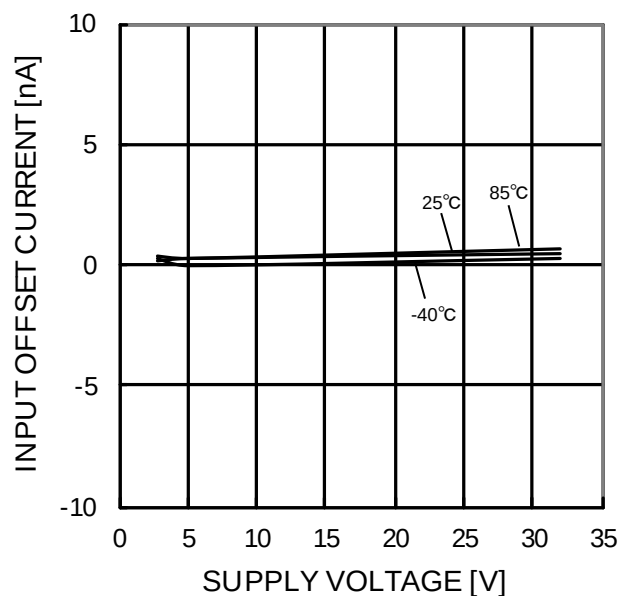
Figure 43. 入力オフセット電流—電源電圧特性 (V ICM =0V, OUT=1.4V)
