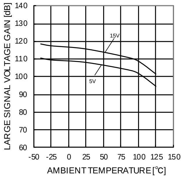
Figure 94. 大振幅電圧利得－温度特性 (RL=2kΩ)
