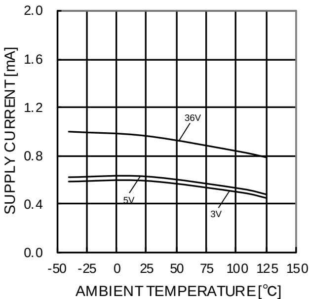
Figure 76. 回路電流－温度特性
