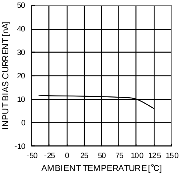
Figure 89. 入力バイアス電流－温度特性 ( V_{CC}=30V , V_{ICM}=28V , OUT=1.4V )
