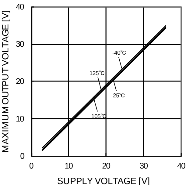
Figure 53. 出力電圧－電源電圧特性 (RL=10kΩ)
