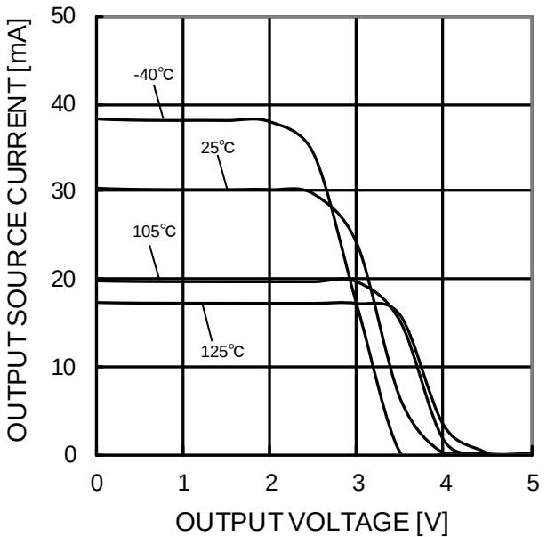
Figure 55. 出力ソース電流－出力電圧特性 (VCC=5V)
