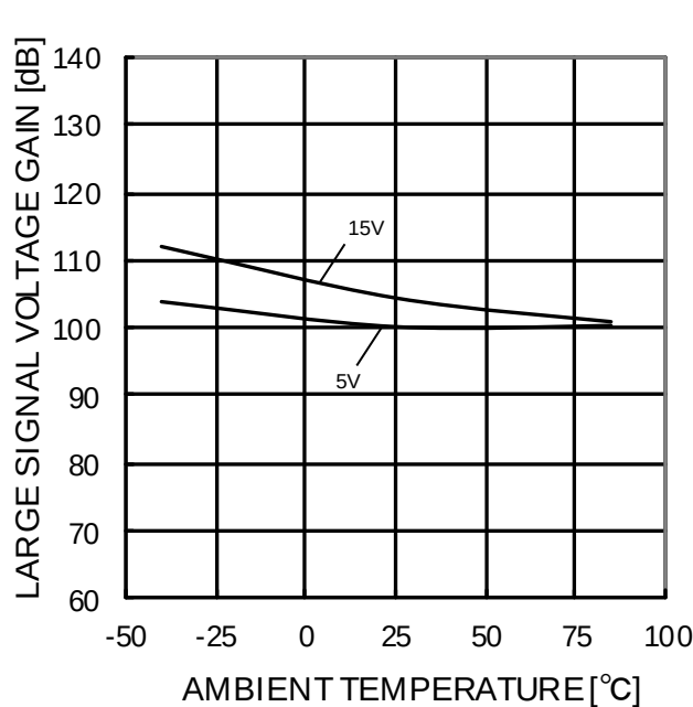
Figure 46. 大振幅電圧利得－温度特性 (RL=2kΩ)
