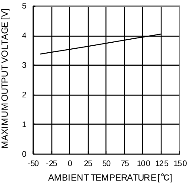
Figure 78. 最大出力電圧－温度特性 (VCC=5V, RL=2kΩ)
