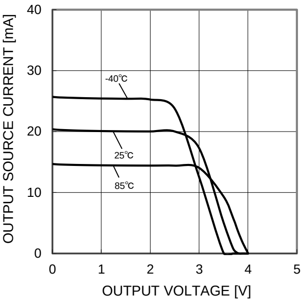
Figure 7. 出力ソース電流－出力電圧特性 (VCC=5V)
