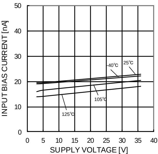
Figure 63. 入力バイアス電流－電源電圧特性 ( V_{ICM}=0V , OUT=1.4V )
