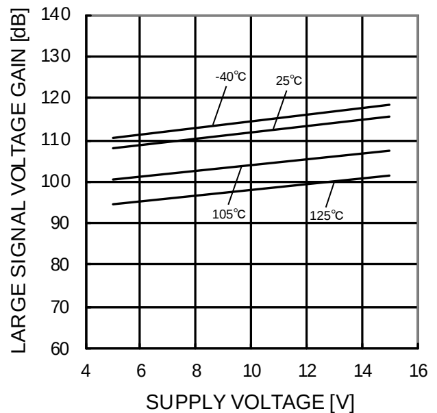
Figure 93. 大振幅電圧利得－電源電圧特性 (R L =2kΩ)
