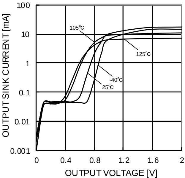
Figure 57. 出力シンク電流－出力電圧特性 (VCC=5V)
