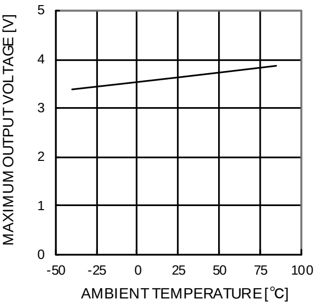
Figure 30. 最大出力電圧－温度特性 (VCC=5V, RL=2kΩ)
