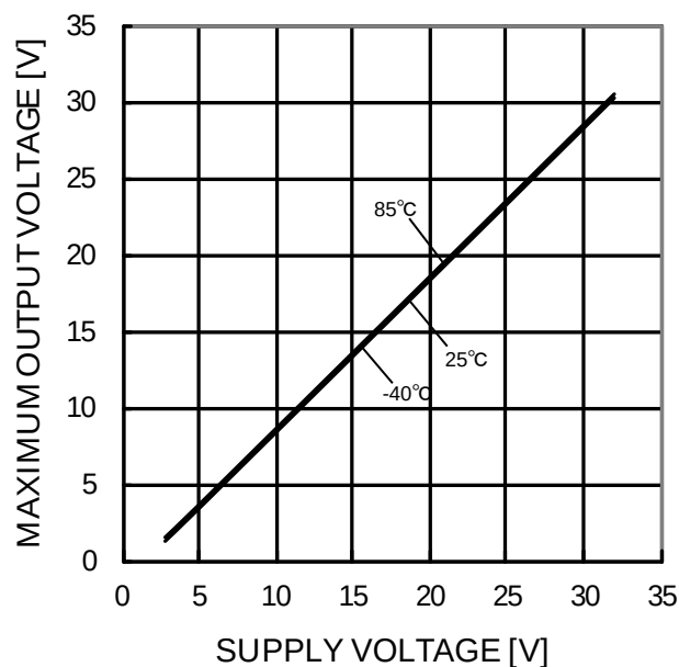
Figure 29. 出力電圧－電源電圧特性 (RL=10kΩ)
