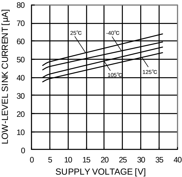
Figure 83. LOW レベルシンク電流－電源電圧特性 (OUT=0.2V)
