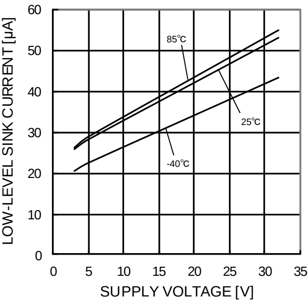
Figure 35. LOW レベルシンク電流－電源電圧特性 (OUT=0.2V)
