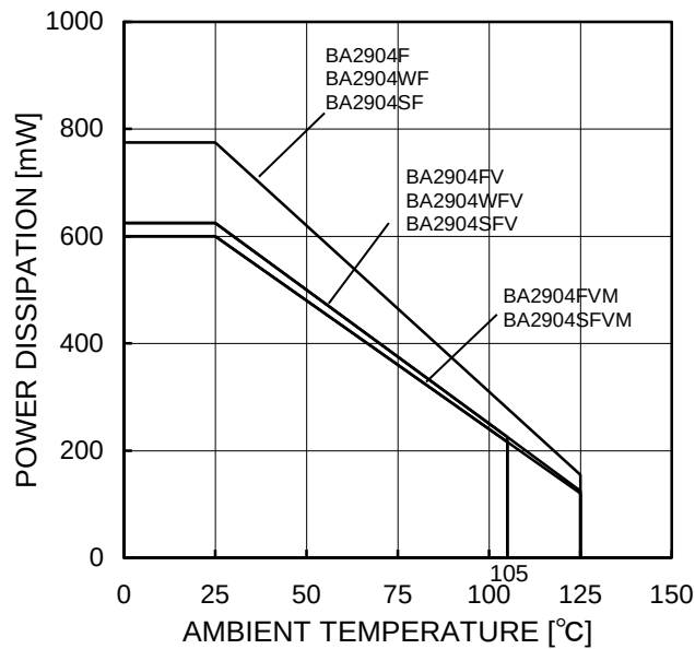
Figure 50. ディレーティングカーブ
