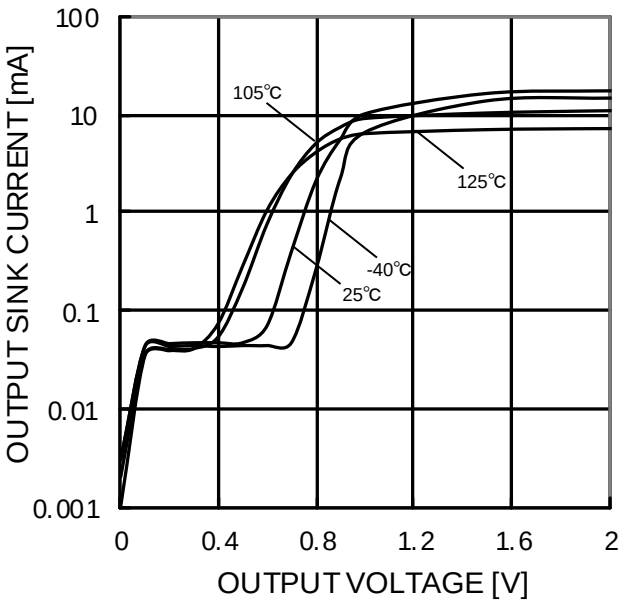
Figure 81. 出力シンク電流－出力電圧特性 (VCC=5V)
