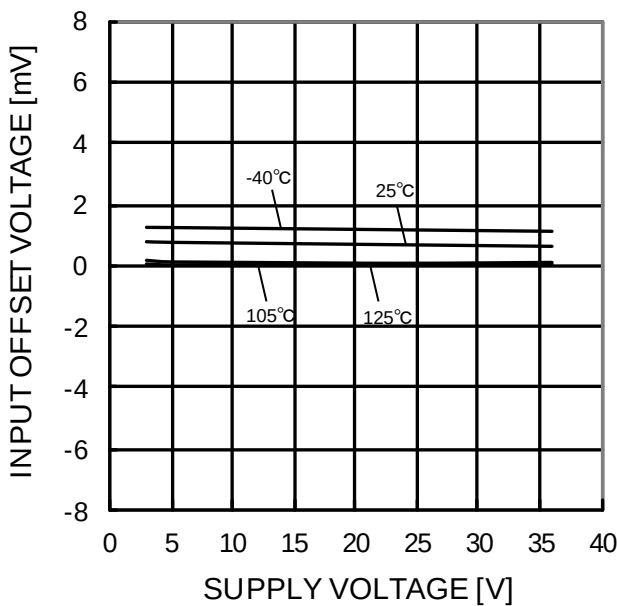
Figure 61. 入力オフセット電圧－電源電圧特性 (V ICM =0V, OUT=1.4V)
