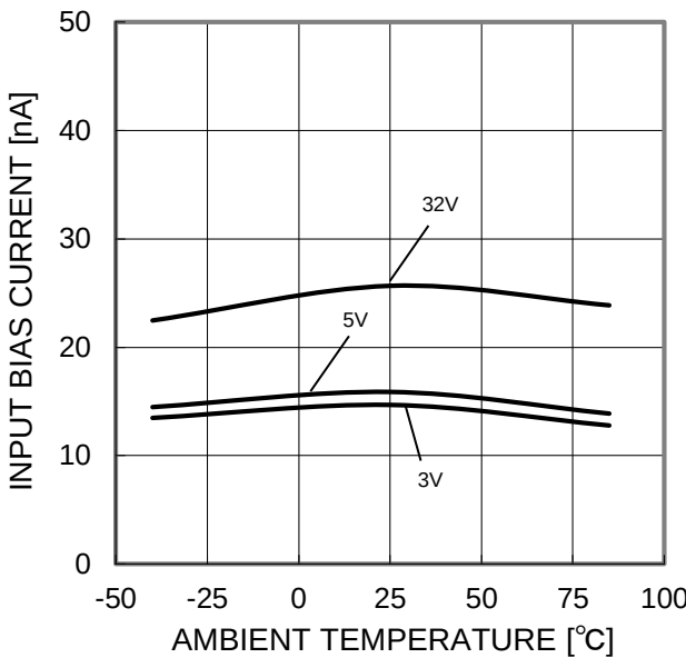
Figure 16. 入力バイアス電流－温度特性 ( V_{ICM}=0V , OUT=1.4V )
