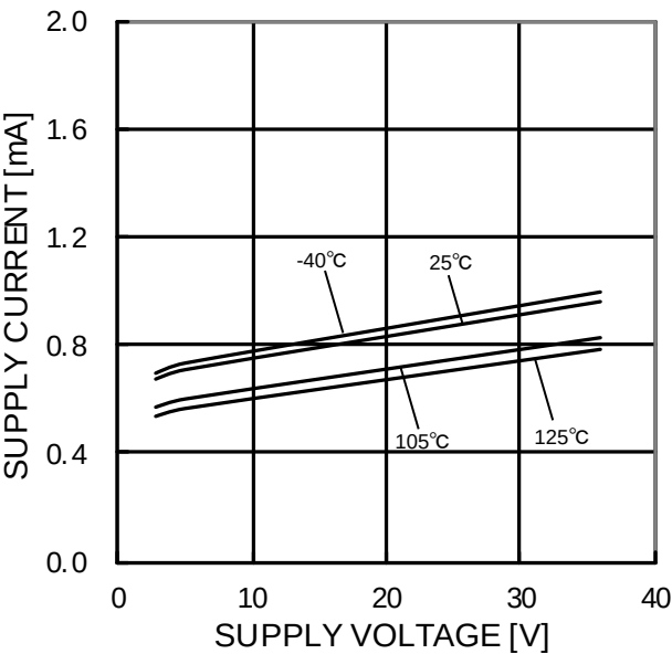
Figure 75. 回路電流－電源電圧特性
