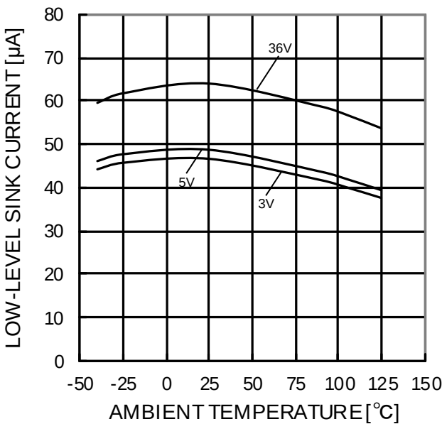
Figure 60. LOW レベルシンク電流－温度特性 (OUT=0.2V)
