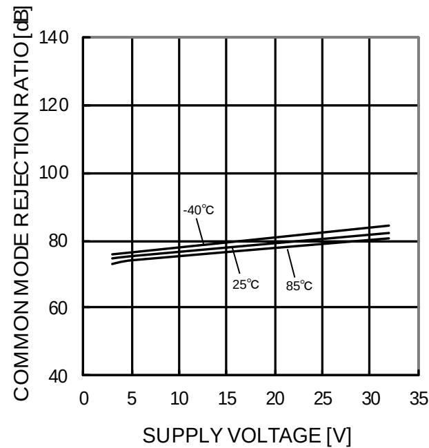
Figure 47. 同相信号除去比－電源電圧特性
