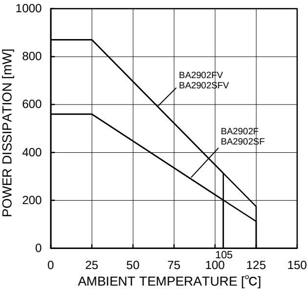
Figure 74. ディレーティングカーブ
