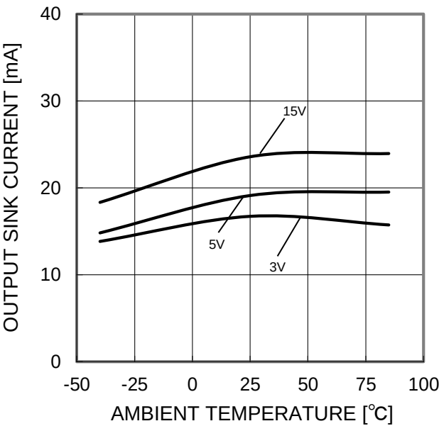
Figure 10. 出力シンク電流－温度特性 (OUT=VCC)
