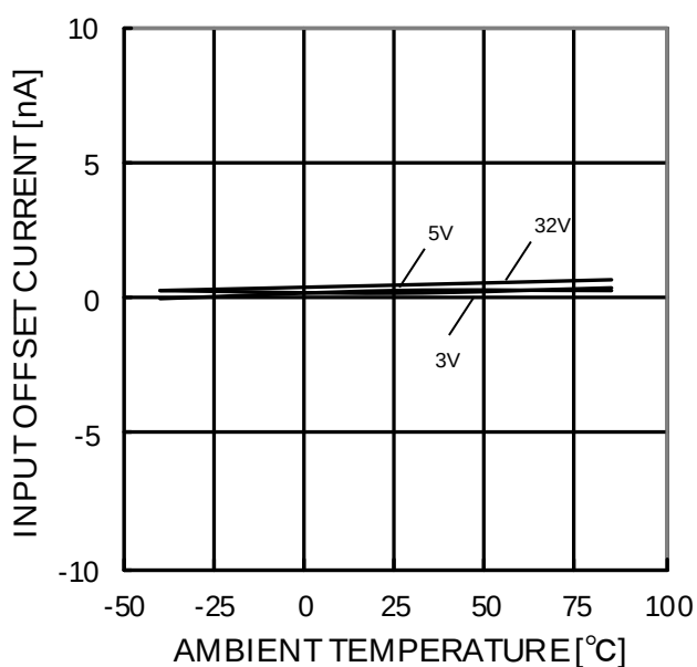
Figure 44. 入力オフセット電流—温度特性 (V ICM =0V, OUT=1.4V)
