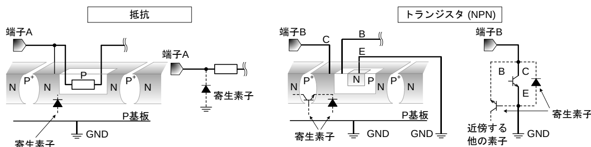
Figure 103. モノリシック IC 構造例
