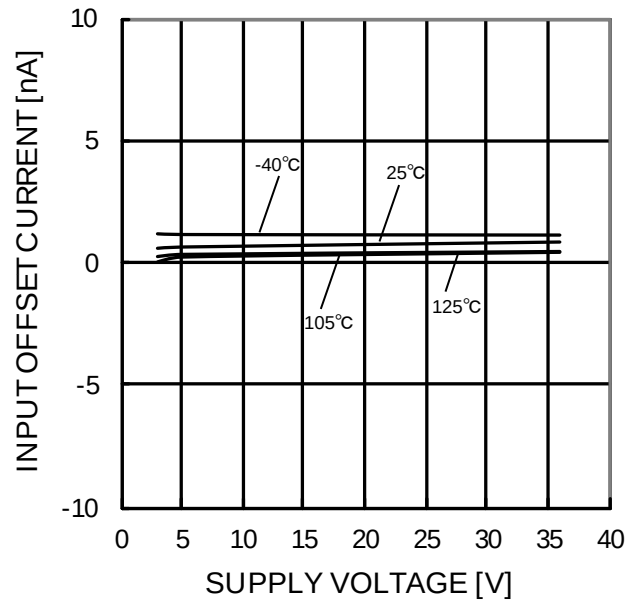
Figure 91. 入力オフセット電流－電源電圧特性 (V ICM =0V, OUT=1.4V)
