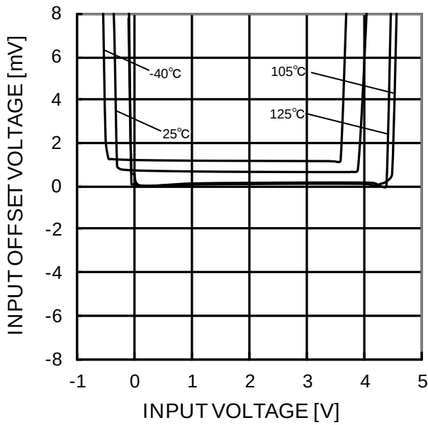
Figure 66. 入力オフセット電圧—同相入力電圧特性 ( V_{CC}=5V )
