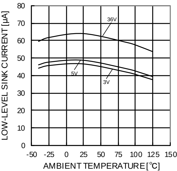
Figure 84. LOW レベルシンク電流－温度特性 (OUT=0.2V)
