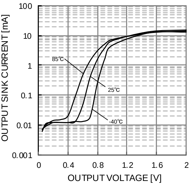
Figure 9. 出力シンク電流－出力電圧特性 (VCC=5V)
