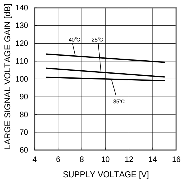
Figure 21. 大振幅電圧利得－電源電圧特性 (R L =2kΩ)
