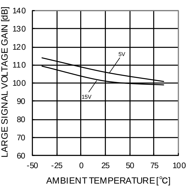
Figure 22. 大振幅電圧利得－温度特性 (RL=2kΩ)
