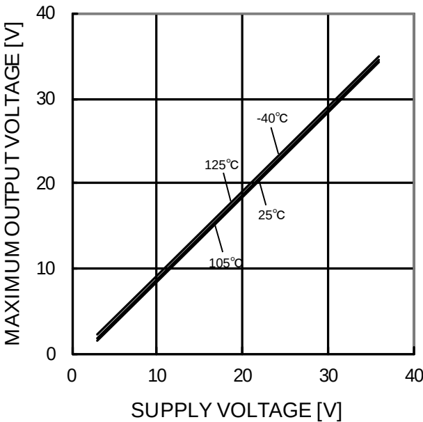
Figure 77. 出力電圧－電源電圧特性 (RL=10kΩ)
