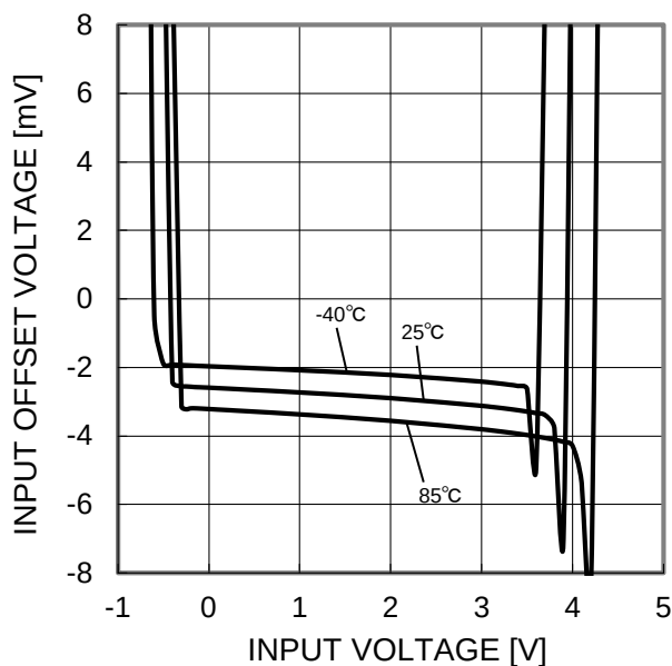
Figure 18. 入力オフセット電圧－同相入力電圧特性 (VCC=5V)
