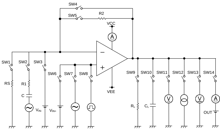
Figure 99. 測定回路 2 (片チャンネルのみ)
