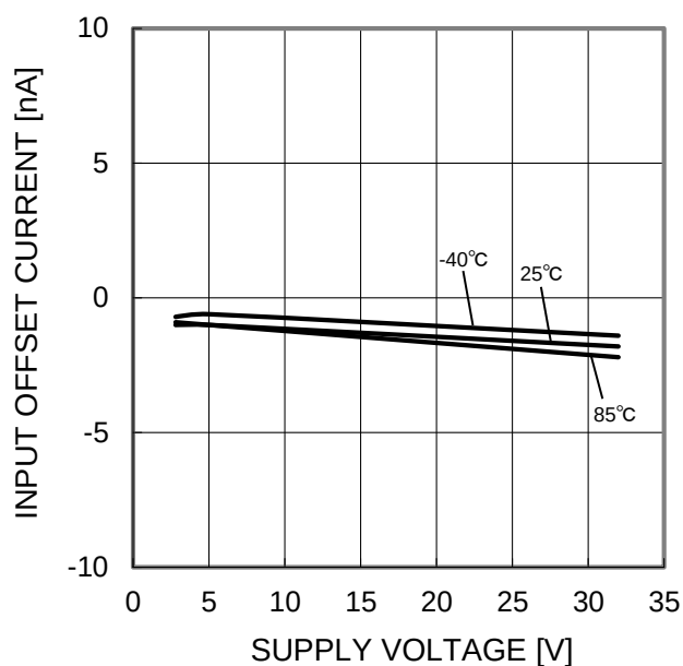
Figure 19. 入力オフセット電流－電源電圧特性 (V ICM =0V, OUT=1.4V)
