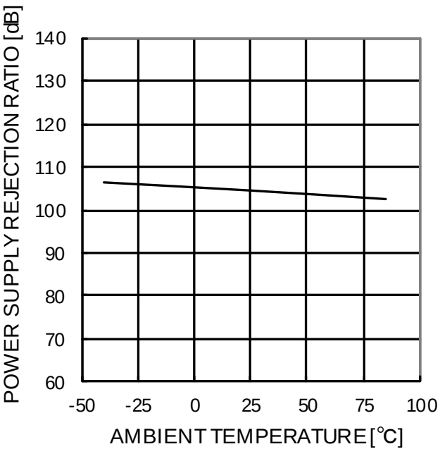
Figure 25. 電源電圧除去比－温度特性
