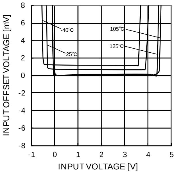
Figure 90. 入力オフセット電圧－同相入力電圧特性 (VCC=5V)
