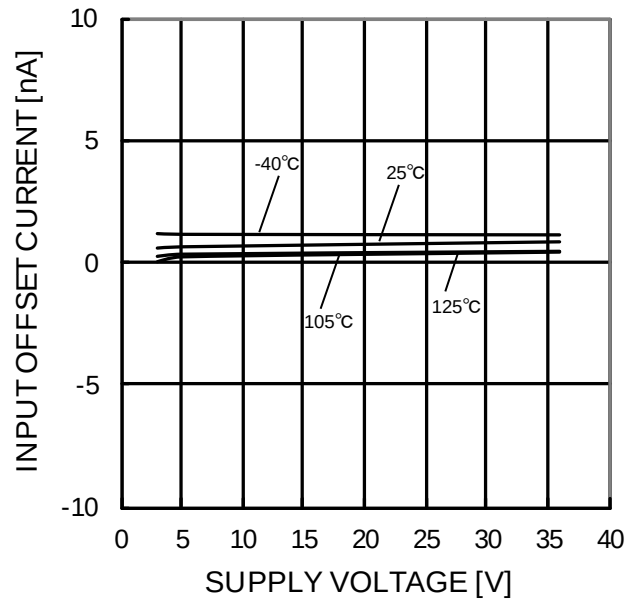
Figure 67. 入力オフセット電流—電源電圧特性 ( V_{ICM}=0V , OUT=1.4V )
