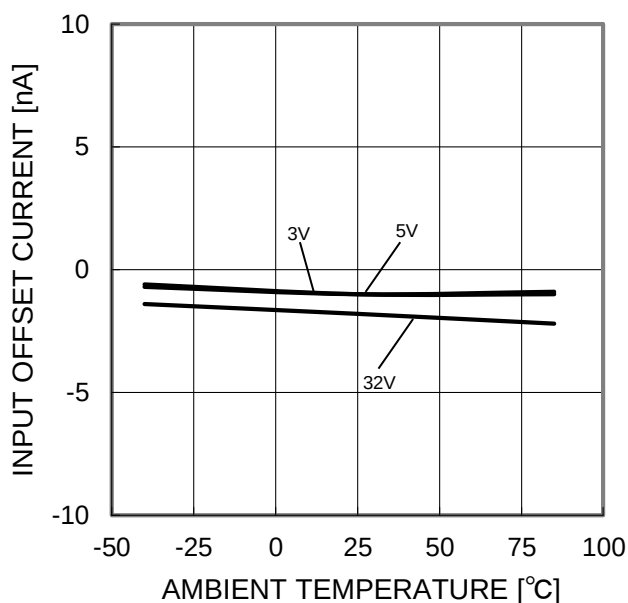
Figure 20. 入力オフセット電流－温度特性 (V ICM =0V, OUT=1.4V)
