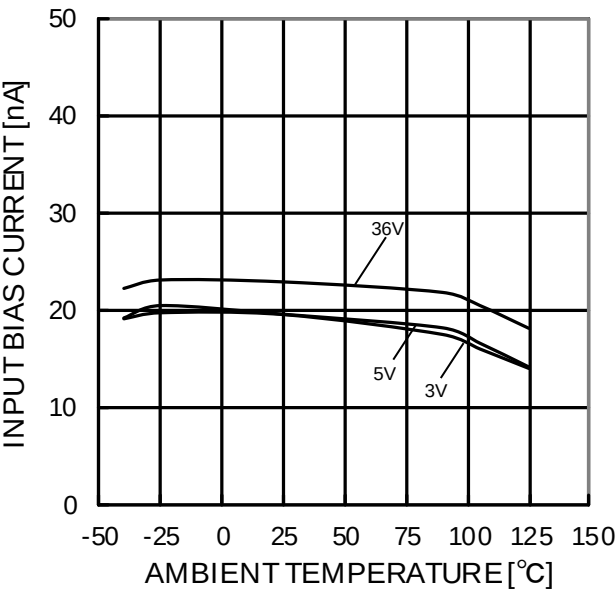
Figure 88. 入力バイアス電流－温度特性 ( V_{ICM}=0V , OUT=1.4V )
