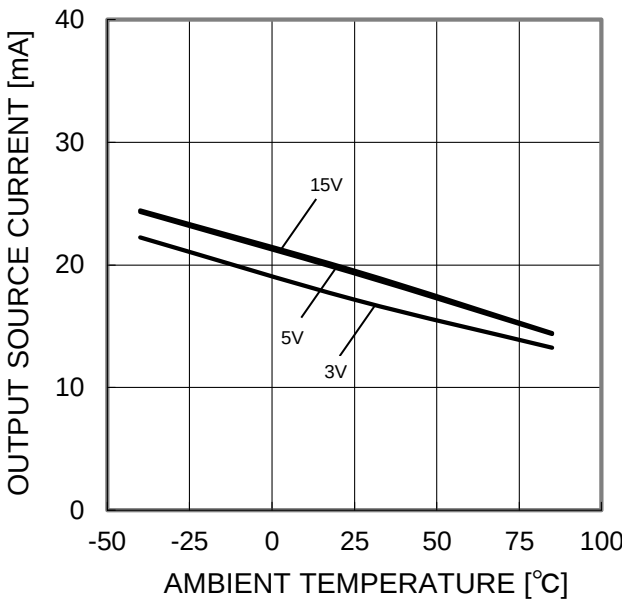
Figure 8. 出力ソース電流－温度特性 (OUT=0V)
