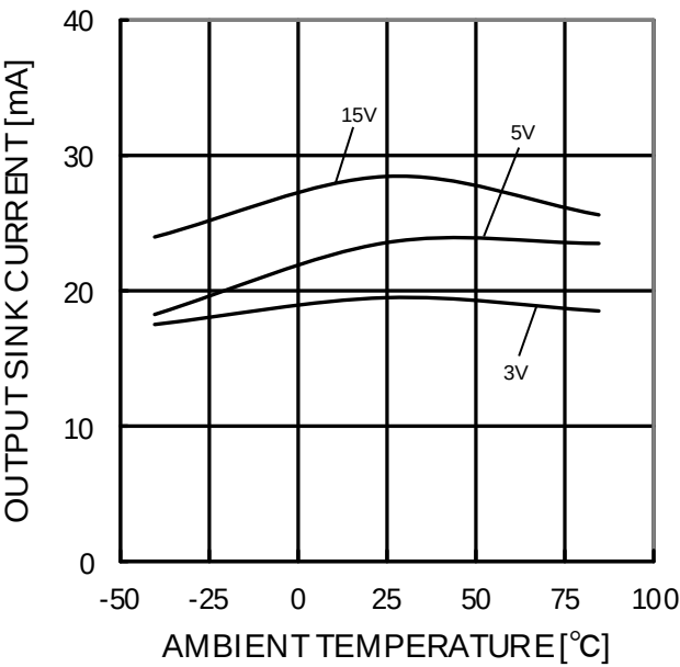
Figure 34. 出力シンク電流－温度特性 (OUT=VCC)
