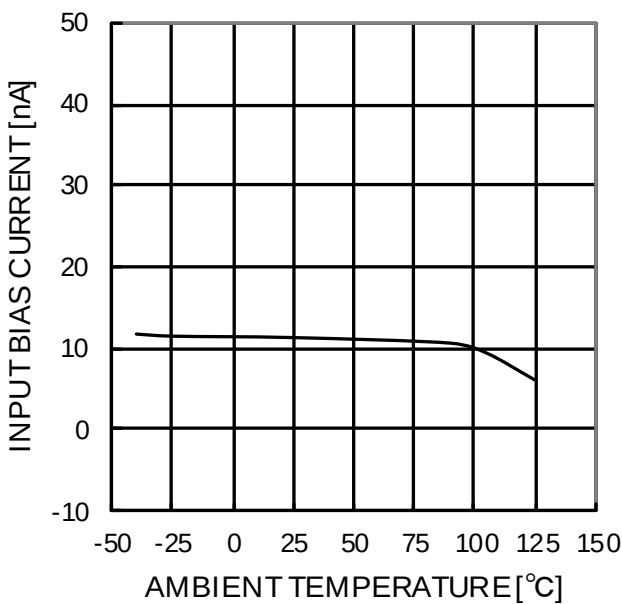
Figure 65. 入力バイアス電流－温度特性 ( VCC=30V , V_{ICM}=28V , OUT=1.4V )
