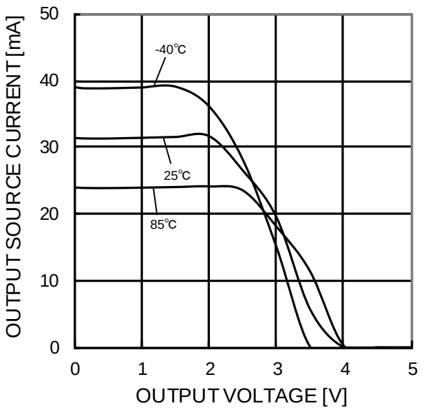
Figure 31. 出力ソース電流－出力電圧特性 (VCC=5V)
