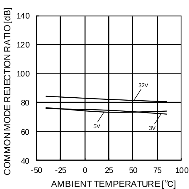
Figure 48. 同相信号除去比－温度特性
