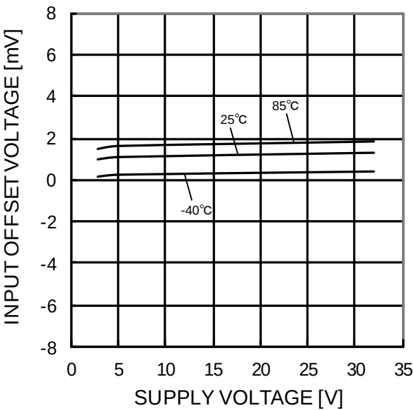
Figure 37. 入力オフセット電圧－電源電圧特性 (V ICM =0V, OUT=1.4V)
