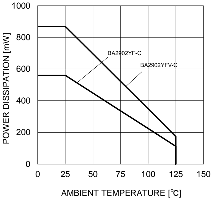
Figure 26. ディレーティングカーブ
