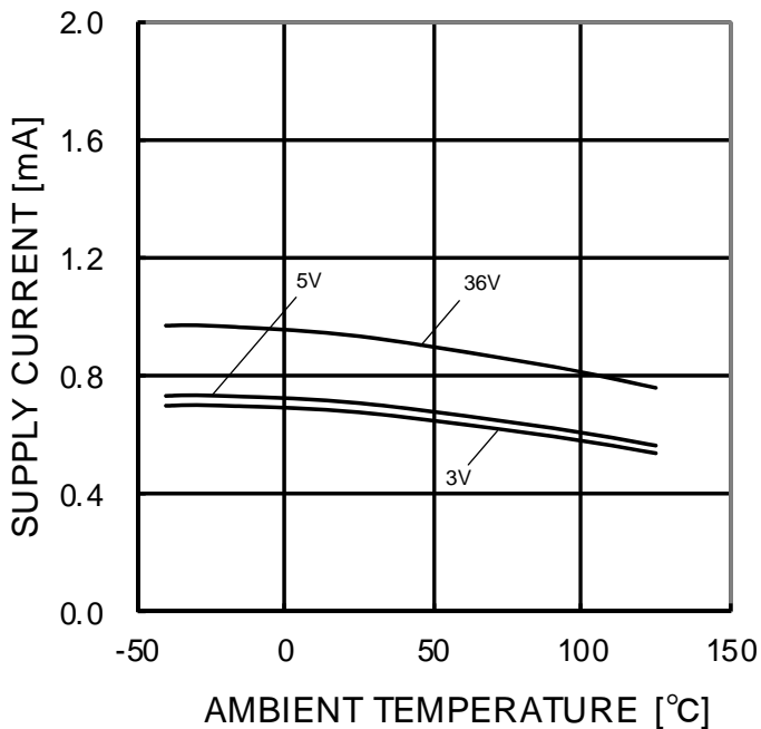
Figure 28. 回路電流－温度特性
