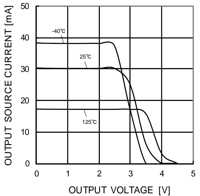
Figure 7. 出力ソース電流－出力電圧特性 (VCC=5V)
