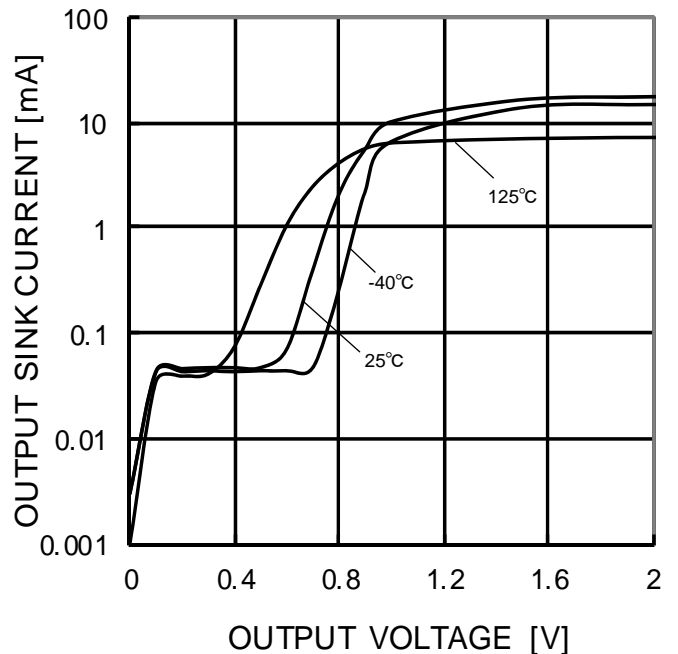
Figure 9. 出力シンク電流－出力電圧特性 (VCC=5V)
