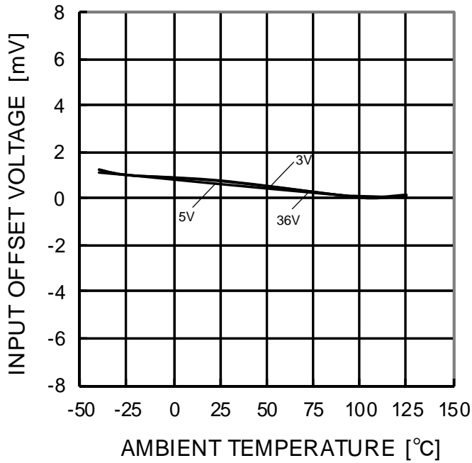
Figure 38. 入力オフセット電圧－温度特性 (Vicm=0V, OUT=1.4V)
