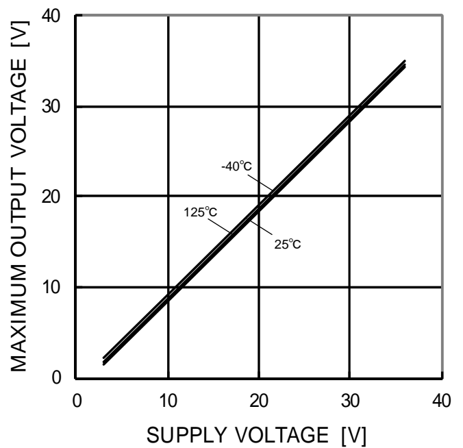
Figure 29. 出力電圧－電源電圧特性 (RL=10kΩ)
