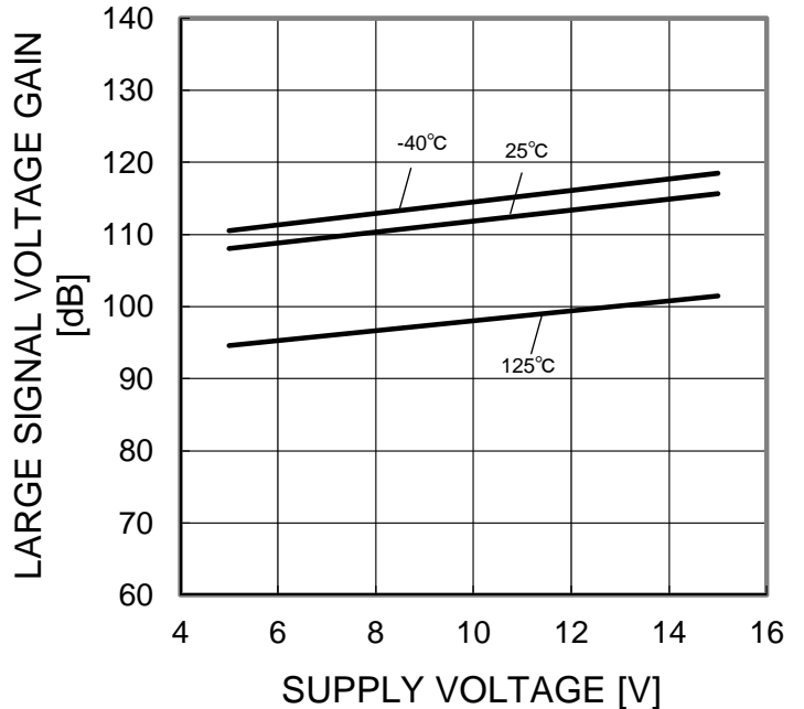
Figure 45. 大振幅電圧利得—電源電圧特性 (RL=2kΩ)
