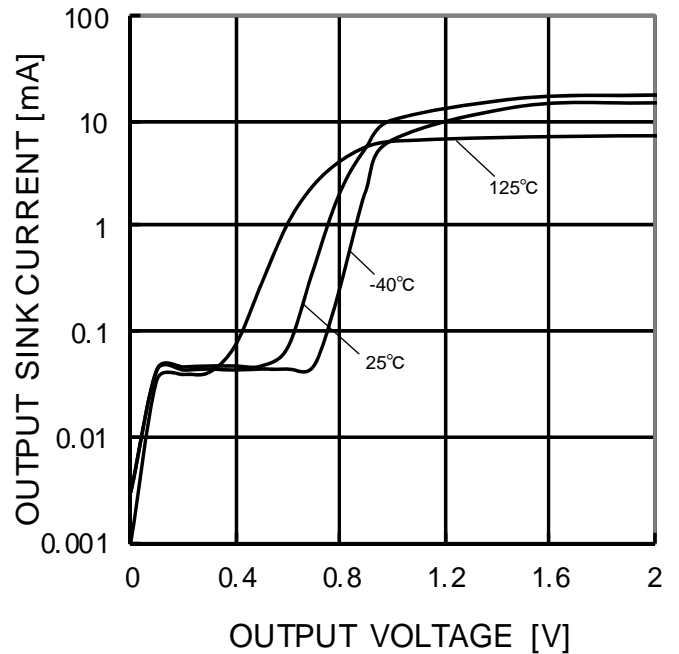
Figure 33. 出力シンク電流－出力電圧特性 (VCC=5V)
