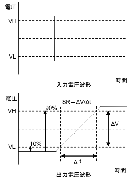
Figure 54. スルーレート測定時 入出力波形
