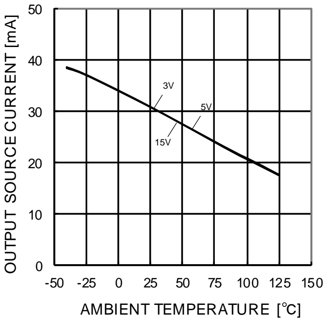
Figure 32. 出力ソース電流－温度特性 (OUT=0V)
