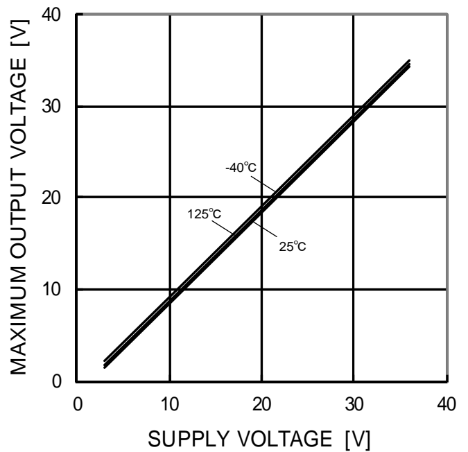
Figure 5. 出力電圧—電源電圧特性 (RL=10kΩ)
