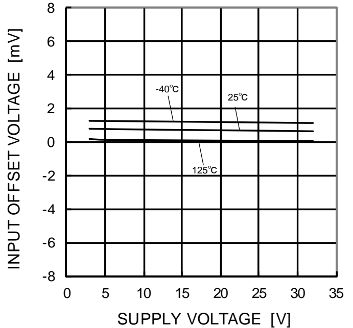
Figure 37. 入力オフセット電圧－電源電圧特性 (Vicm=0V, OUT=1.4V)
