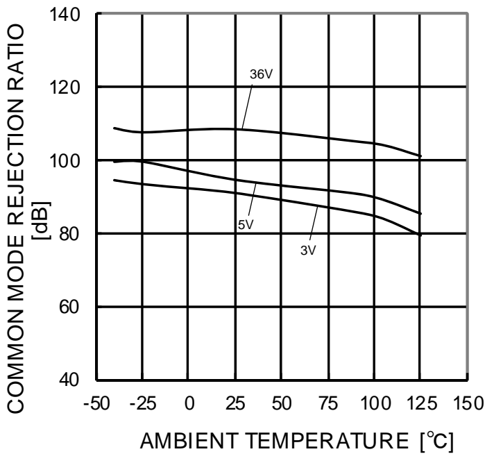
Figure 24. 同相信号除去比－温度特性
