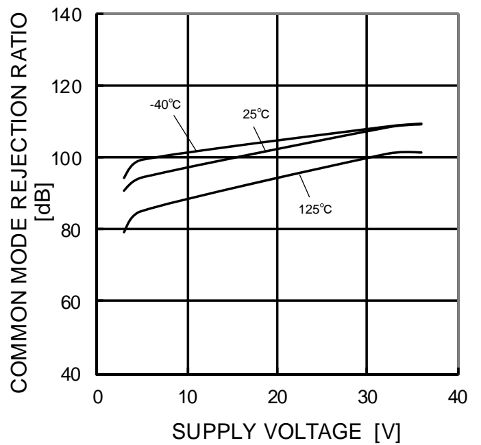
Figure 47. 同相信号除去比－電源電圧特性
