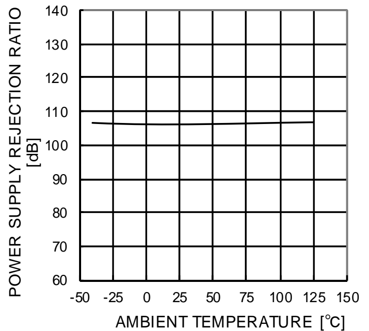
Figure 25 電源電圧除去比－温度特性
