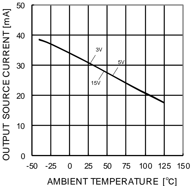
Figure 8. 出力ソース電流－温度特性 (OUT=0V)
