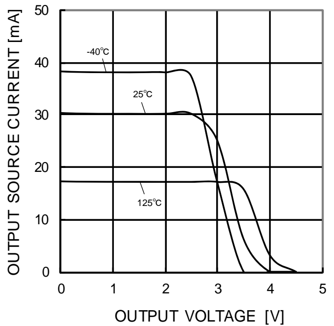
Figure 31. 出力ソース電流－出力電圧特性 (VCC=5V)
