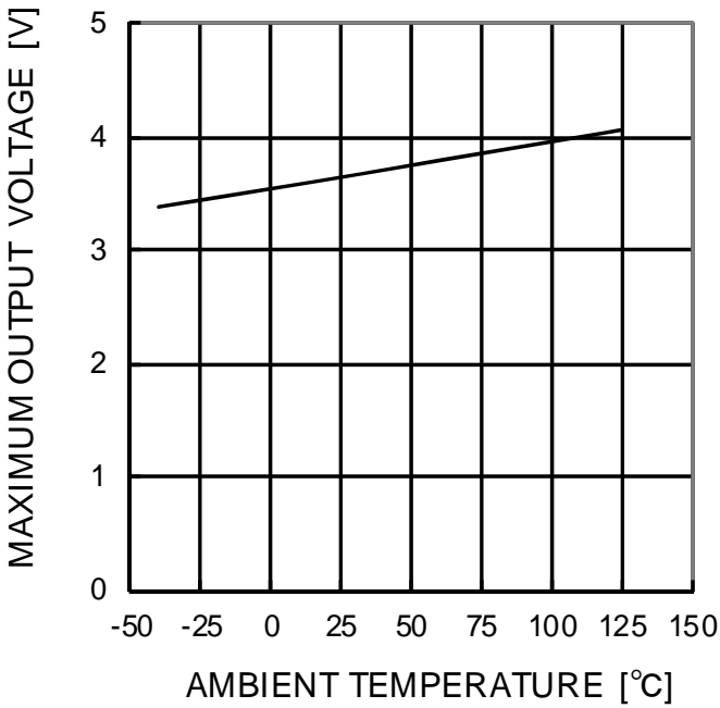
Figure 30. 最大出力電圧－温度特性 (VCC=5V, RL=2kΩ)
