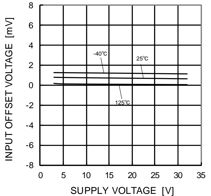
Figure 13. 入力オフセット電圧－電源電圧特性 (Vicm=0V, OUT=1.4V)
