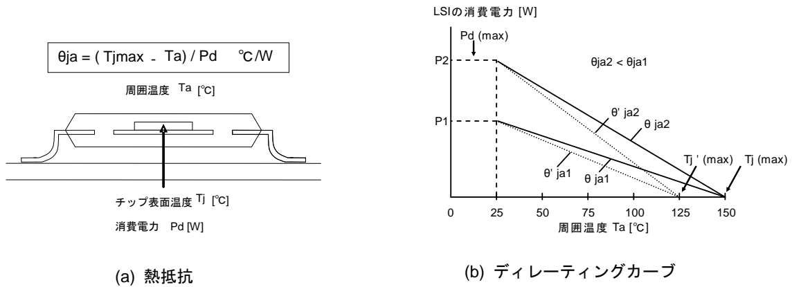
Figure 50. 熱抵抗とディレーティングカーブ
