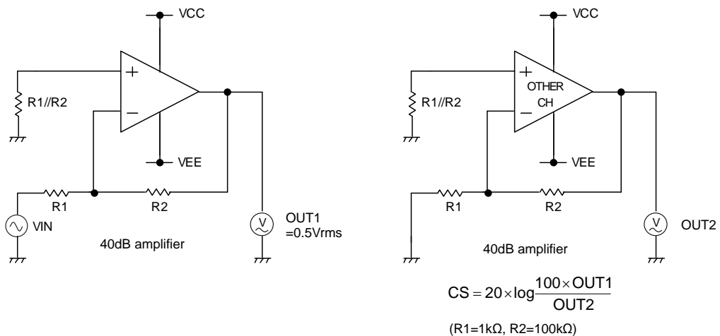
Figure 55. 測定回路 3 (チャンネルセパレーション)
