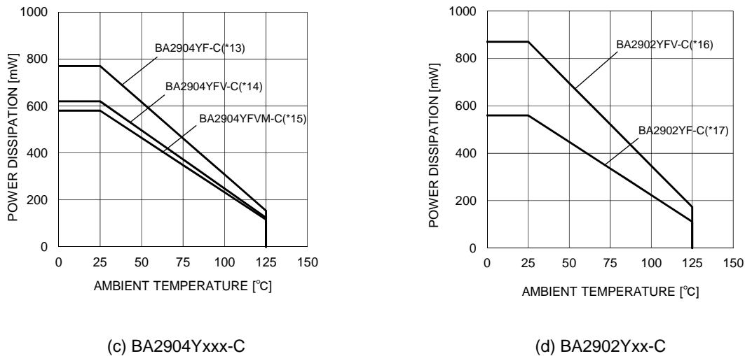
Figure 50. 熱抵抗とディレーティングカーブ
