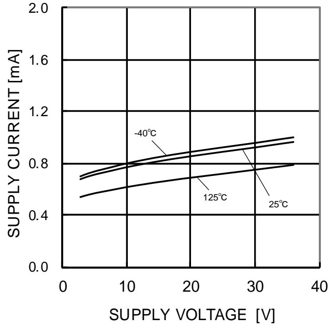
Figure 27. 回路電流－電源電圧特性
