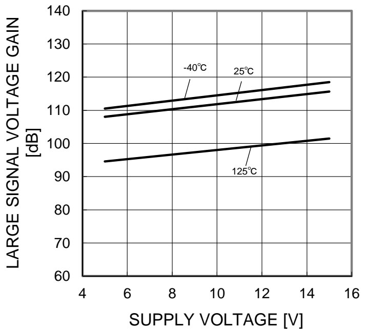
Figure 21. 大振幅電圧利得—電源電圧特性 (RL=2kΩ)
