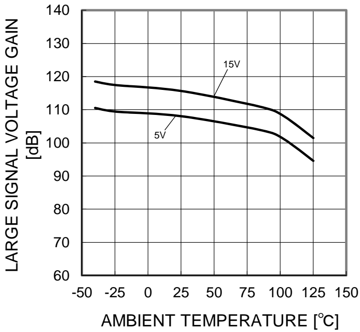
Figure 46. 大振幅電圧利得－温度特性 (RL=2kΩ)
