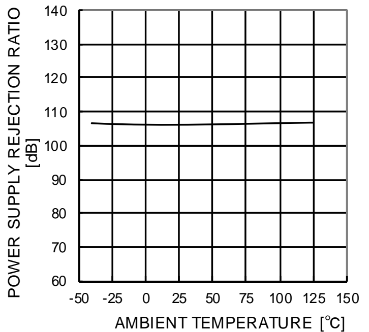
Figure 49. 電源電圧除去比－温度特性
