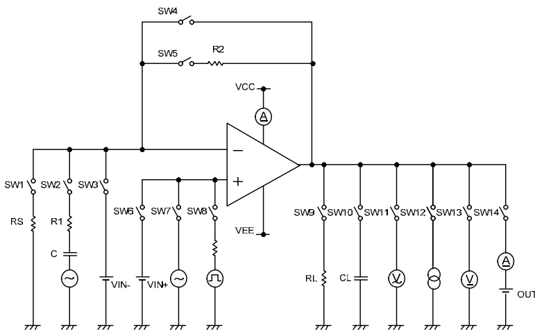
Figure 53. 測定回路 2 (片チャンネルのみ)
