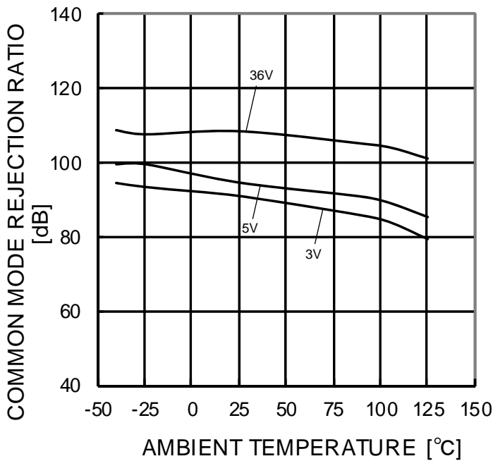
Figure 48. 同相信号除去比－温度特性
