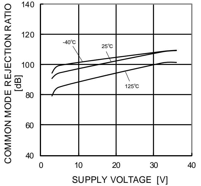
Figure 23. 同相信号除去比－電源電圧特性
