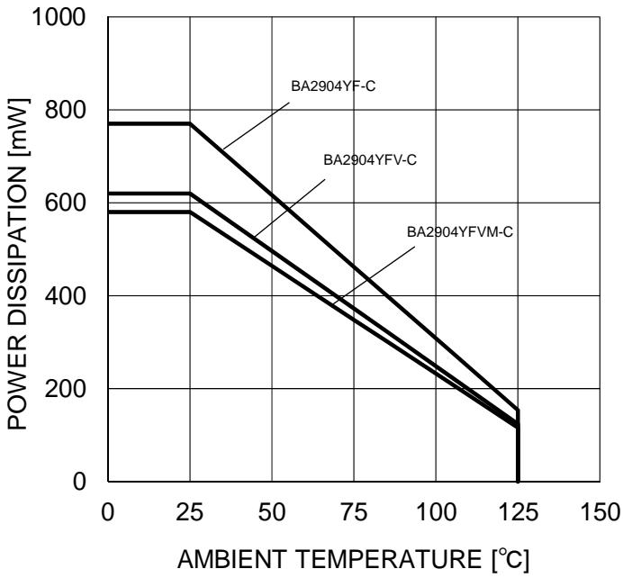
Figure 2. ディレーティングカーブ
