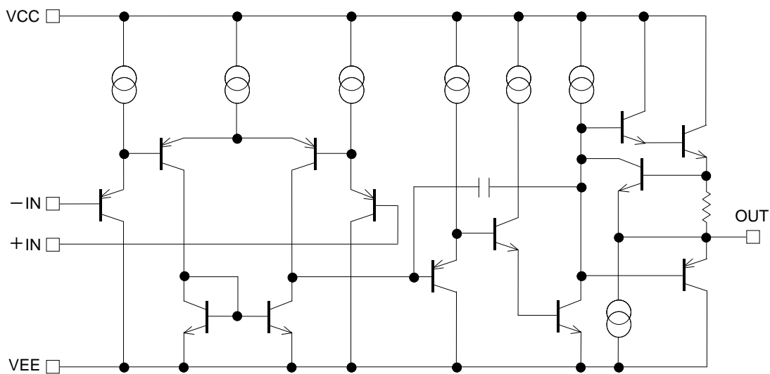
Figure 1. 内部等価回路図 (1回路のみ)
