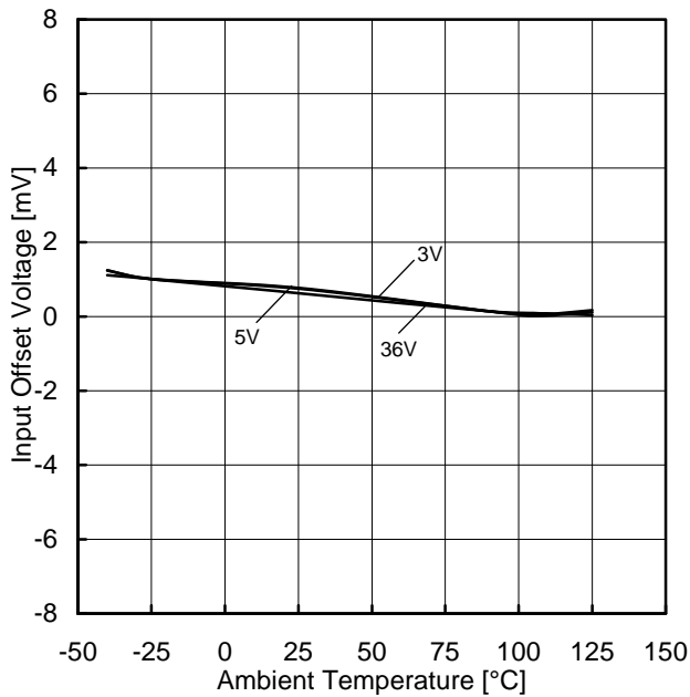
Figure 14. 入力オフセット電圧-温度特性 ( V_{ICM}=0V , E_K=-1.4V )
