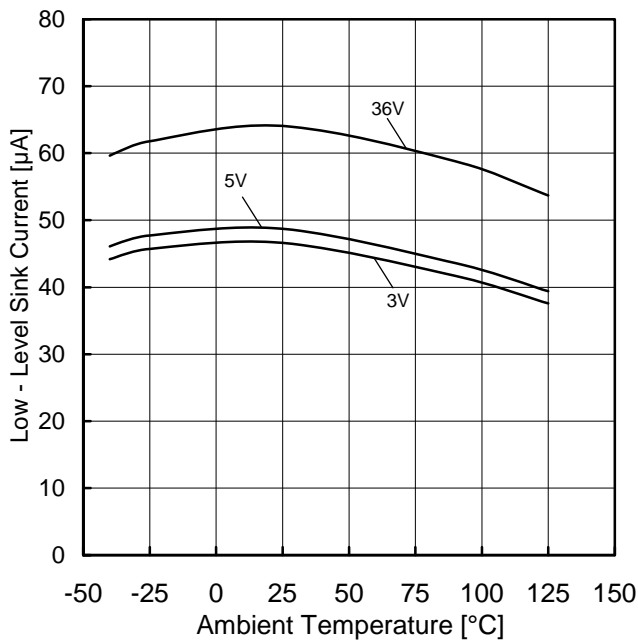
Figure 36. LOW レベルシンク電流－温度特性 (OUT=0.2V)
