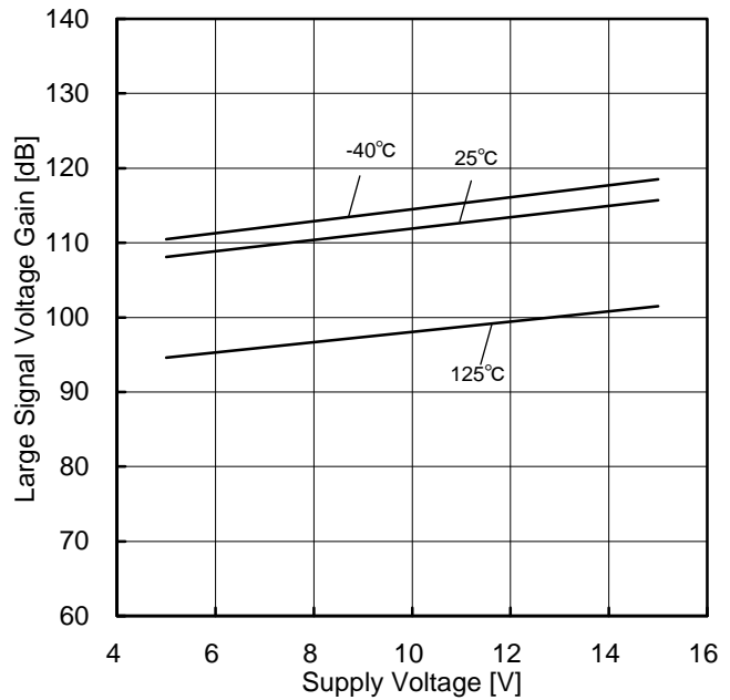
Figure 45. 大振幅電圧利得—電源電圧特性 (RL=2kΩ)
