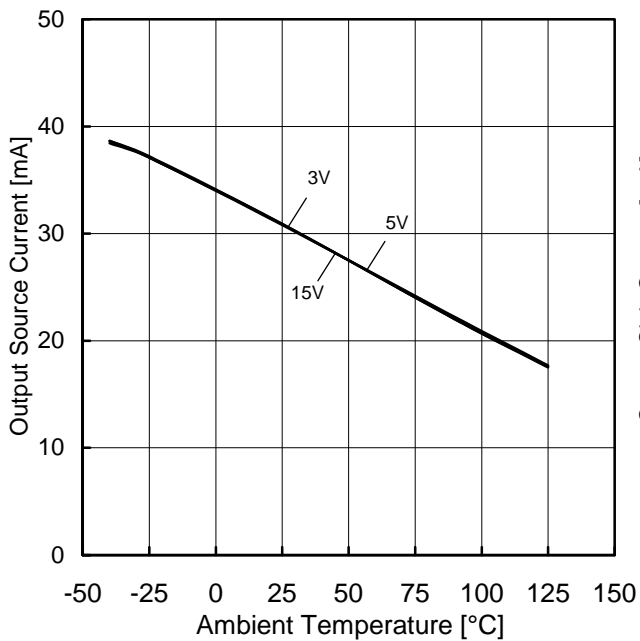
Figure 32. 出カソース電流－温度特性 (OUT=0V)
