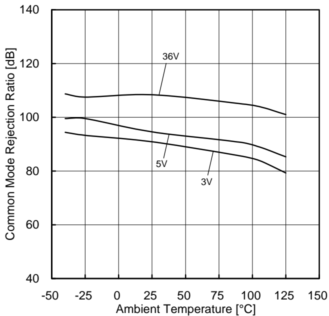
Figure 24. 同相信号除去比-温度特性
