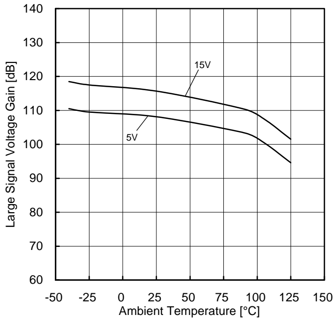
Figure 46. 大振幅電圧利得-温度特性 ( R_L=2k\Omega )
