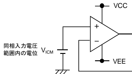
Figure 56. 未使用回路の処理例
