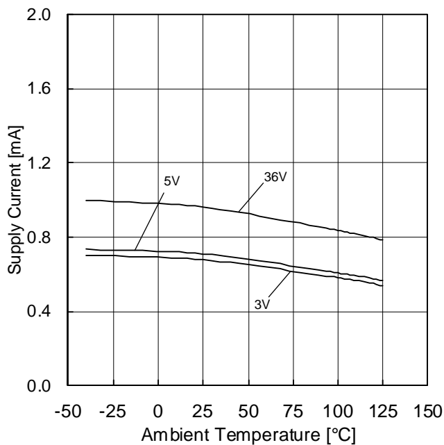
Figure 28. 回路電流－温度特性
