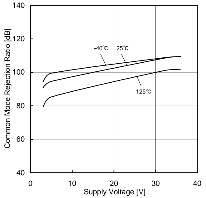
Figure 47. 同相信号除去比-電源電圧特性
