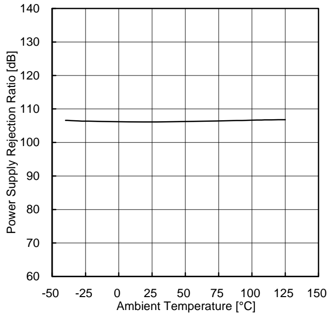
Figure 49. 電源電圧除去比-温度特性
