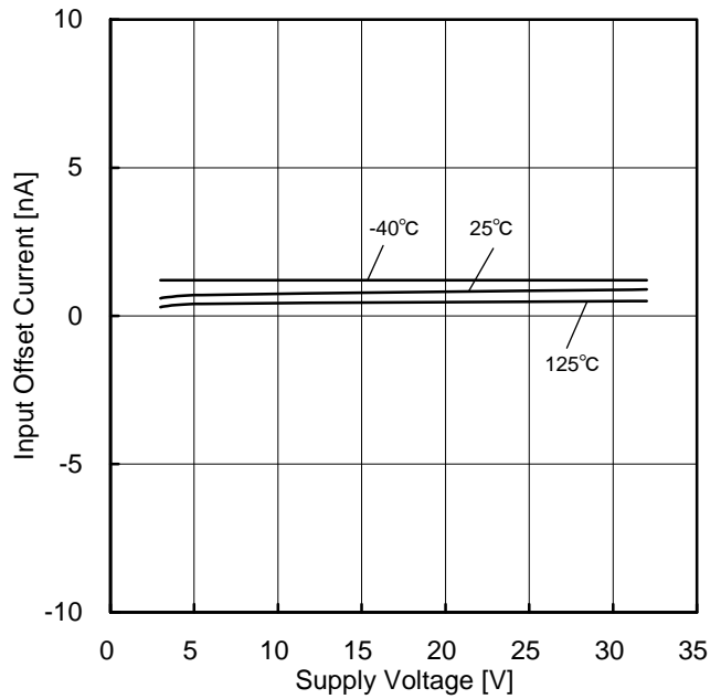
Figure 19. 入力オフセット電流—電源電圧特性 (V ICM =0V, E K =-1.4V)
