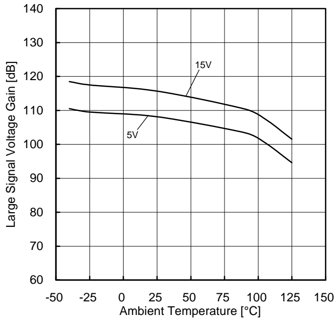
Figure 22. 大振幅電圧利得-温度特性 ( R_L=2k\Omega )
