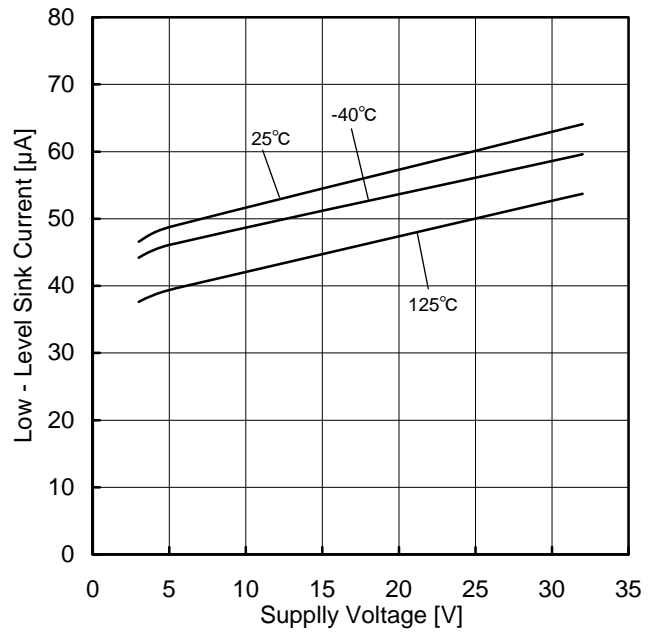
Figure 11. LOW レベルシンク電流－電源電圧特性 (OUT=0.2V)
