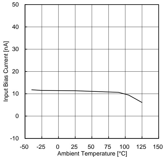
Figure 41. 入力バイアス電流－温度特性 ( V_{CC}=30V , V_{ICM}=28V , E_K=-1.4V )
