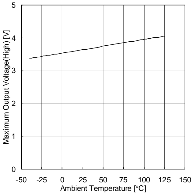
Figure 30. 最大出力電圧(High)－温度特性 (VCC=5V, R L =2kΩ)
