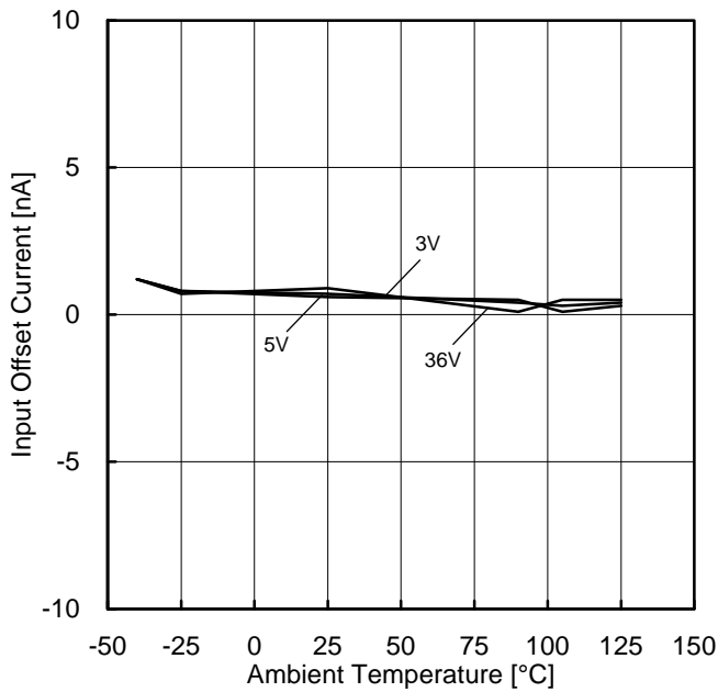
Figure 44. 入力オフセット電流—温度特性 (VICM=0V, EK=-1.4V)
