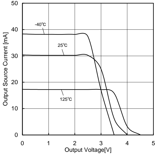
Figure 7. 出カソース電流－出力電圧特性 (VCC=5V)
