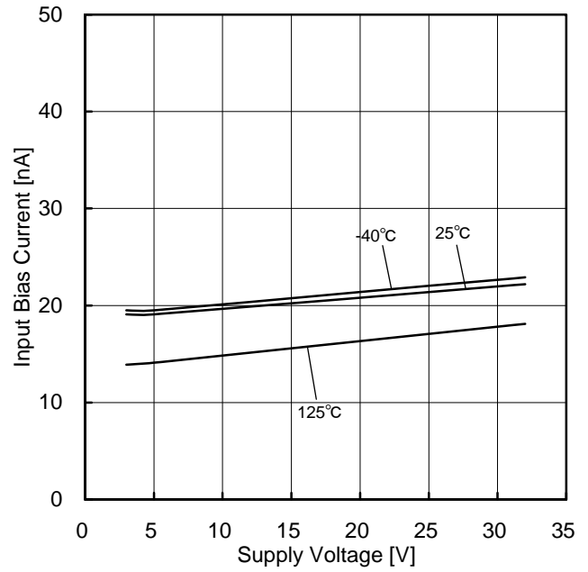
Figure 39. 入力バイアス電流－電源電圧特性 ( V_{ICM}=0V , E_K=-1.4V )
