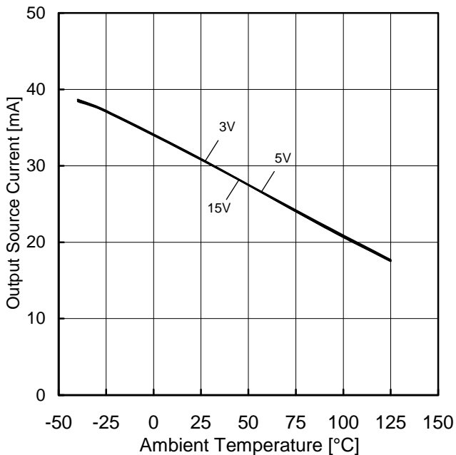
Figure 8. 出カソース電流－温度特性 (OUT=0V)
