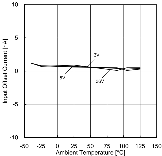
Figure 20. 入力オフセット電流—温度特性 (V ICM =0V, E K =-1.4V)
