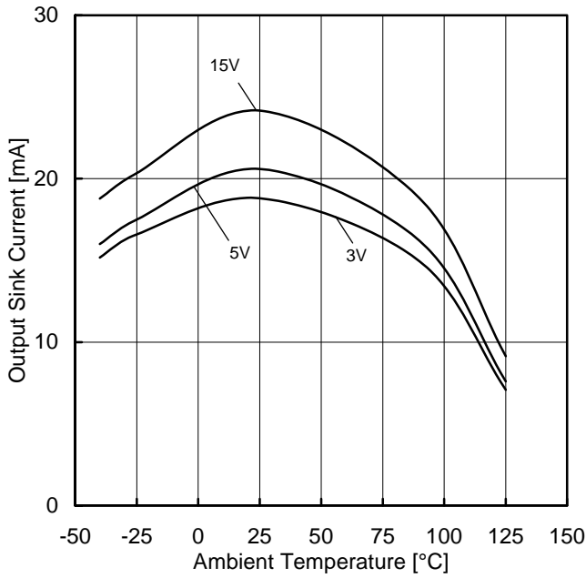
Figure 34. 出力シンク電流－温度特性 (OUT=VCC)
