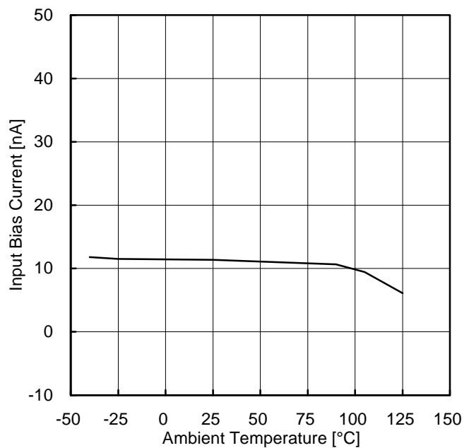
Figure 17. 入力バイアス電流-温度特性 ( V_{CC}=30V , V_{ICM}=28V , E_K=-1.4V )
