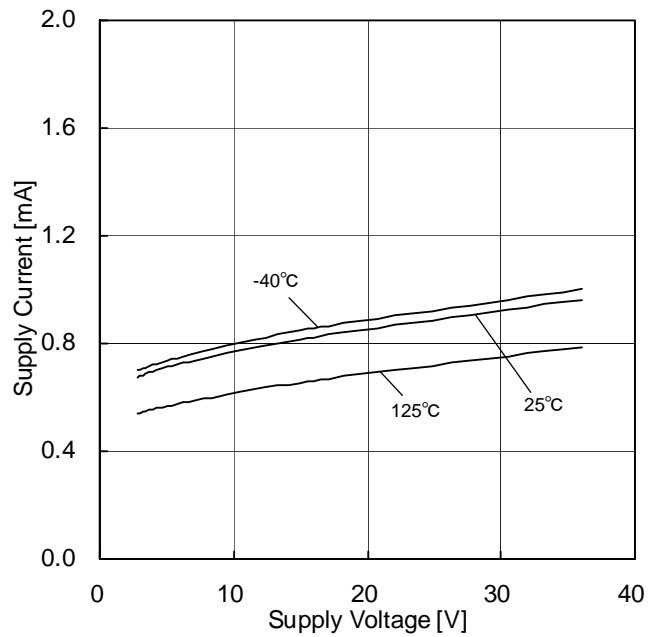
Figure 27. 回路電流－電源電圧特性
