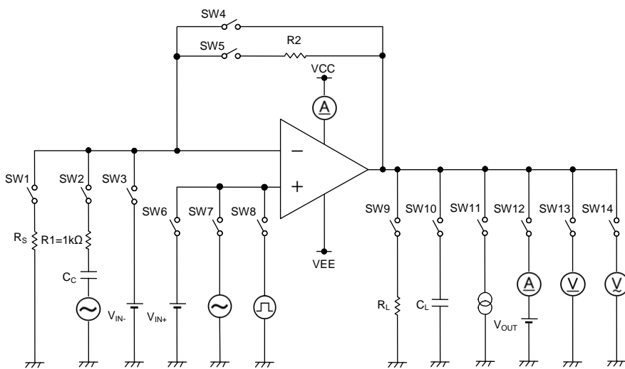
Figure 52. 測定回路 2 (片チャンネルのみ)
