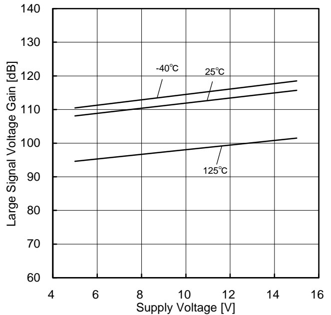
Figure 21. 大振幅電圧利得—電源電圧特性 (R L =2kΩ)
