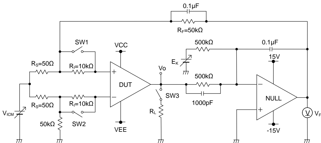
Figure 51. 測定回路 1 (1 チャンネルのみ)
