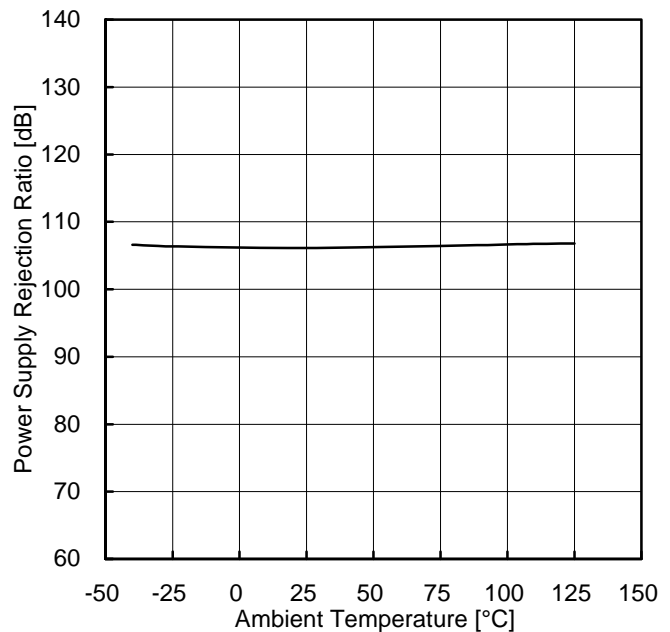
Figure 25 電源電圧除去比-温度特性
