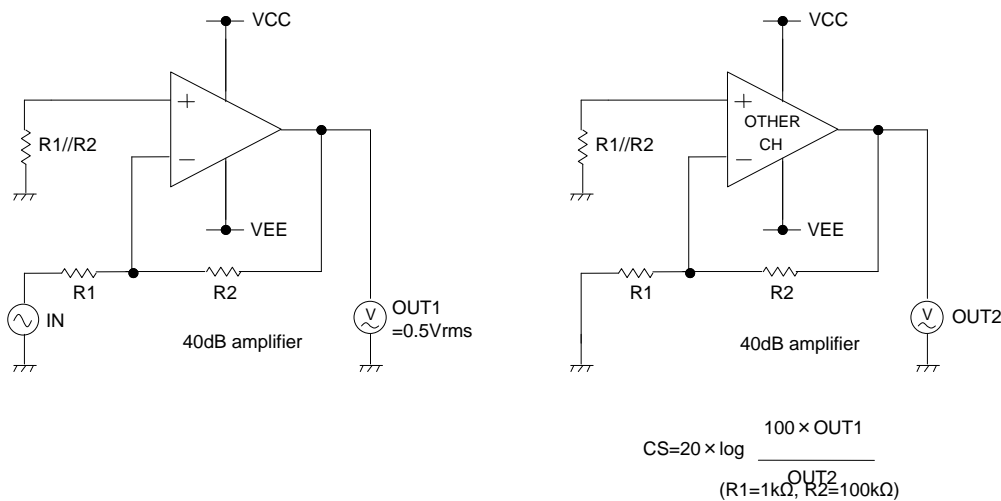
Figure 54. 測定回路 3 (チャンネルセパレーション)
