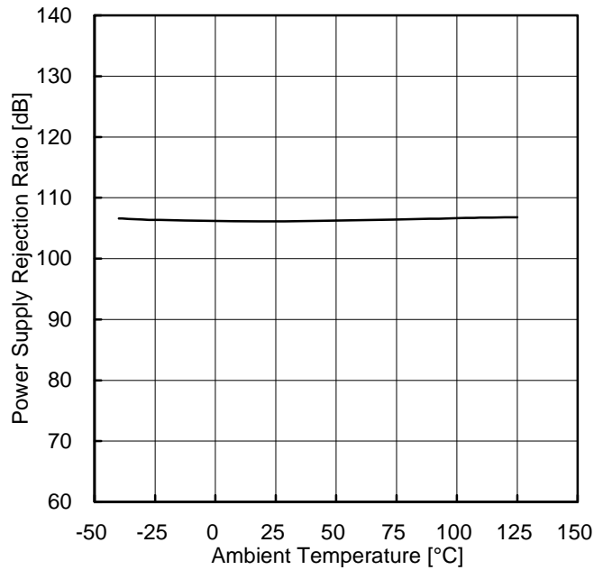
Figure 49. 電源電圧除去比-温度特性
