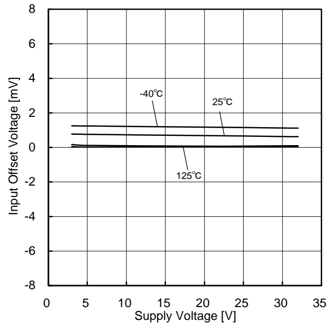
Figure 37. 入力オフセット電圧－電源電圧特性 (V ICM =0V, E K =-1.4V)
