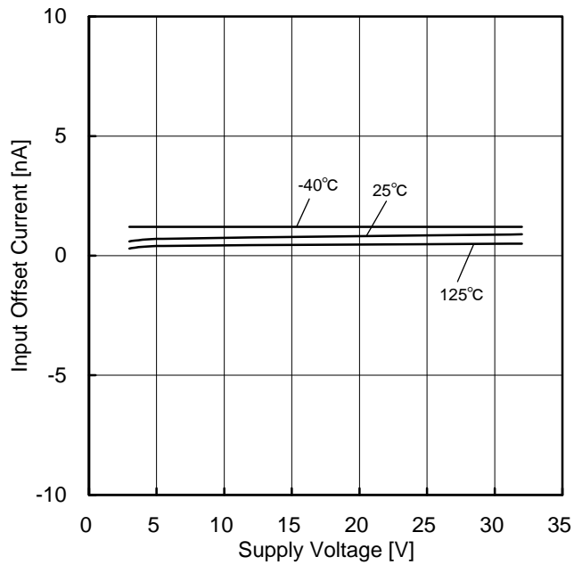
Figure 43. 入力オフセット電流—電源電圧特性 (VICM=0V, EK=-1.4V)
