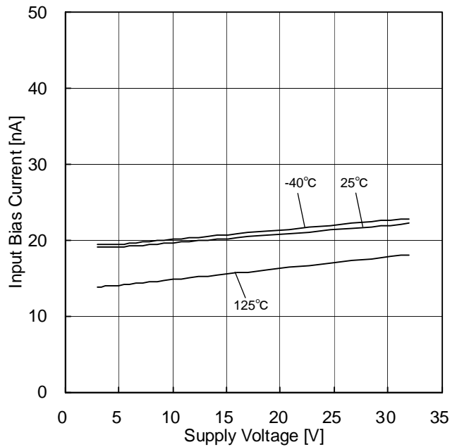
Figure 15. 入力バイアス電流-電源電圧特性 ( V_{ICM}=0V , E_K=-1.4V )
