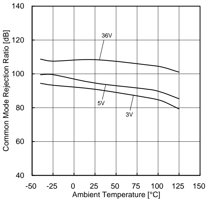
Figure 48. 同相信号除去比-温度特性
