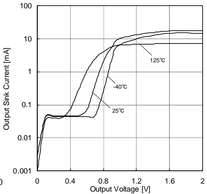
Figure 33. 出カシンク電流－出力電圧特性 (VCC=5V)
