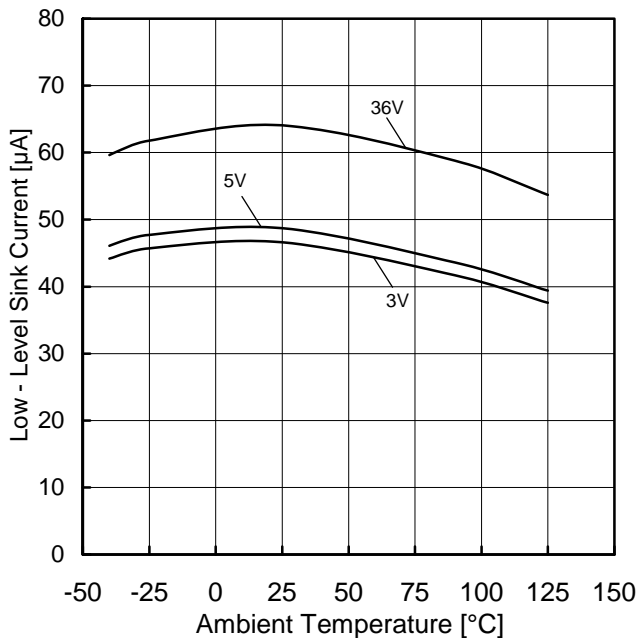
Figure 12. LOW レベルシンク電流－温度特性 (OUT=0.2V)
