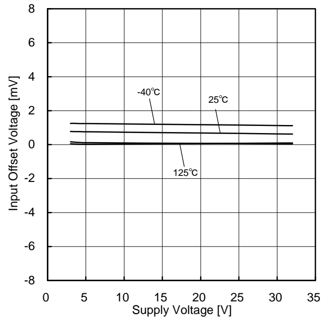
Figure 13. 入力オフセット電圧－電源電圧特性 (V ICM =0V, E K =-1.4V)
