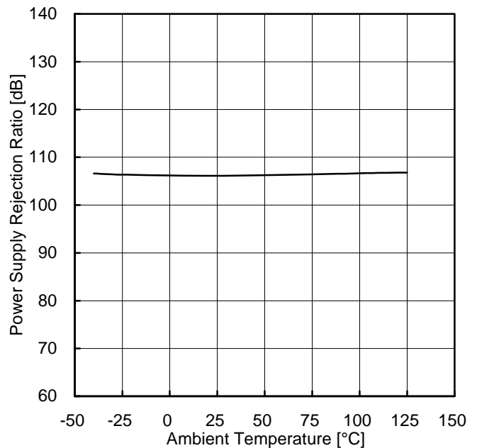
Figure 25 電源電圧除去比-温度特性
