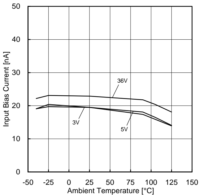
Figure 16. 入力バイアス電流-温度特性 ( V_{ICM}=0V , E_K=-1.4V )
