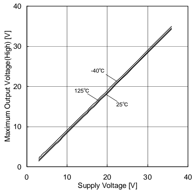
Figure 29. 最大出力電圧(High)－電源電圧特性 ( R_L=10k\Omega )
