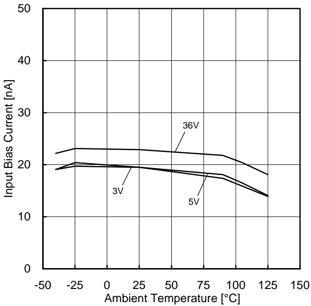
Figure 40. 入力バイアス電流－温度特性 ( V_{ICM}=0V , E_K=-1.4V )
