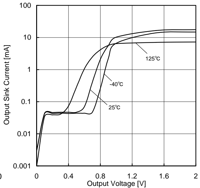
Figure 9. 出カシンク電流－出力電圧特性 (VCC=5V)
