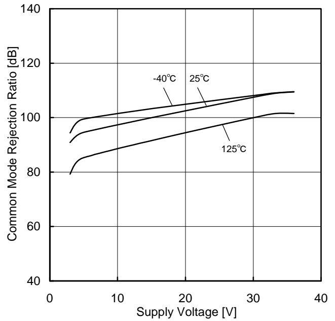
Figure 23. 同相信号除去比-電源電圧特性
