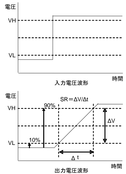
Figure 53. スルーレート測定時 入出力波形
