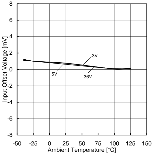
Figure 38. 入力オフセット電圧－温度特性 ( V_{ICM}=0V , E_K=-1.4V )
