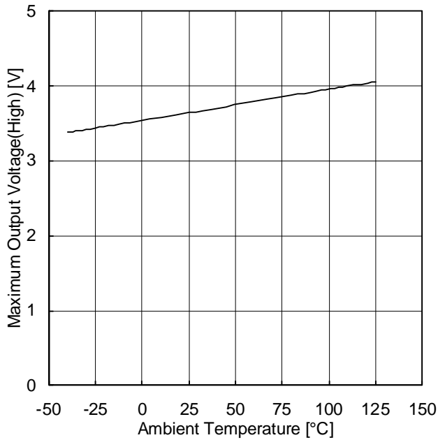
Figure 6. 最大出力電圧(High)－温度特性 (VCC=5V, R L =2kΩ)
