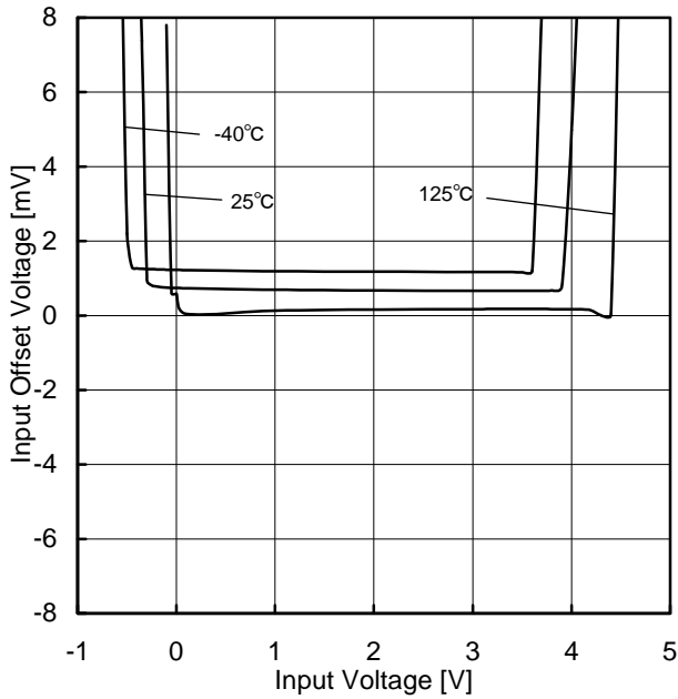
Figure 42. 入力オフセット電圧—同相入力電圧特性 (VCC=5V)
