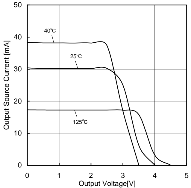
Figure 31. 出カソース電流－出力電圧特性 (VCC=5V)
