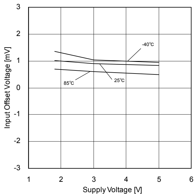
Figure 12. 入力オフセット電圧 - 電源電圧特性
