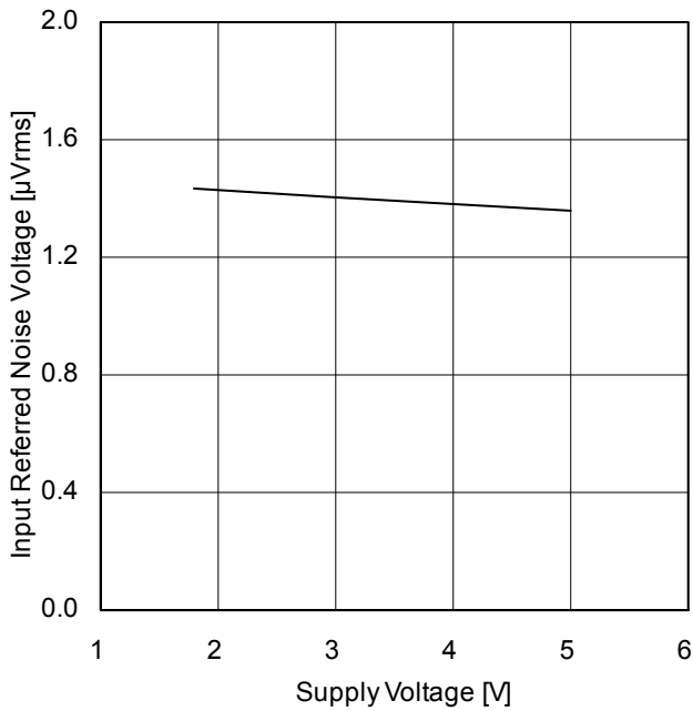
Figure 51. 入力換算雑音電圧 - 電源電圧特性 ( T_A=25^\circ\text{C} )
