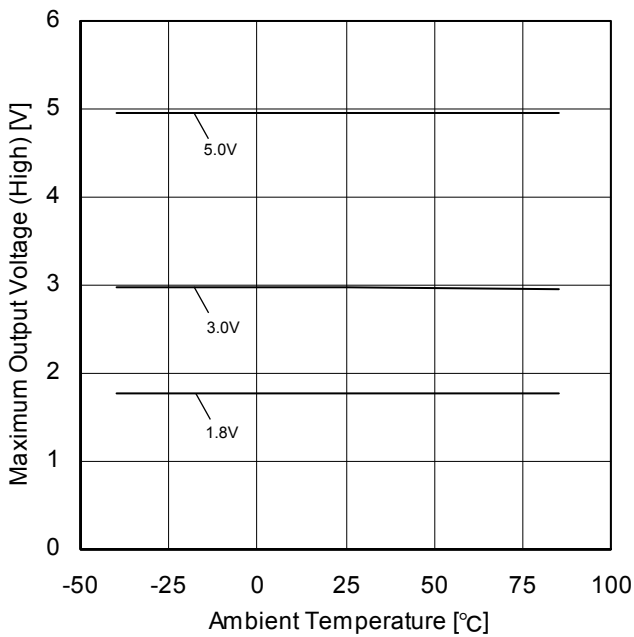
Figure 9. 最大出力電圧(High) - 温度特性 ( R_L=2k\Omega )
