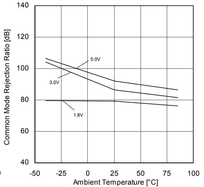
Figure 71. 同相信号除去比 - 温度特性
