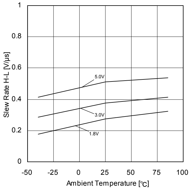
Figure 75. スルーレート(H-L) - 温度特性 ( R_L=2k\Omega )
