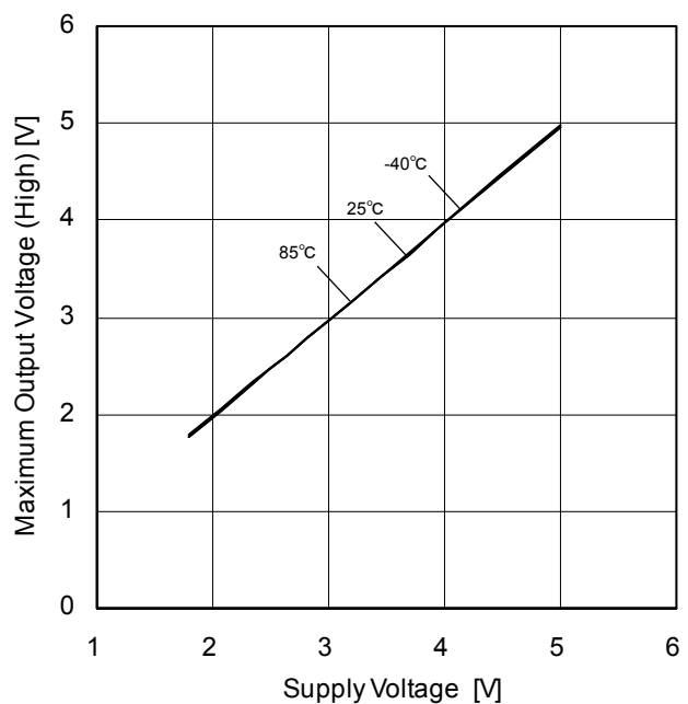
Figure 34. 最大出力電圧(High) - 電源電圧特性 ( R_L=2k\Omega )
