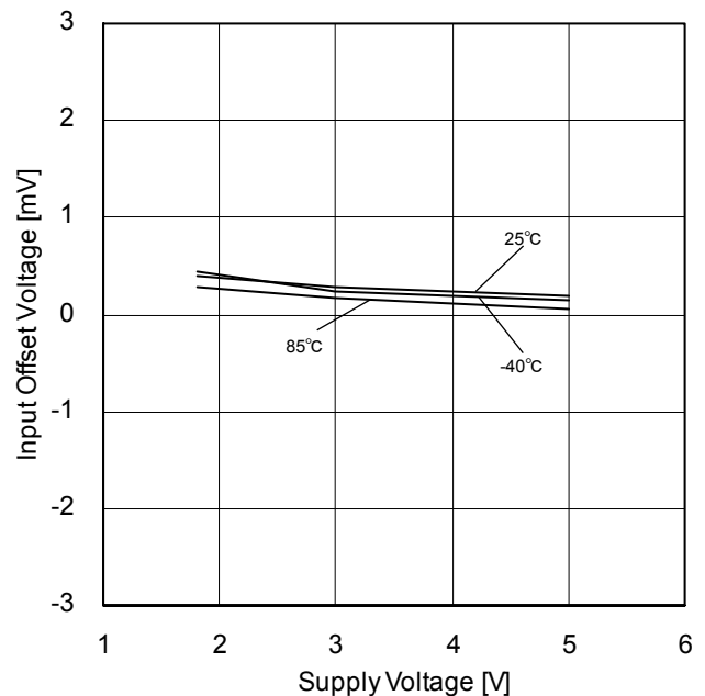
Figure 65. 入力オフセット電圧 - 電源電圧特性
