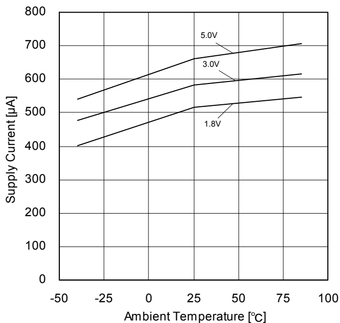
Figure 29. 回路電流 - 温度特性
