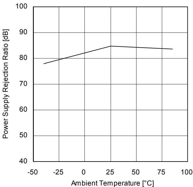
Figure 19. 電源電圧除去比 - 温度特性 ( V_+=1.8V \sim 5.0V )
