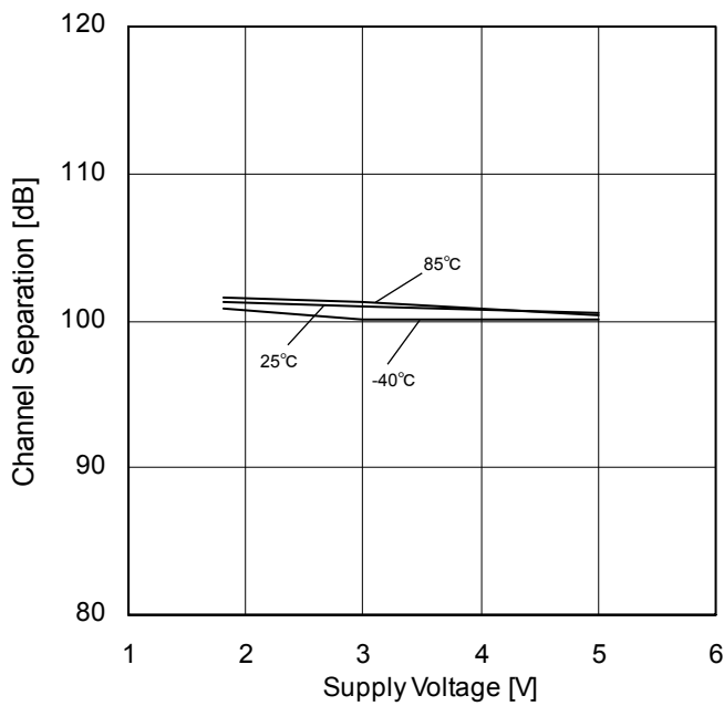
Figure 80. チャンネルセパレーション - 電源電圧特性
