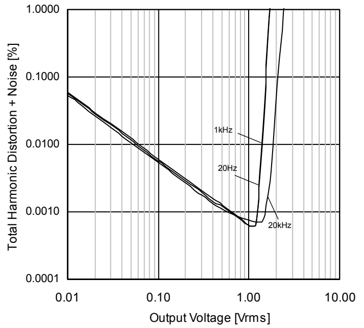
Figure 79. 全高調波歪率+雑音 - 出力電圧特性 ( V_+ = 5\text{V} , R_L = 2\text{k}\Omega , T_A = 25^\circ\text{C} )
