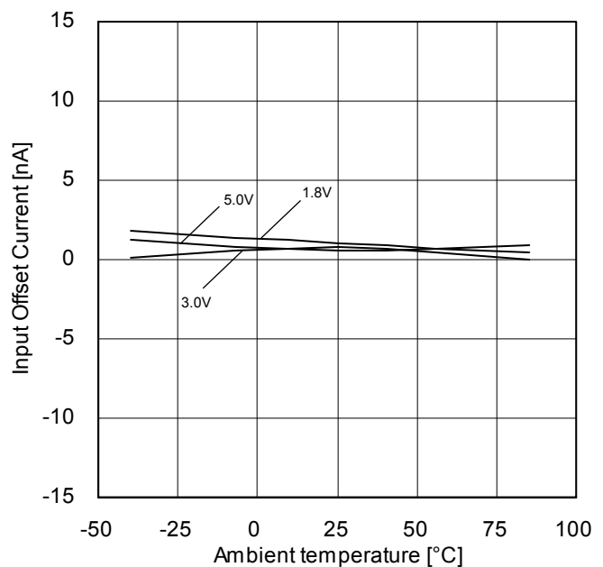
Figure 69. 入力オフセット電圧 - 温度特性
