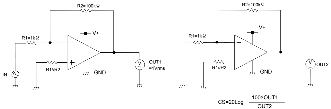
Figure 84. 測定回路 3 (チャンネルセパレーション)
