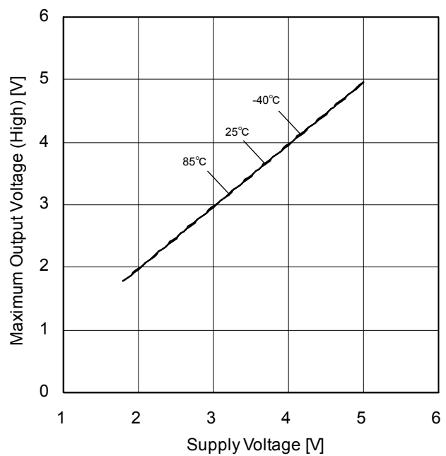
Figure 8. 最大出力電圧(High) - 電源電圧特性 ( R_L=2k\Omega )
