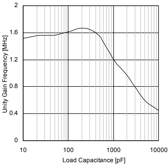
Figure 49. 単一利得周波数 - 負荷容量 ( V_+=5V, T_A=25^\circ C )
