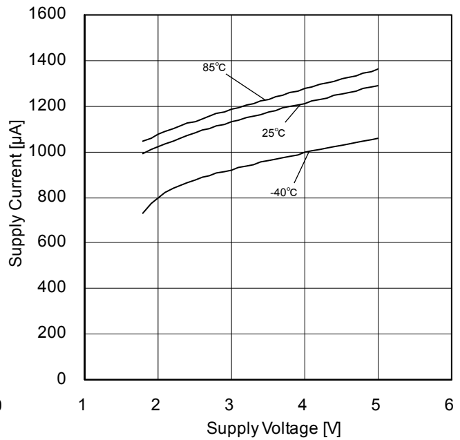
Figure 55. 回路電流 - 電源電圧特性
