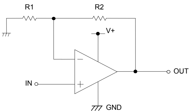
Figure 87. 非反転増幅回路
