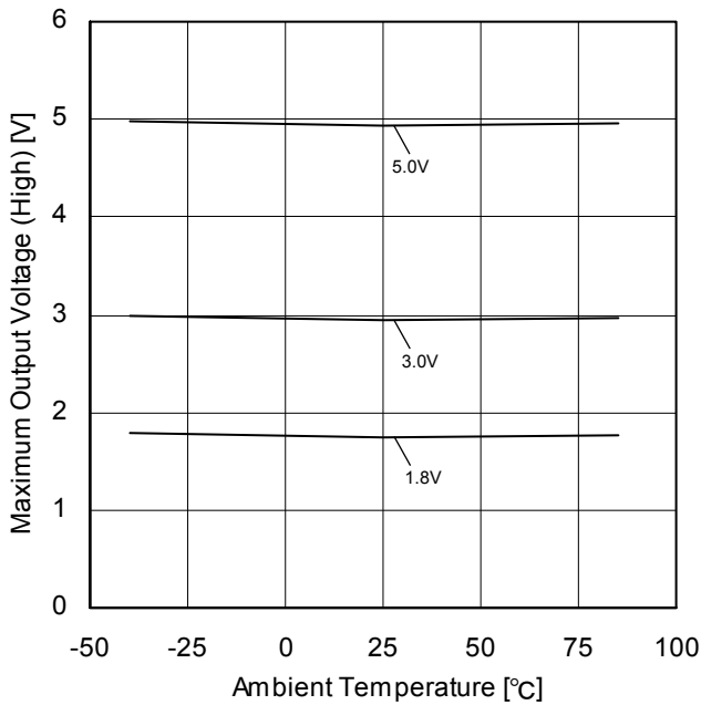
Figure 58. 最大出力電圧(High) - 温度特性 ( R_L=20k\Omega )
