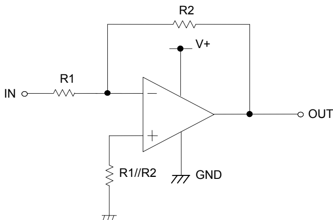
Figure 86. 反転増幅回路
