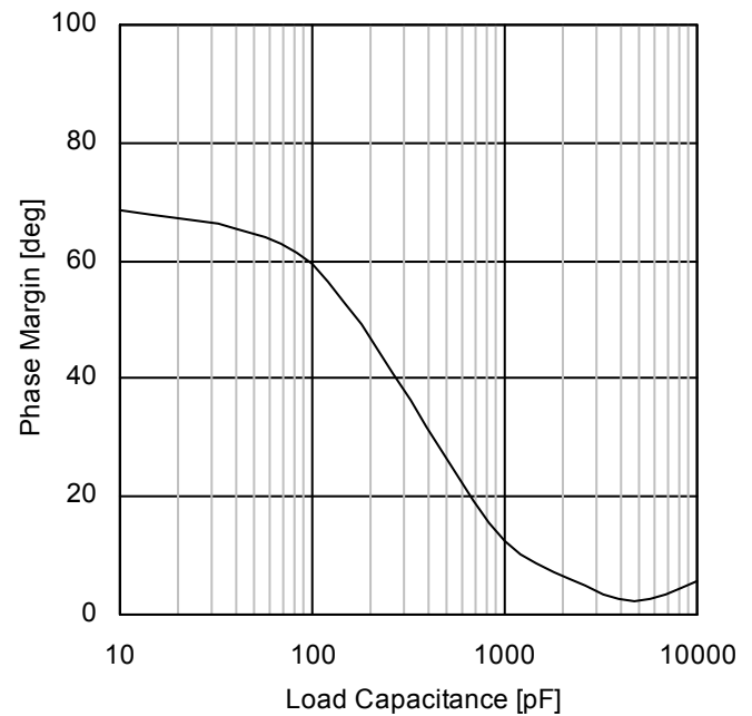
Figure 50. 位相余裕 - 負荷容量 ( V_+=5V, T_A=25^\circ C )
