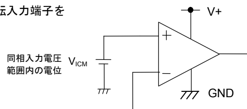
Figure 90. 未使用回路処理例
