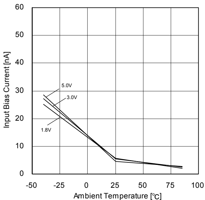
Figure 68. 入力バイアス電流 - 温度特性
