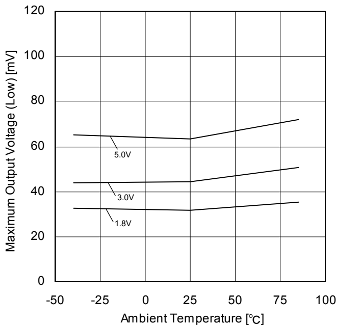
Figure 64. 最大出力電圧(Low) - 温度特性 ( R_L=2k\Omega )
