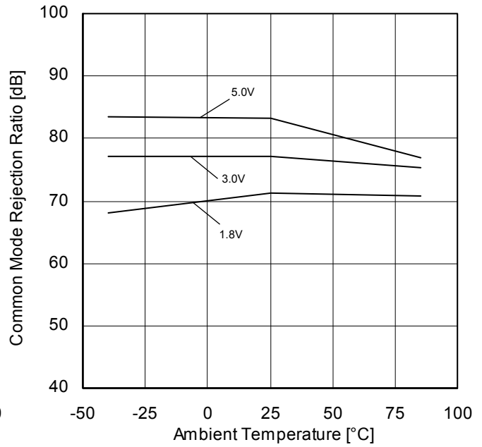
Figure 44. 同相信号除去比 - 温度特性
