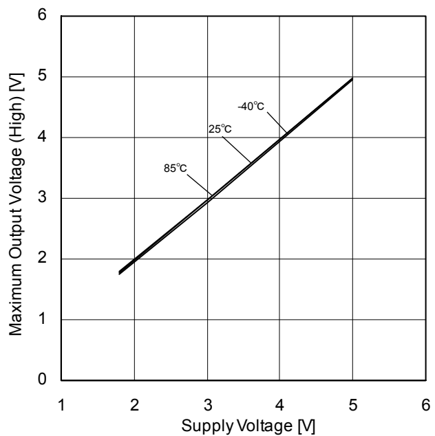
Figure 57. 最大出力電圧(High) - 電源電圧特性 ( R_L=20k\Omega )
