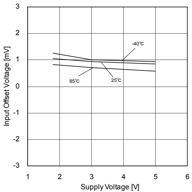
Figure 38. 入力オフセット電圧 - 電源電圧特性
