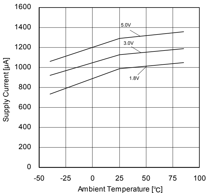
Figure 56. 回路電流 - 温度特性
