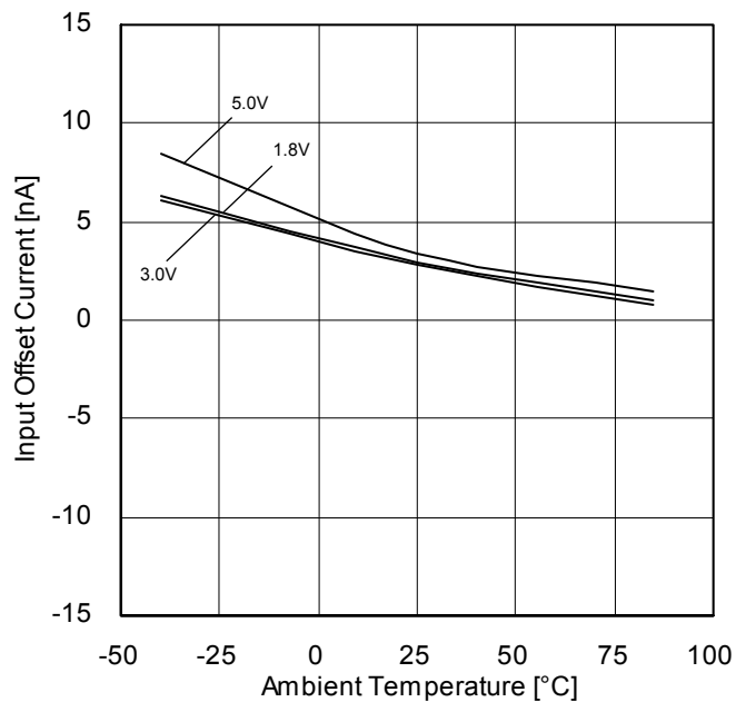
Figure 16. 入力オフセット電流 - 温度特性
