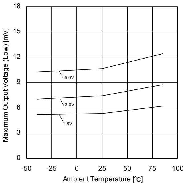
Figure 60. 最大出力電圧(Low) - 温度特性 ( R_L=20k\Omega )
