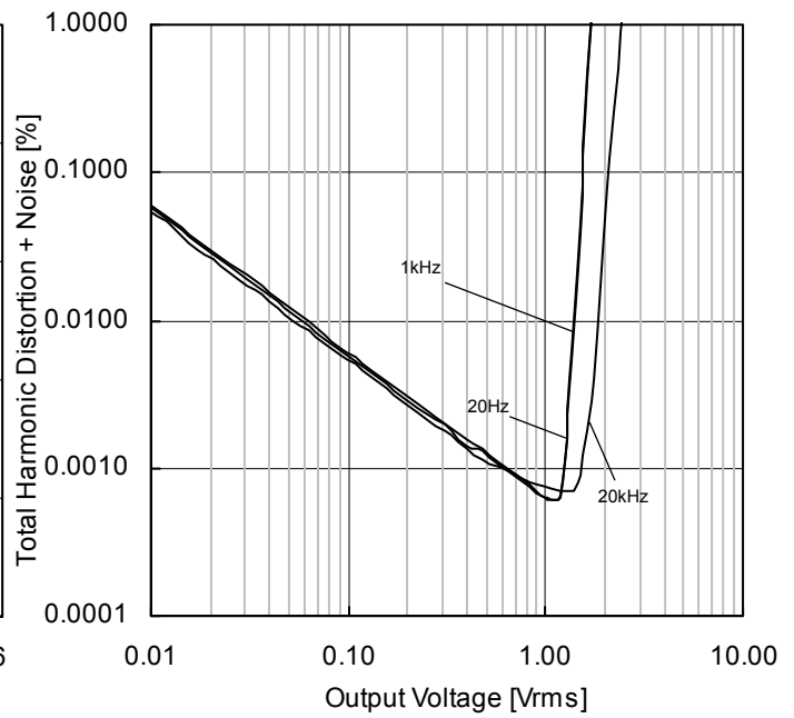
Figure 26. 全高調波歪率+雑音 - 出力電圧 ( V_+=5\text{V} , R_L=2\text{k}\Omega , T_A=25^\circ\text{C} )
