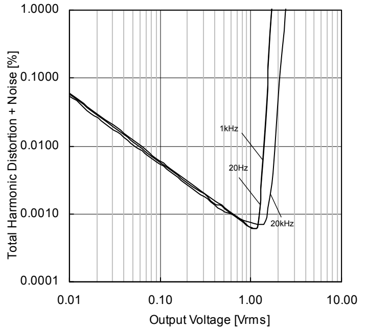
Figure 52. 全高調波歪率+雑音 - 出力電圧特性 ( V_+=5\text{V} , R_L=2\text{k}\Omega , T_A=25^\circ\text{C} )
