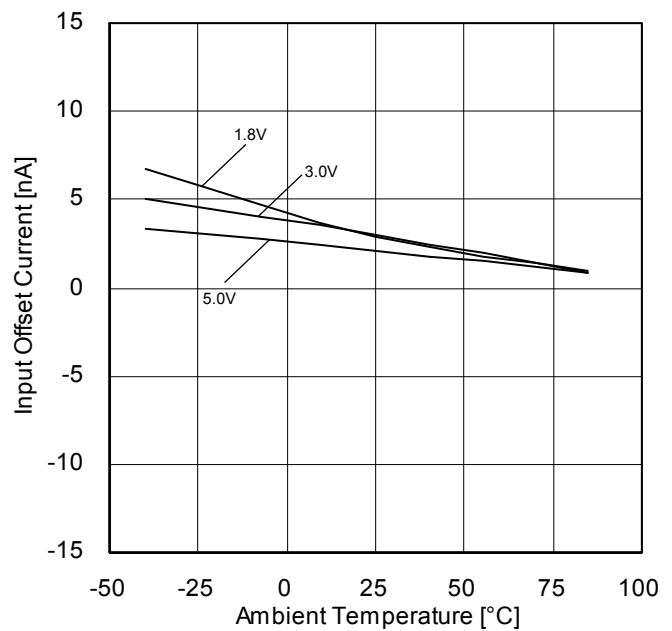
Figure 42. 入力オフセット電流 - 温度特性
