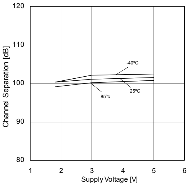
Figure 53. チャンネルセパレーション - 電源電圧特性
