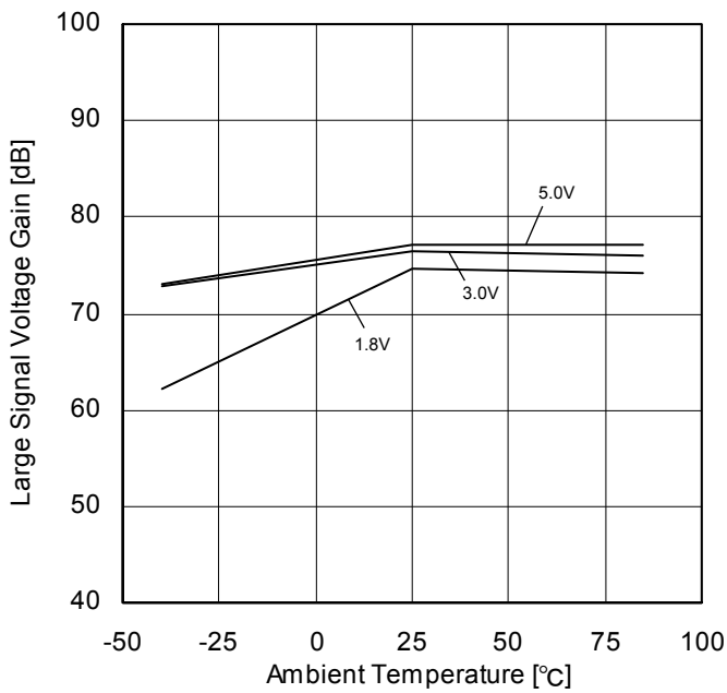
Figure 17. 大振幅電圧利得 - 温度特性 ( R_L=2k\Omega )
