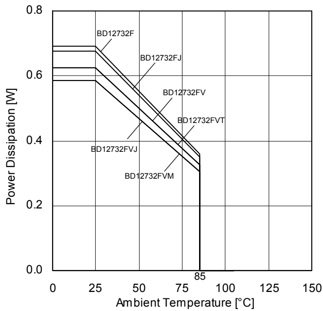
Figure 27. ディレーティングカーブ
