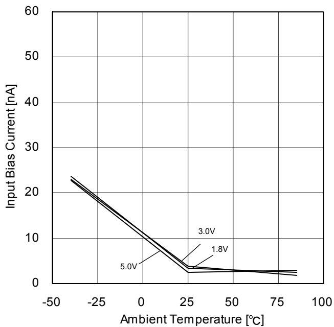
Figure 41. 入力バイアス電流 - 温度特性
