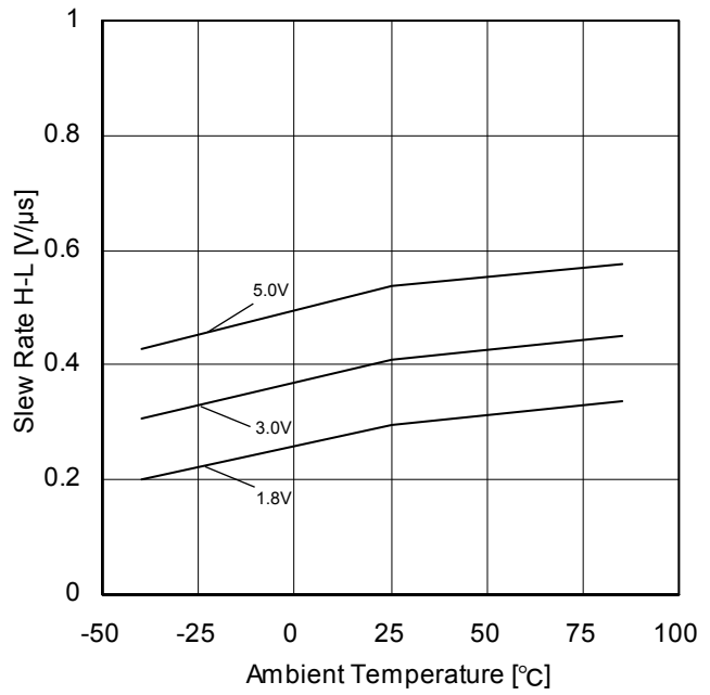
Figure 48. スルーレート(H-L) - 温度特性 ( R_L=2k\Omega )
