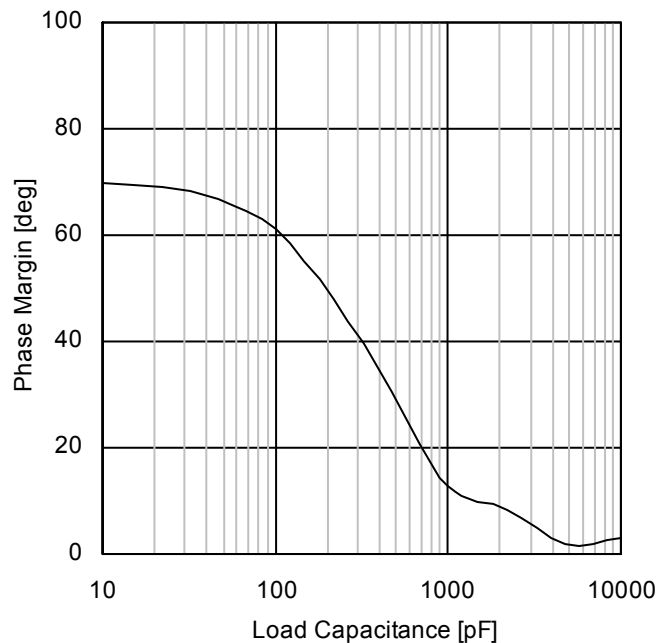
Figure 24. 位相余裕 - 負荷容量 ( V+=5V, T_A=25^\circ C )
