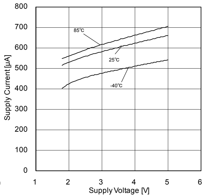
Figure 28. 回路電流 - 電源電圧特性
