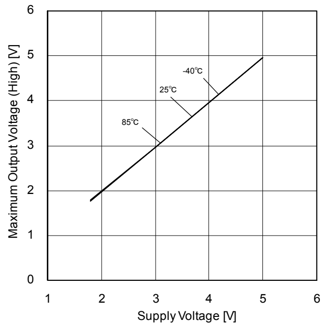
Figure 4. 最大出力電圧(High) - 電源電圧特性 ( R_L=20k\Omega )
