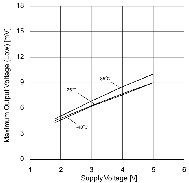
Figure 32. 最大出力電圧(Low) - 電源電圧特性 ( R_L=20k\Omega )
