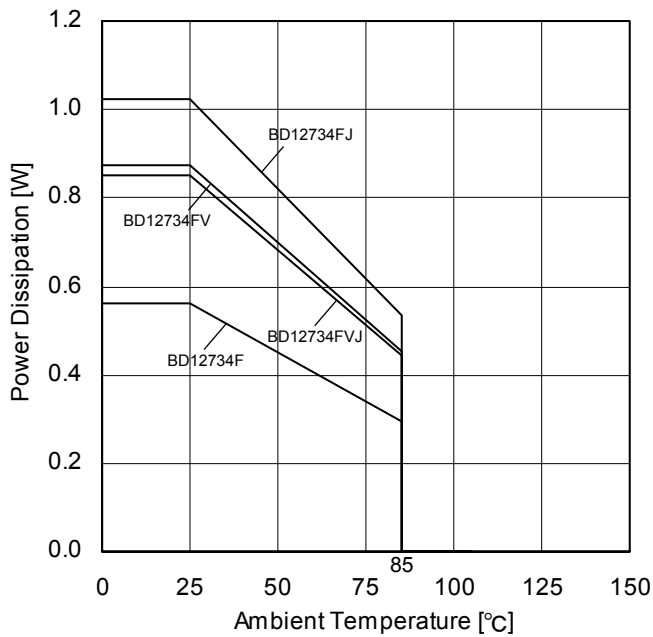
Figure 54. ディレーティングカーブ
