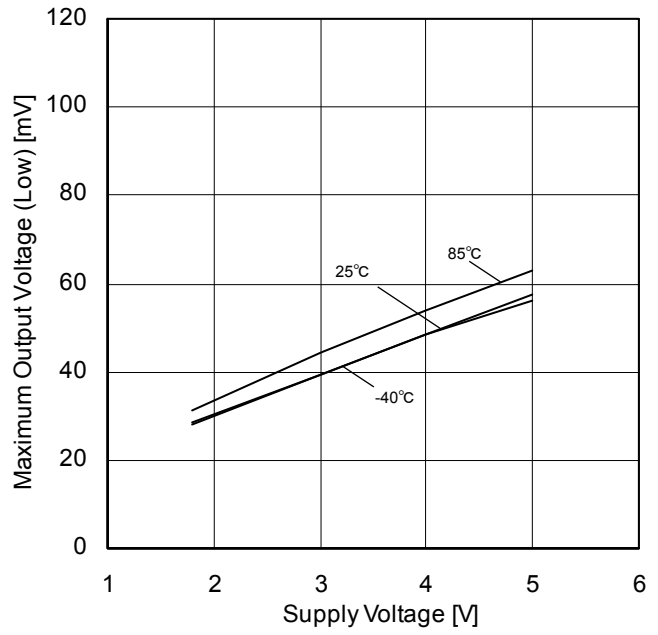
Figure 36. 最大出力電圧(Low) - 電源電圧特性 ( R_L=2k\Omega )
