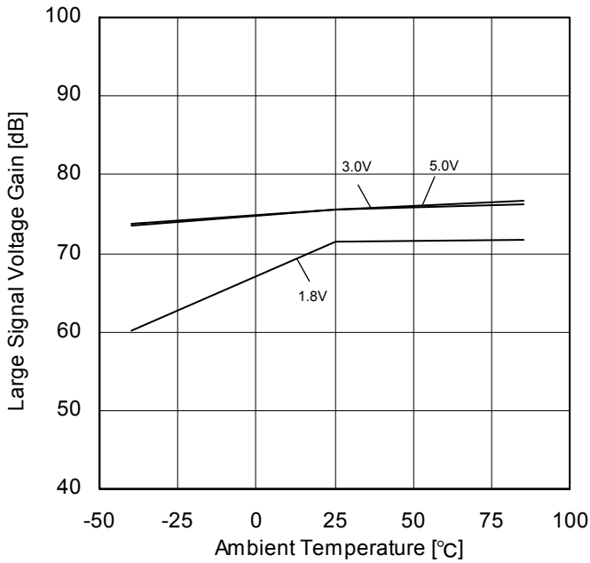
Figure 43. 大振幅電圧利得 - 温度特性 ( R_L=2k\Omega )
