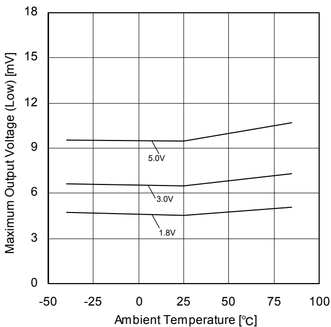
Figure 7. 最大出力電圧(Low) - 温度特性 ( R_L=20k\Omega )
