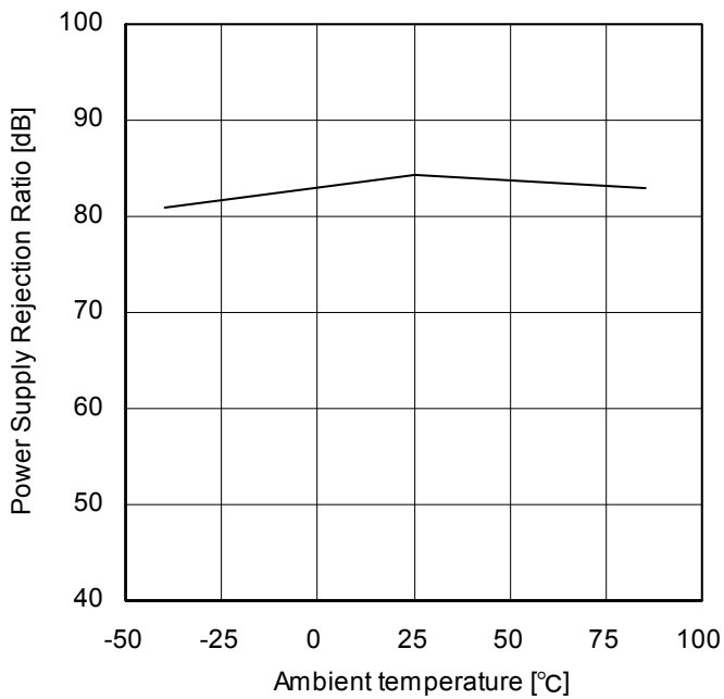
Figure 72. 電源電圧除去比 - 温度特性 ( V+=1.8V \sim 5.0V )
