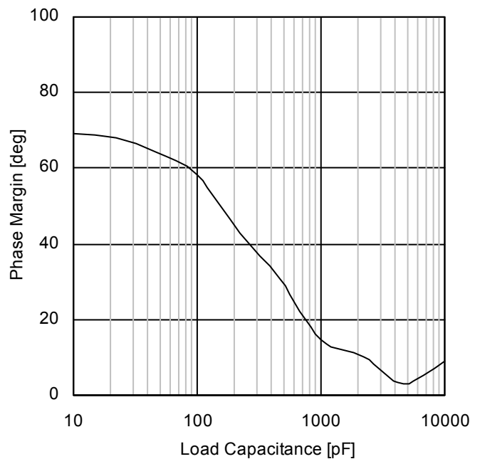
Figure 77. 位相余裕 - 負荷容量 ( V+=5V, T_A=25^\circ C )
