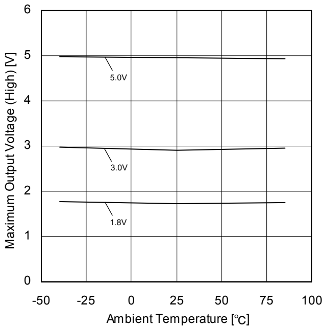
Figure 62. 最大出力電圧(High) - 温度特性 ( R_L=2k\Omega )
