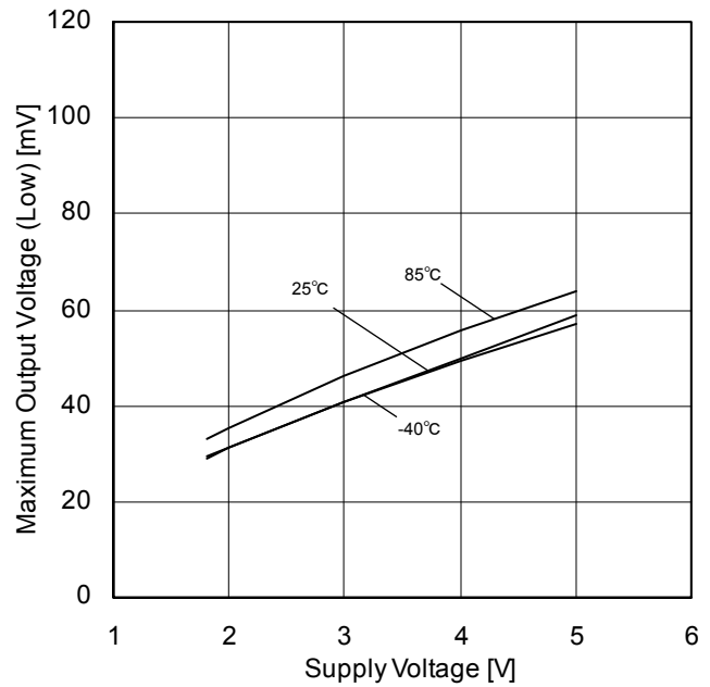
Figure 10. 最大出力電圧(Low) - 電源電圧特性 ( R_L=2k\Omega )
