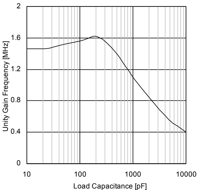
Figure 76. 単一利得周波数 - 負荷容量 ( V+=5V, T_A=25^\circ C )
