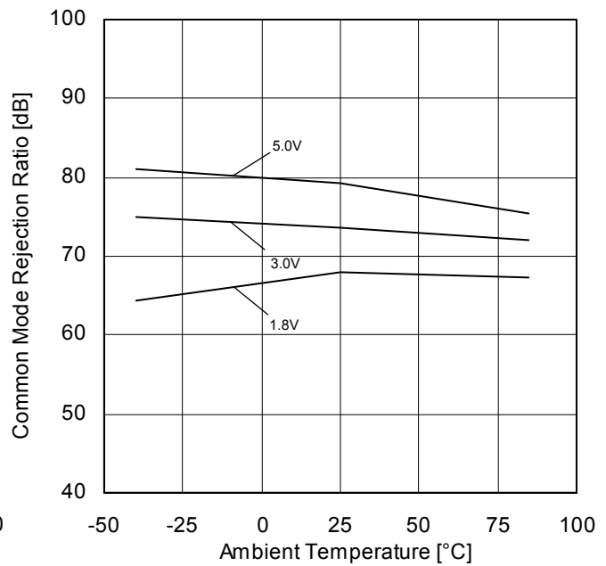
Figure 18. 同相信号除去比 - 温度特性
