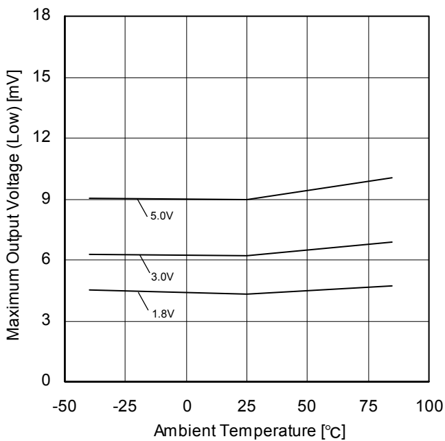
Figure 33. 最大出力電圧(Low) - 温度特性 ( R_L=20k\Omega )
