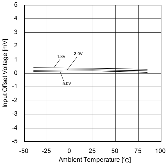
Figure 66. 入力オフセット電圧 - 温度特性
