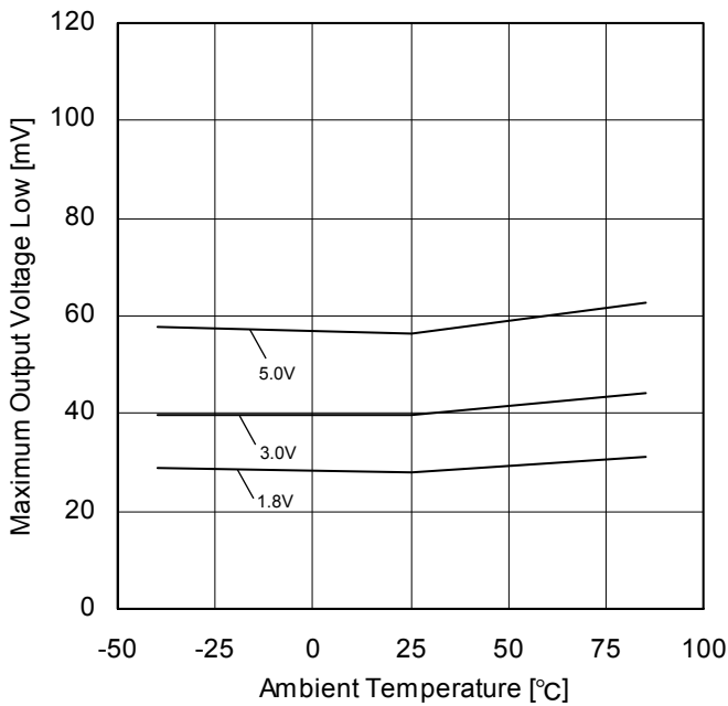
Figure 37. 最大出力電圧(Low) - 温度特性 ( R_L=2k\Omega )
