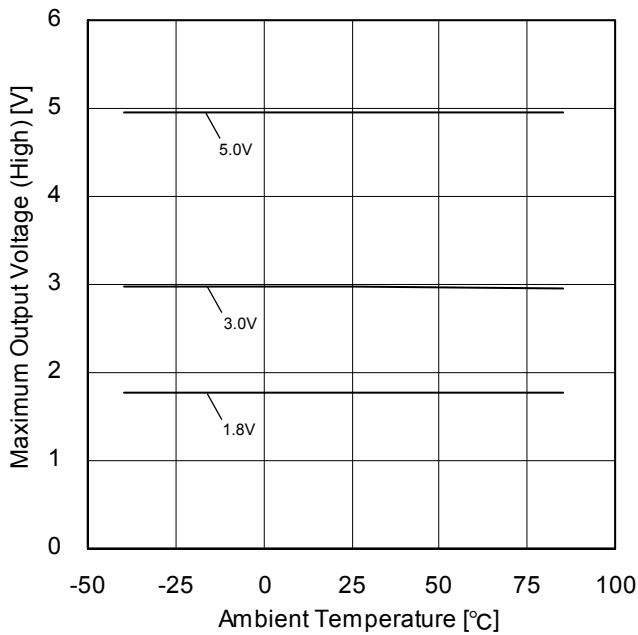
Figure 5. 最大出力電圧(High) - 温度特性 ( R_L=20k\Omega )
