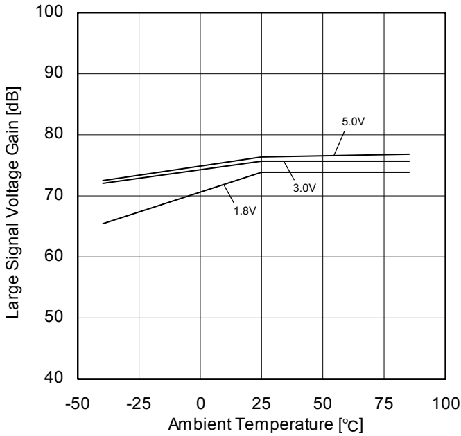
Figure 70. 大振幅電圧利得 - 温度特性 ( R_L=2k\Omega )
