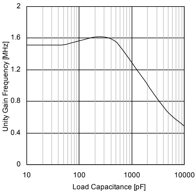
Figure 23. 単一利得周波数 - 負荷容量 ( V+=5V, T_A=25^\circ C )
