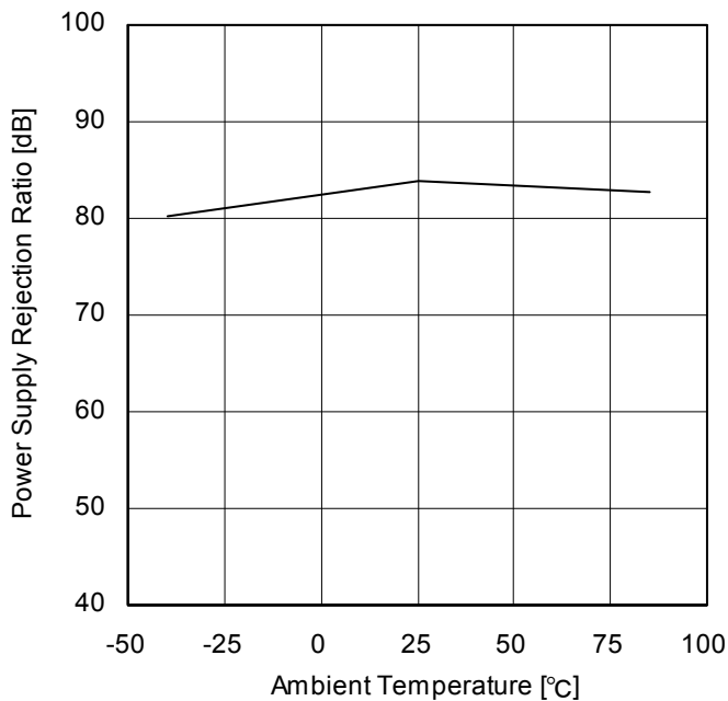
Figure 45. 電源電圧除去比 - 温度特性 ( V_+=1.8V \sim 5.0V )
