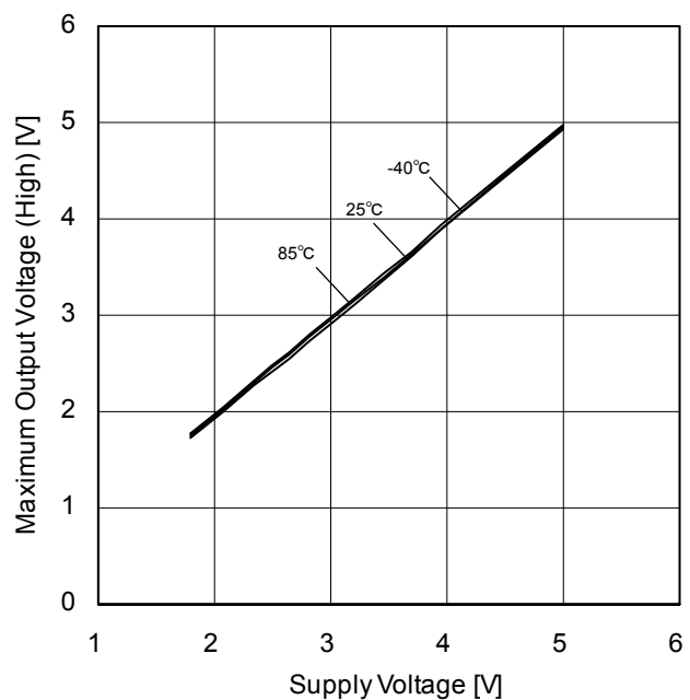
Figure 61. 最大出力電圧(High) - 電源電圧特性 ( R_L=2k\Omega )
