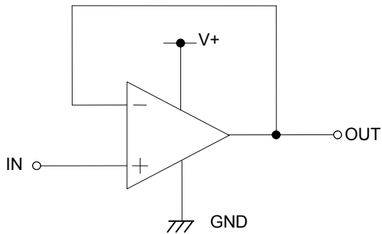
Figure 85. ボルテージフォロア回路
