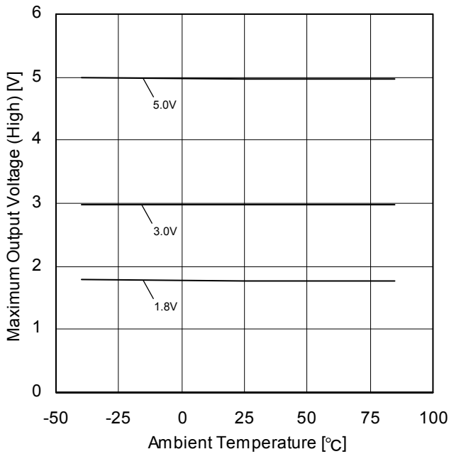
Figure 31. 最大出力電圧(High) - 温度特性 ( R_L=20k\Omega )
