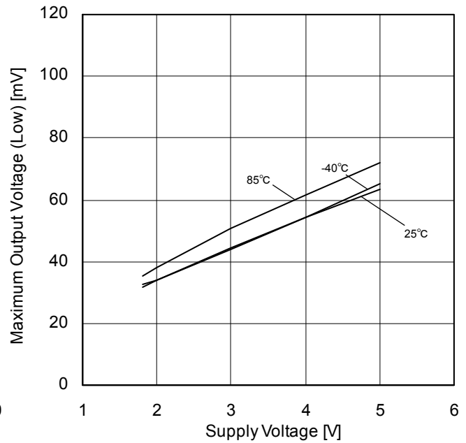
Figure 63. 最大出力電圧(Low) - 電源電圧特性 ( R_L=2k\Omega )
