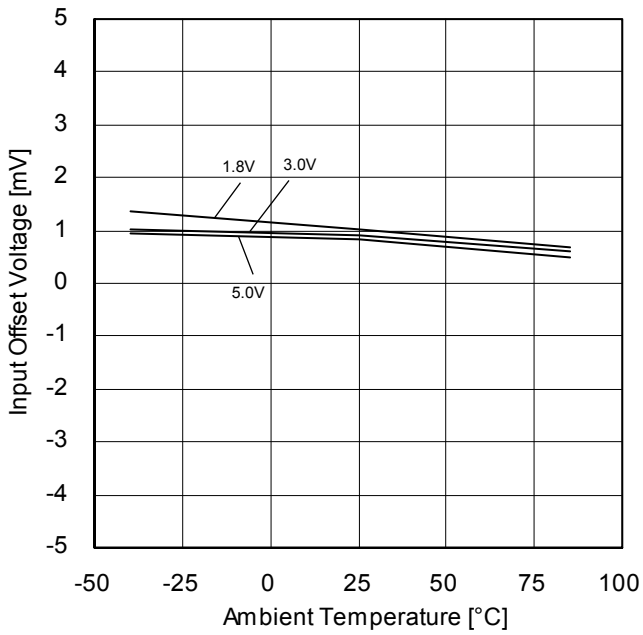
Figure 13. 入力オフセット電圧 - 温度特性
