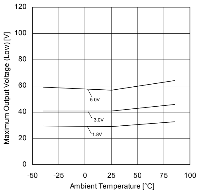
Figure 11. 最大出力電圧(Low) - 温度特性 ( R_L=2k\Omega )
