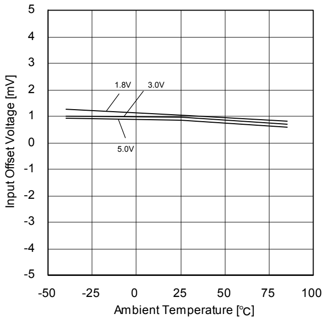
Figure 39. 入力オフセット電圧 - 温度特性
