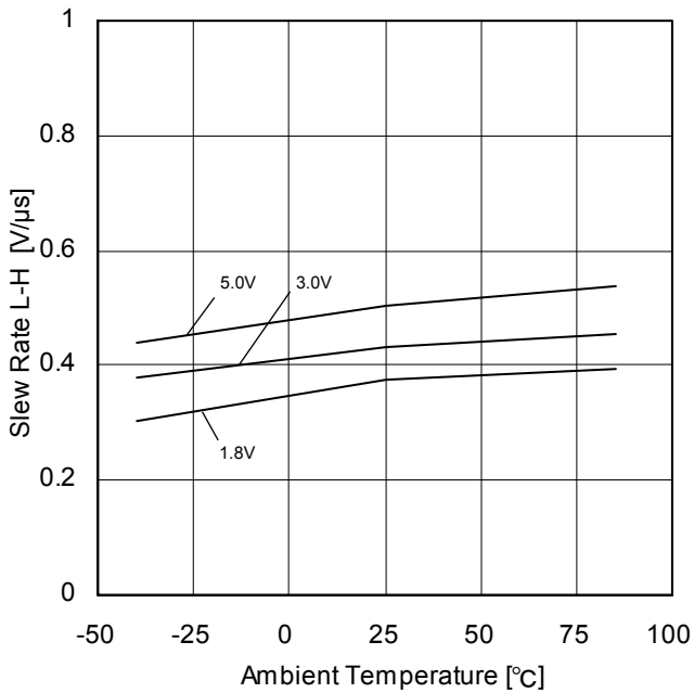
Figure 21. スルーレート(L-H) - 温度特性 ( R_L=2k\Omega )
