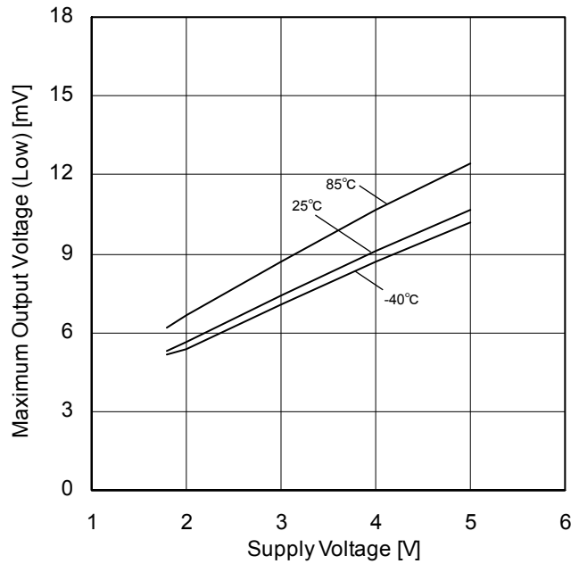
Figure 59. 最大出力電圧(Low) - 電源電圧特性 ( R_L=20k\Omega )
