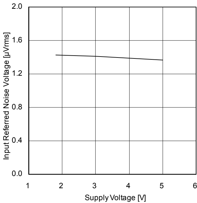
Figure 25. 入力換算雑音電圧 - 電源電圧特性 ( T_A=25^\circ\text{C} )
