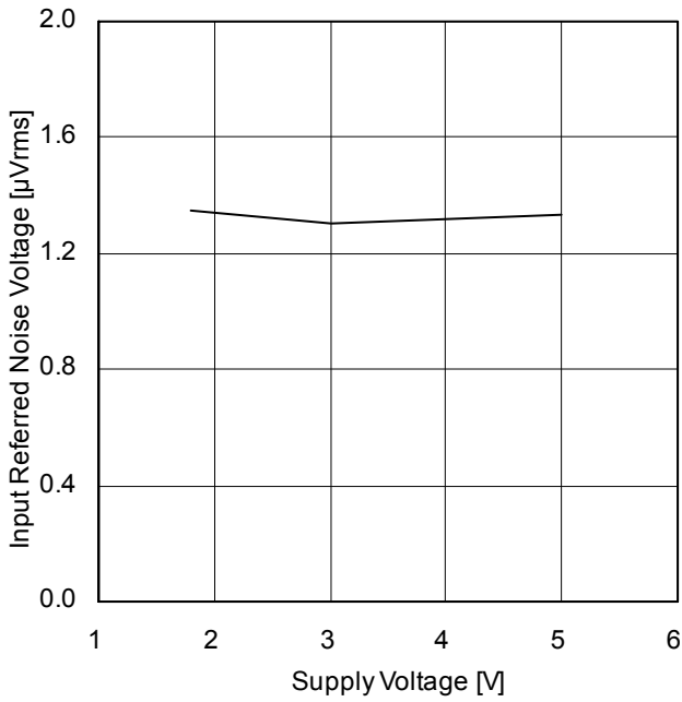
Figure 78. 入力換算雑音電圧 - 電源電圧特性 ( T_A = 25^\circ\text{C} )
