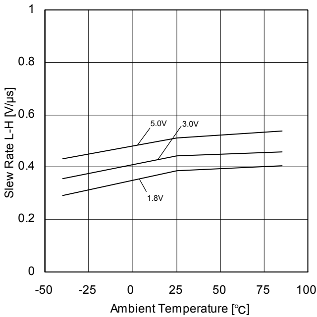
Figure 47. スルーレート(L-H) - 温度特性 ( R_L=2k\Omega )
