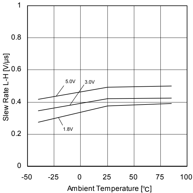
Figure 74. スルーレート(L-H) - 温度特性 ( R_L=2k\Omega )
