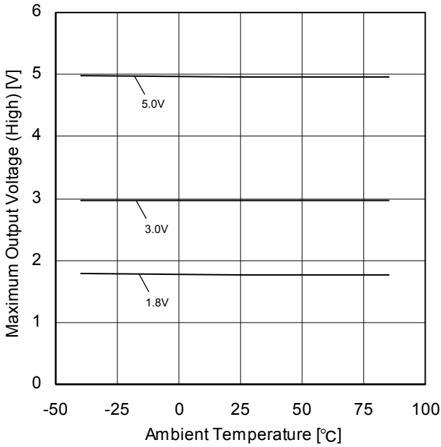
Figure 35. 最大出力電圧(High) - 温度特性 ( R_L=2k\Omega )
