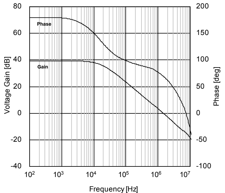
Figure 46. 電圧利得・位相 - 周波数特性 ( V_+=5V, R_L=2k\Omega, T_A=25^\circ C )
