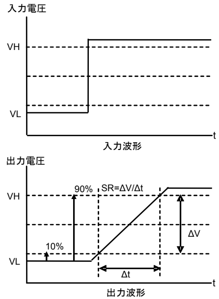
Figure 83. スルーレート測定時 入出力波形
