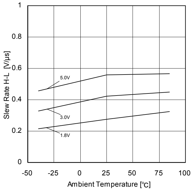
Figure 22. スルーレート(H-L) - 温度特性 ( R_L=2k\Omega )
