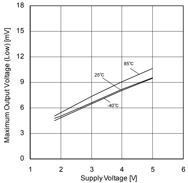
Figure 6. 最大出力電圧(Low) - 電源電圧特性 ( R_L=20k\Omega )
