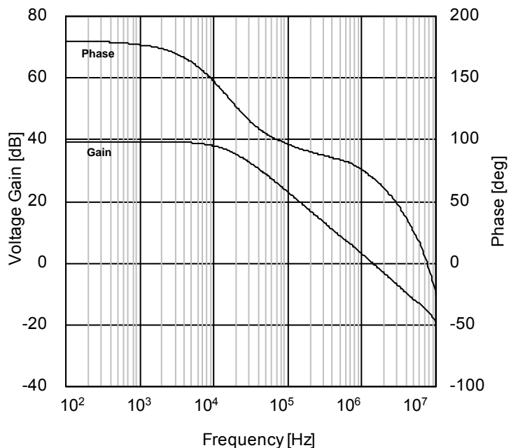
Figure 20. 電圧利得・位相 - 周波数特性 ( V_+=5V, R_L=2k\Omega, T_A=25^\circ C )
