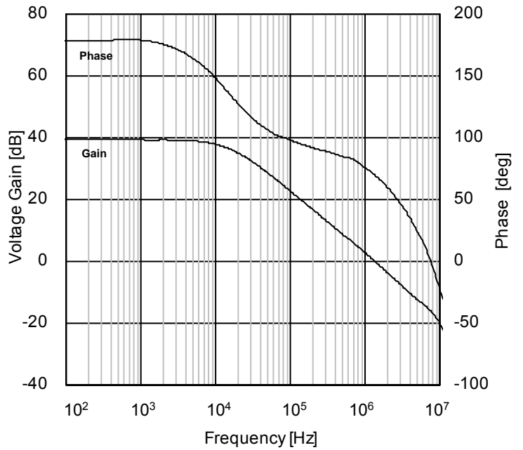
Figure 73. 電圧利得・位相 - 周波数特性 ( V+=5V, R_L=2k\Omega, T_A=25^\circ C )
