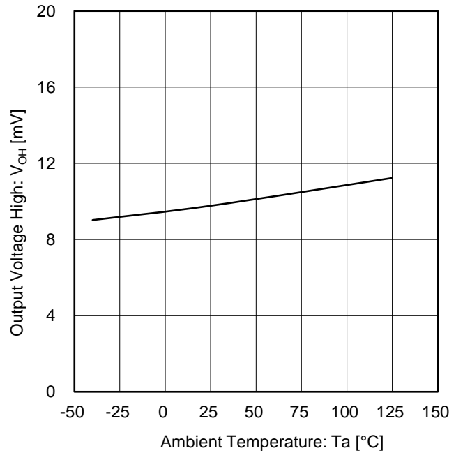
Figure 4. 出力電圧 High vs 温度 ( V_S = 5\text{ V}, R_L = 10\text{ k}\Omega )
