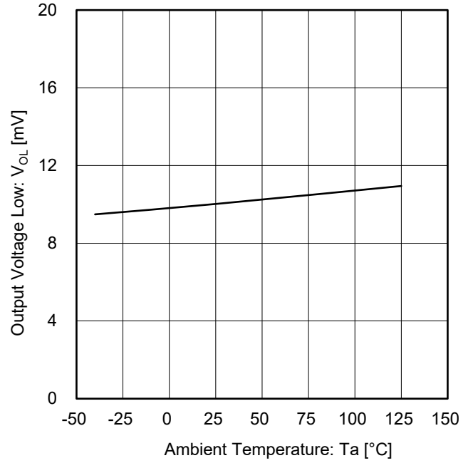
Figure 6. 出力電圧 Low vs 温度 ( V_S = 5\text{ V} , R_L = 10\text{ k}\Omega )
