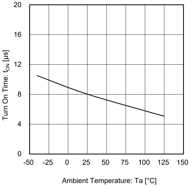
Figure 25. ターンオン時間 vs 温度 ( V_S = 5\text{ V} )
