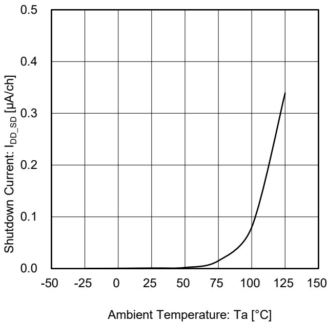
Figure 27. シャットダウン時回路電流 vs 温度 ( V_S = 5\text{ V} )
