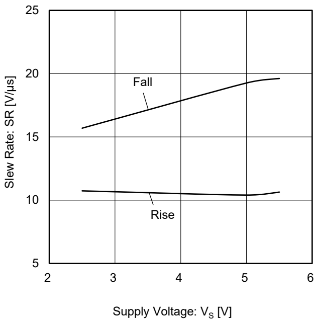
Figure 19. スルーレート vs 電源電圧
