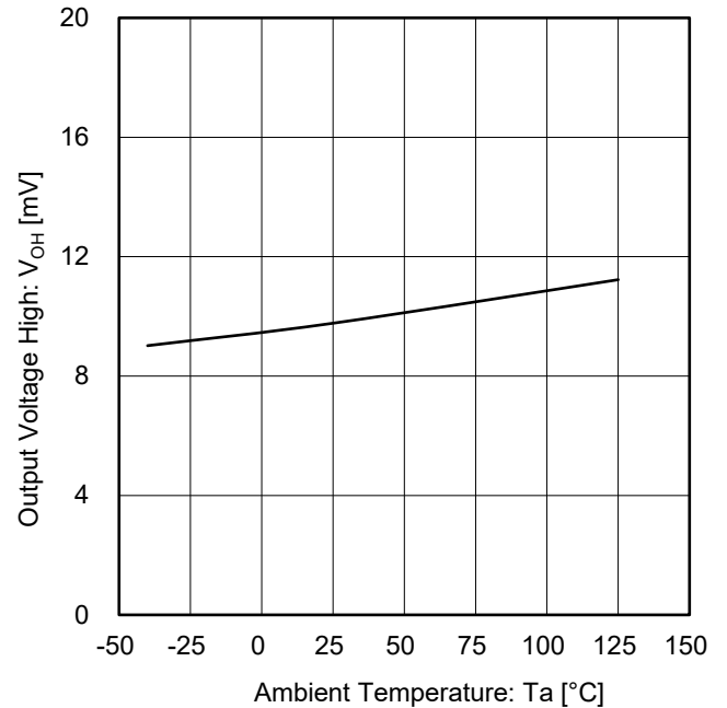
Figure 4. 出力電圧 High vs 温度 ( V_S = 5\text{ V} , R_L = 10\text{ k}\Omega )
