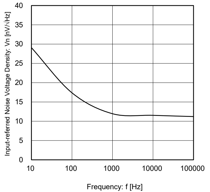
Figure 18. 入力換算雑音電圧密度 vs 周波数 ( V_S = 5\text{ V} )
