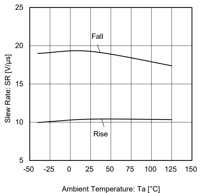
Figure 20. スルーレート vs 温度 ( V_S = 5\text{ V} )
