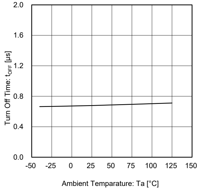
Figure 26. ターンオフ時間 vs 温度 ( V_S = 5\text{ V} )
